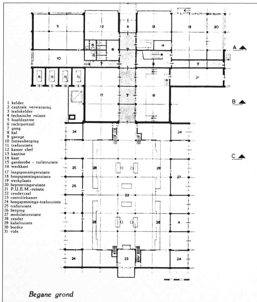
6. Plattegrond van de bega- ne grond van het zenderge- bouw.
