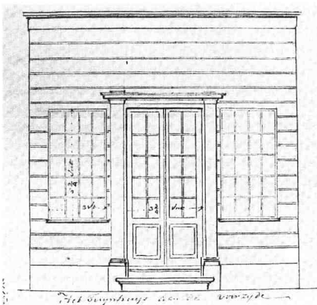
afb. 8 Eén van de bouwtekeningen van het speelhuisje. Familiefarchief Van Stolk band IX nr. 28.
