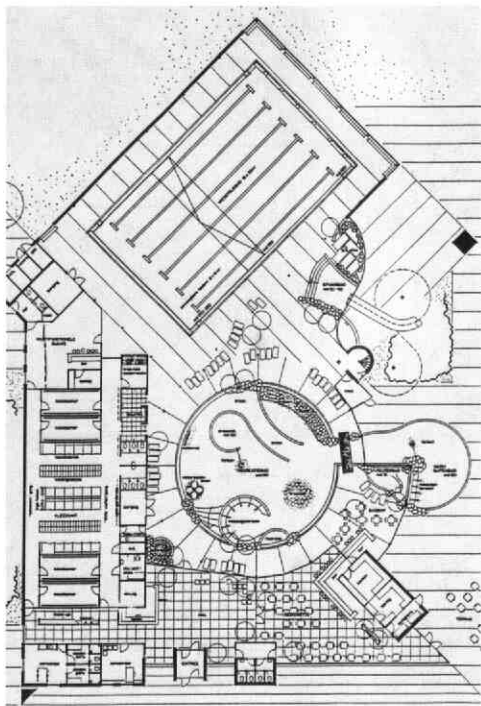
afb. 14 Plattegrond van het nieuwe zwembad. Duidelijk zicht- baar is het 25 m wedstrijd/instruc- tiebad en in het midden het recre- atieve gedeelte. Het buitenbad is helaas verdwe- nen.
