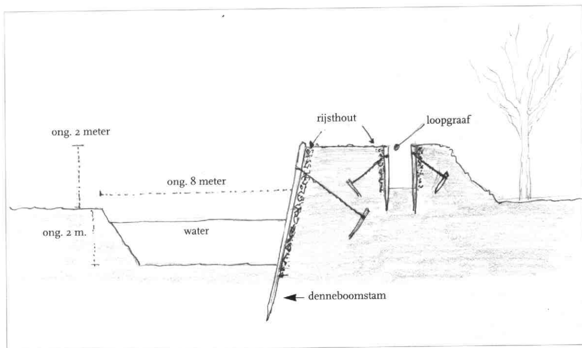
afb. 12 Doorsnee- tekening van een tank- gracht zoals deze aan de westzijde van IJsselstein is aangelegd. (zie platte- grond op pag 271).
