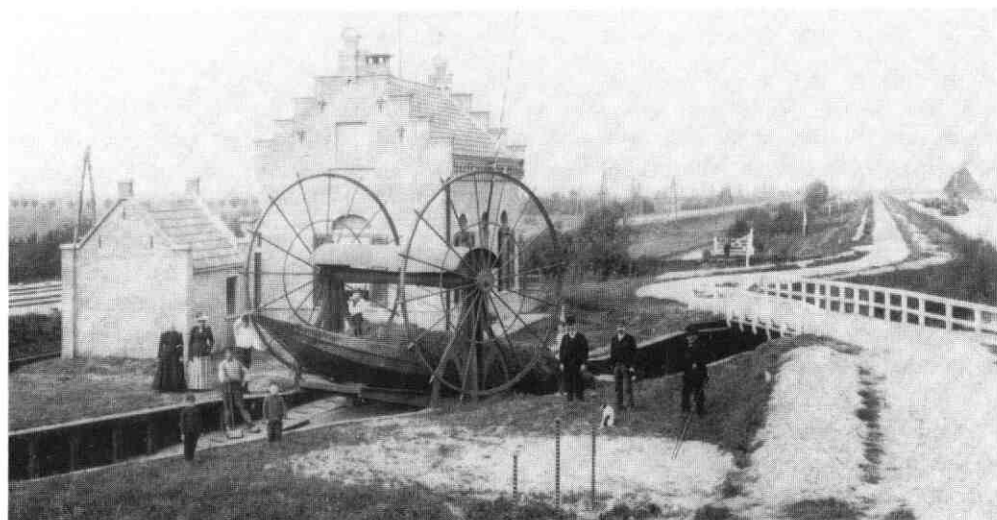
afb. 2 Werking van de overtoom in de Haarrijn bij Maarssen. Deze over- toom werd in 1891 in gebruik geno- men.
