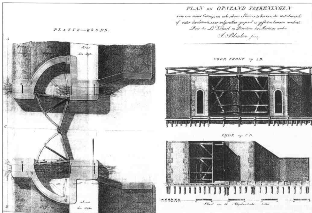
afb. 8 Tekening van een waaierdeur door Jan Blanken uit zijn eerste publicatie van 1808. Links het bovenaanzicht en rechts het voor- en zijaan- zicht.
