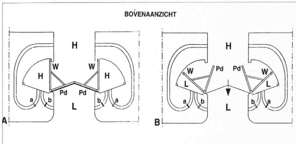
afb. 7 Werking van de waaierdeur: (A) gesloten deur met hoog buitenwater, (B) openen van de deur bij hoog buitenwater en laag binnenwater. Pd= puntdeur en w= waaier. a= schuiven in de riolen naar het buitenfront, b= schuiven in de riolen naar het binnenfront; H= hoogwater en L= laagwater. Uit: Sluizen en stuwen van G.J. Arends
