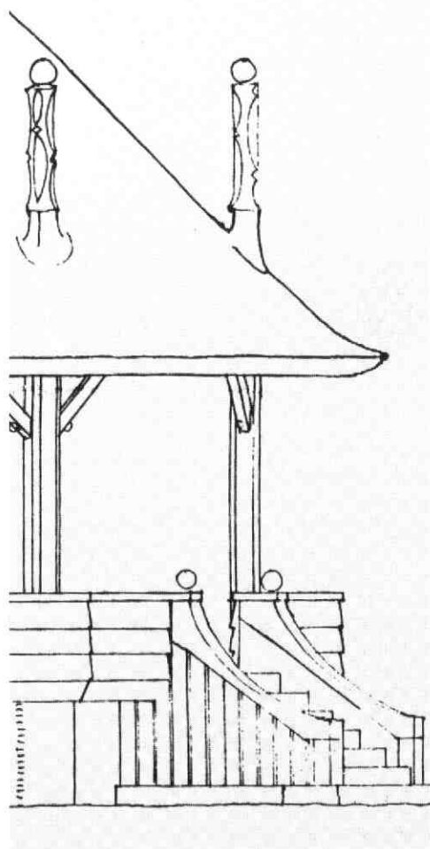
Detail van de bouwtekening, 1 : 50, uit 1925. Boven zien we een gedeelte van de kegelvormige kap met 2 van de 6 eikehouten bergroeden. Deze zijn boven de kap rond uitgehold en de top werd gevormd door een bal. Let op de fraaie toegangstrap; deze heeft 1 bloktrede en 7 optreden.
