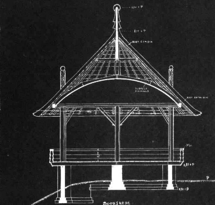
DOORSNEDE
