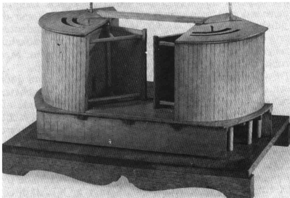
afb. 9 Model van een waaier- sluisdeur. Vermoedelijk uit de nalatenschap van Jan Blanken, thans in het Rijksmuseum.
