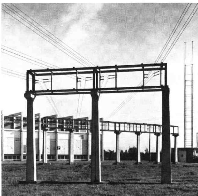
3. Portalen welke de kabels het zenderge- bouw naar de antennes geleiden.
