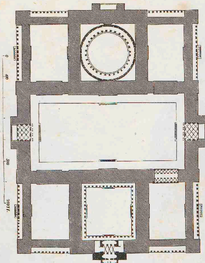
1. Ontwerp voor Whitehall door Imigo Jones (1572—1652).
