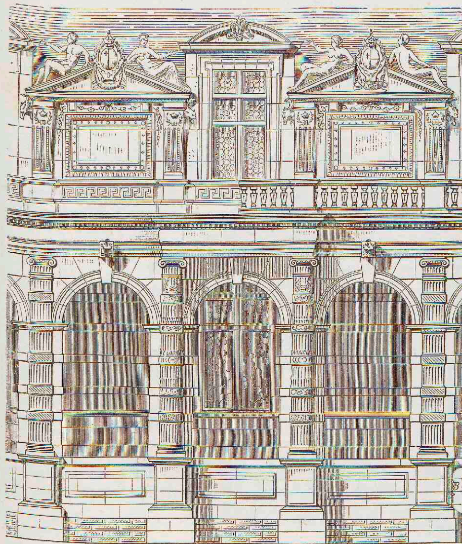
2. Tuilerieën. Gedeelte des gevels aan de tuinzijde.
