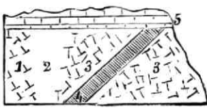
FIG. 17. KLIPPE AM SERRO COLORADO.
