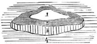
FIG. 24. GEODE IM PHOSPHORIT VON HERMANUS.
