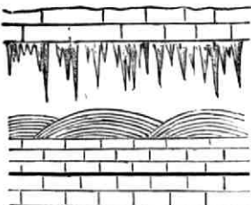
FIG. 27. GROTTE BEI FONTEIN, mit Sinterbildungen ausgekleidet. Kalkbänke in schwebender Lage bilden ihr Liegendes und sind seewärts steil abgebrochen.
