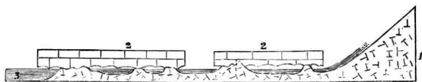
FIG. 28. EROSIONSERSCHENUNGEN BEI ANTIKURIE. — 1. Diabas. — 2. Korallenkalk. — 3. Meer.
