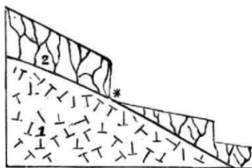
FIG. 33. QUELLENBILDUNG. 1. Diabas. — 2. Zerklüfteter Kalkstein. — * Ursprungsstelle der Quelle.
