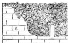
FIG. 20. AN DER TEUFELS- KLIPPE BEI FEIK.
