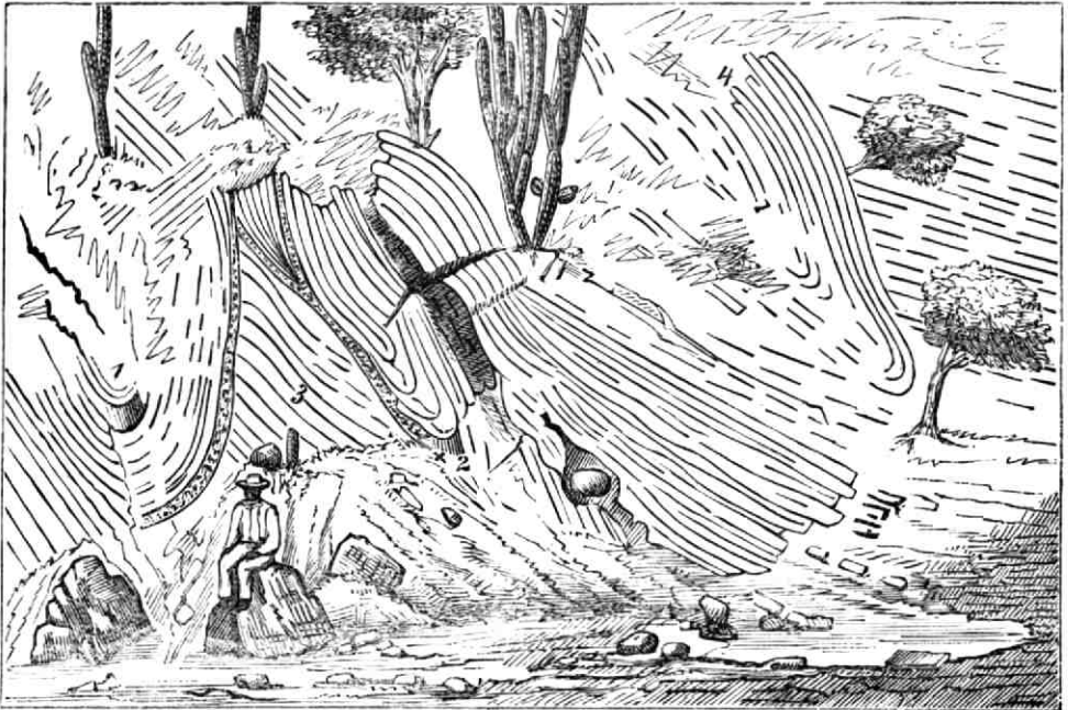
FIG. 9. GEFALTETE KIESELSCHIEFER AM FUSSE DES ST. CHRISTOFFELS.
