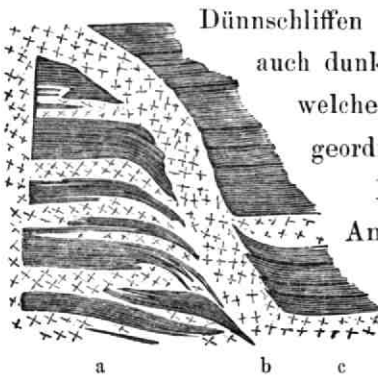
FIG. 39. SCHLIEREN IM GRANITE DES SISABO.
