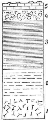
FIG. 19. PROFIL AM SERRO CULEBRA.
