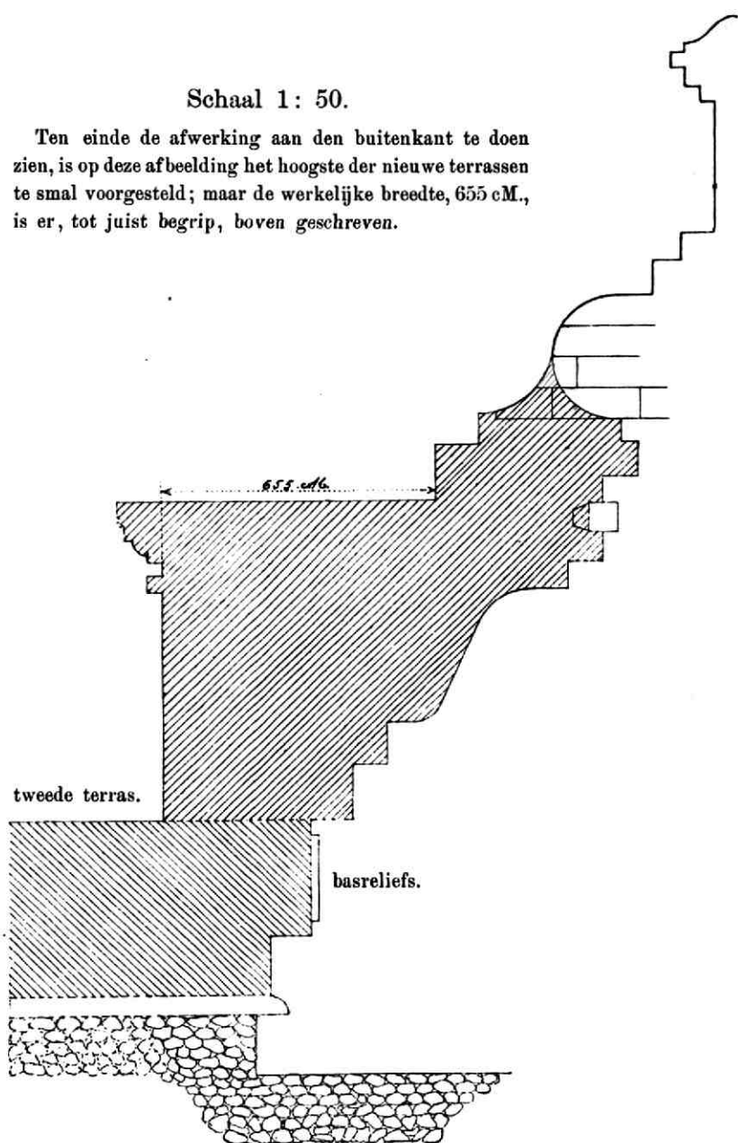
Pl. I. Doorsnede van den begraven voet van Bārā Boedoer, volgens IJzerman.
