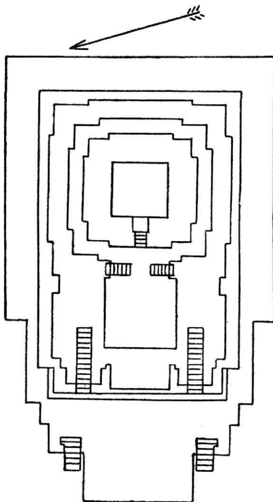
Pl. X. Plattegrond van Tj. Toempang, 1:200, naar Verbeek (ms.).
