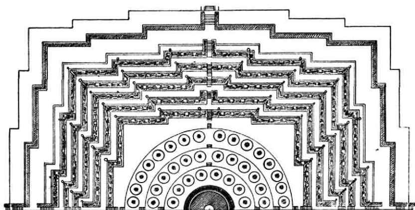
Pl. IV. Halve plattegrond van Bārā Boedoer, 1:1200.
