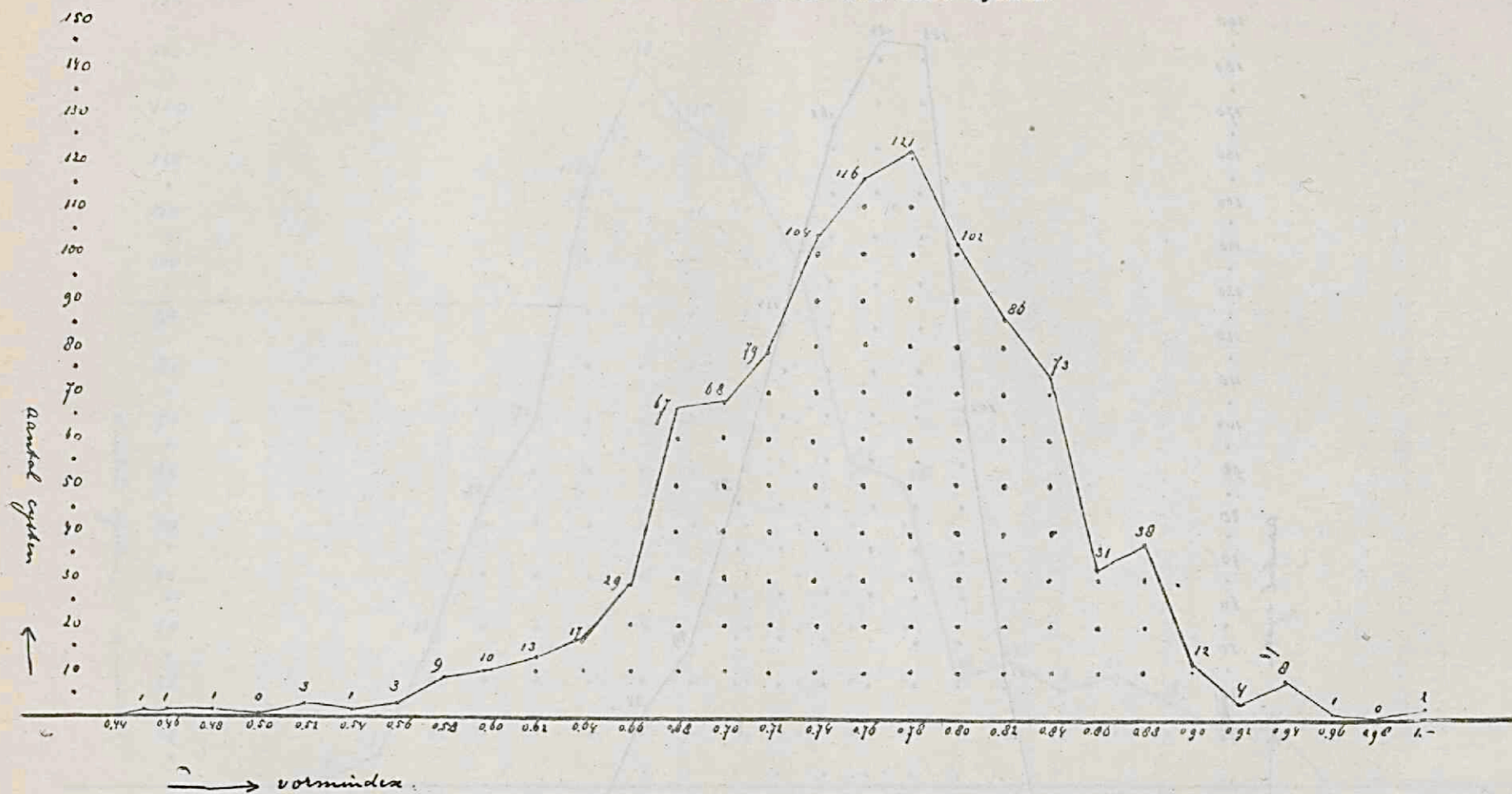
CURVE III. Vormindices van 1000 cysten.
