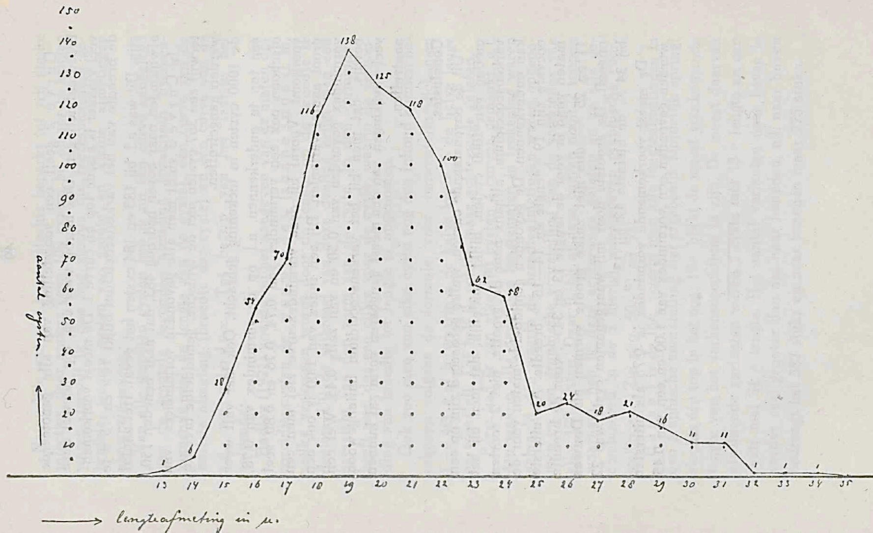
CURVE I. Lengteafmetingen van 1000 cysten.
