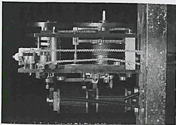
E—2. Chronoskoop van Hipp.
