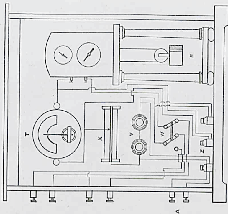
Schema der opstelling van den chronoskoop van Hipp.
