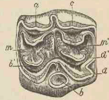
Fig. 197. Hipparion gracile Kaup. Ob. Miocaen. Pikermit bei Athen. Ob. Backzahn von unten \frac{1}{4} .
