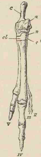
Fig. 71. Rechter Hinterfuss von Känguruh \frac{1}{8} nat. Gr. (nach Flower).
