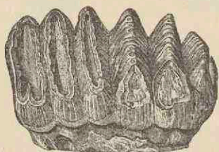
Fig. 37. Polylophodonte Oberkiefermolar von Stegodon (verkleinert).
