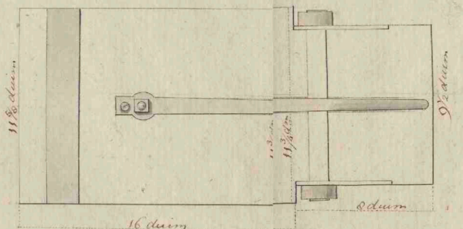
Stell Hoût van voren te zien
