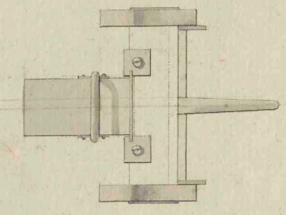
Stell Hoût van agteren te zien
