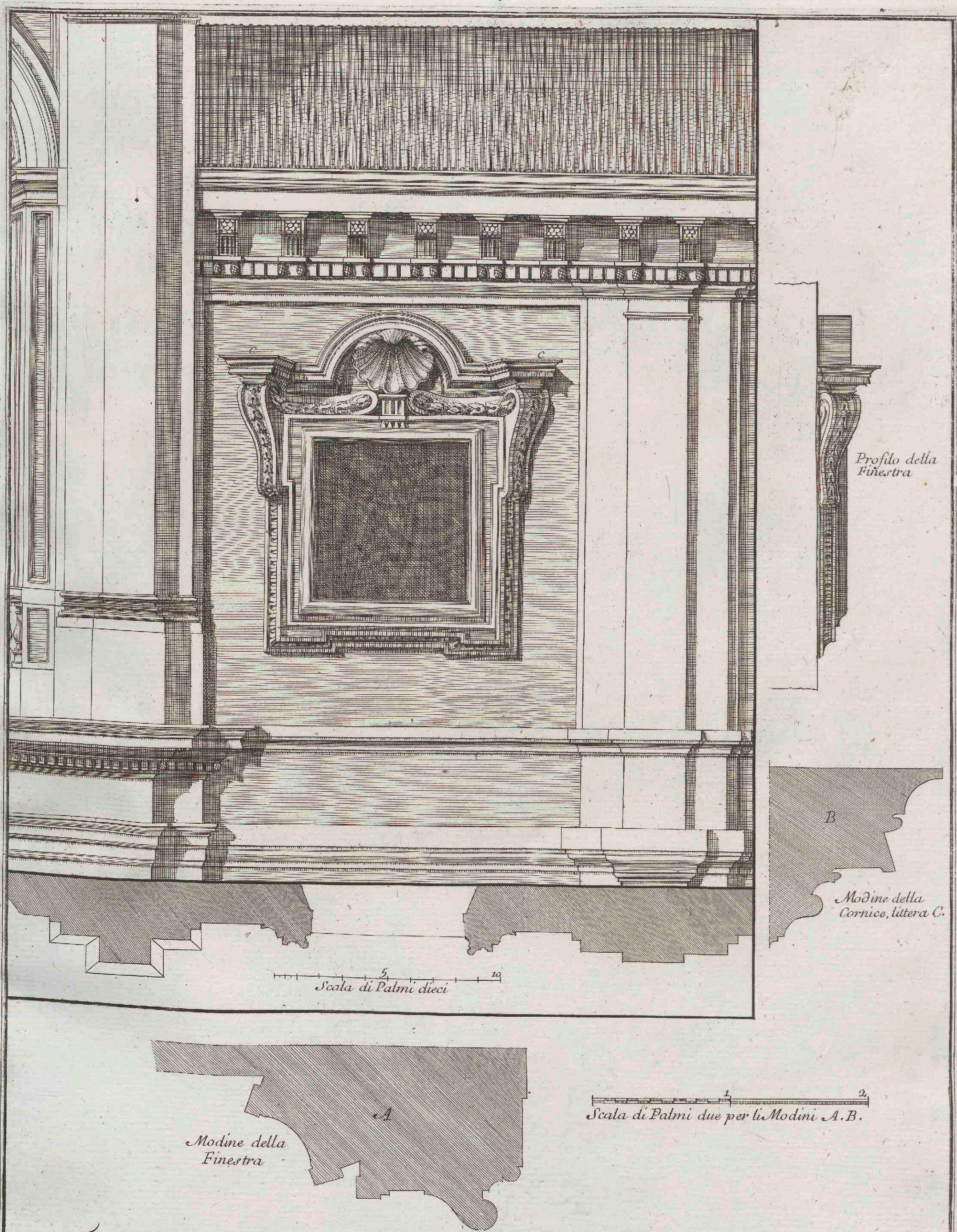
Finestra del terzo piano della facciata del Palazzo Barberino del Sig. re Principe di Pelestrina. Architettura del Cavalier Borromini.
