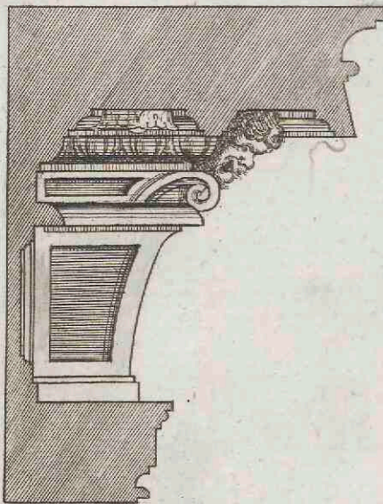
Profilo del Cornicione con uno de Modelli
