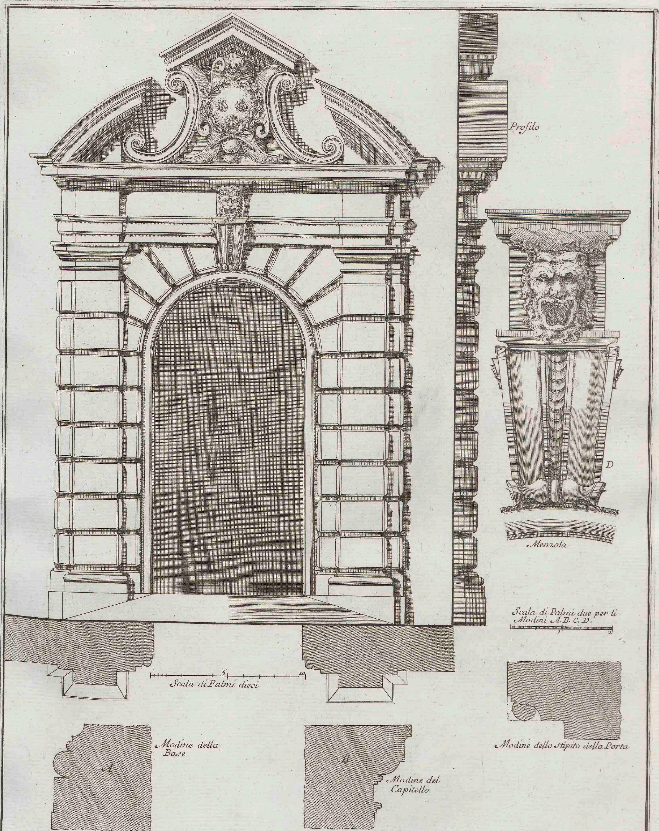
Porta del Teatro delle Commedie del Palazzo Barberino del Sig. re Principe di Pelestrina. Architettura del Cavalier Pietro Berrettini da Cortona.
