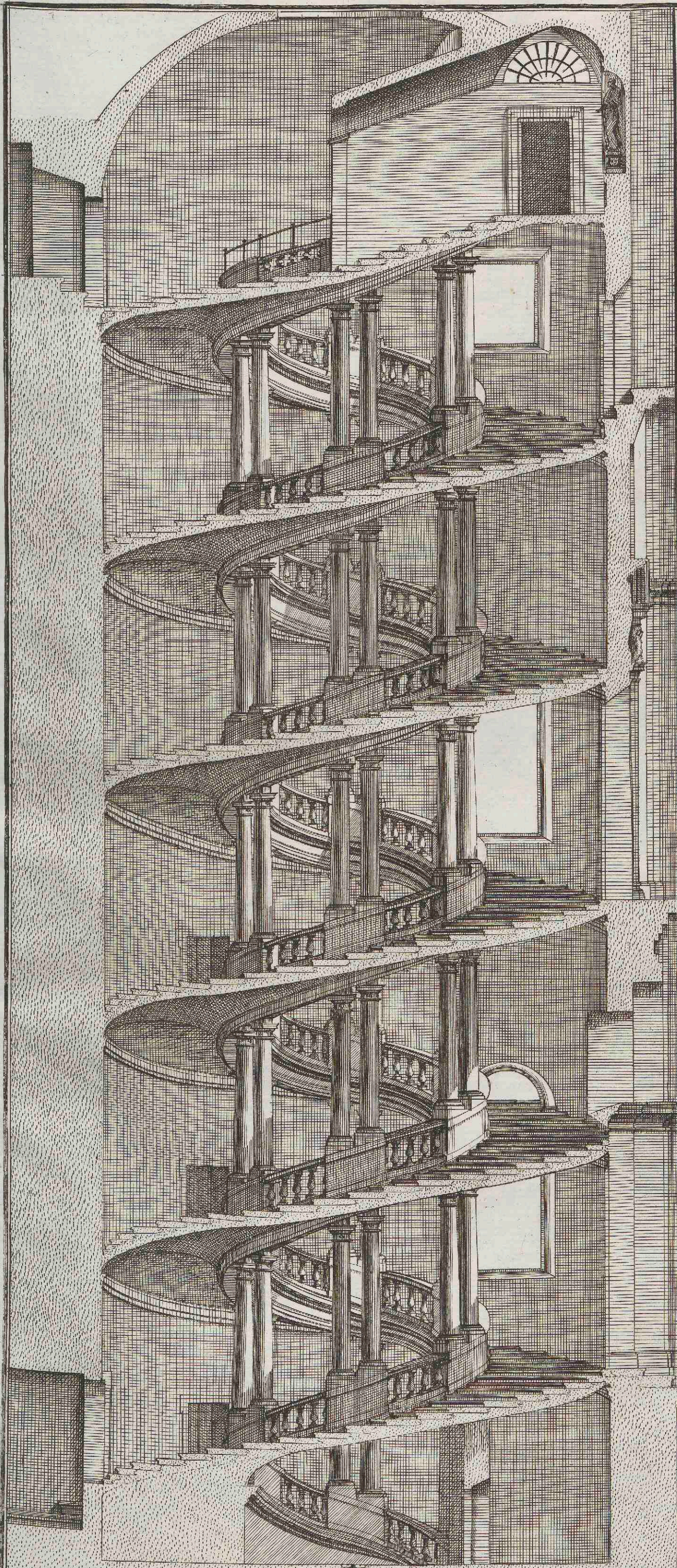
Scala a Samaca del Palazzo Barberino del Sig. ro Principe di Palestrina. Architet. ta del Cavalier Borromini. Nella Stamp. a di Dom. no de Rossi in Roma alla Pace.
