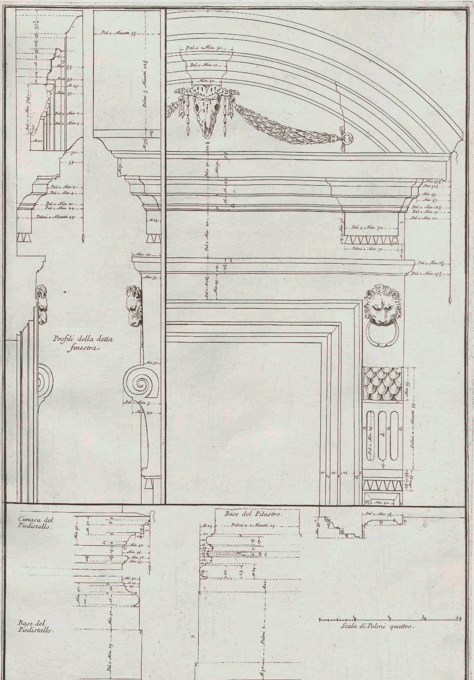
Modini dell'antecedente finestra del terzo ordine.
