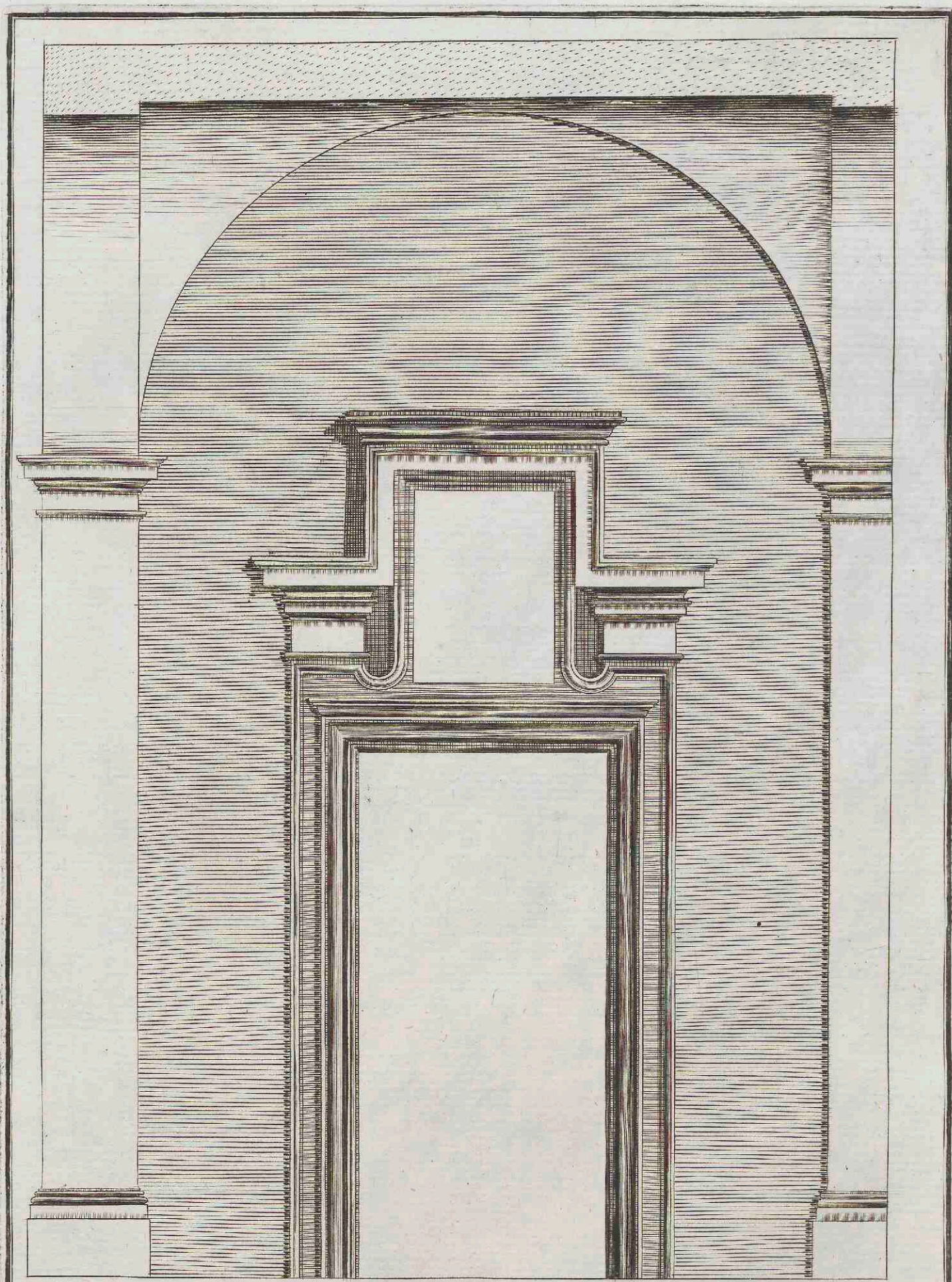
Modine delli Stipiti della Porta
