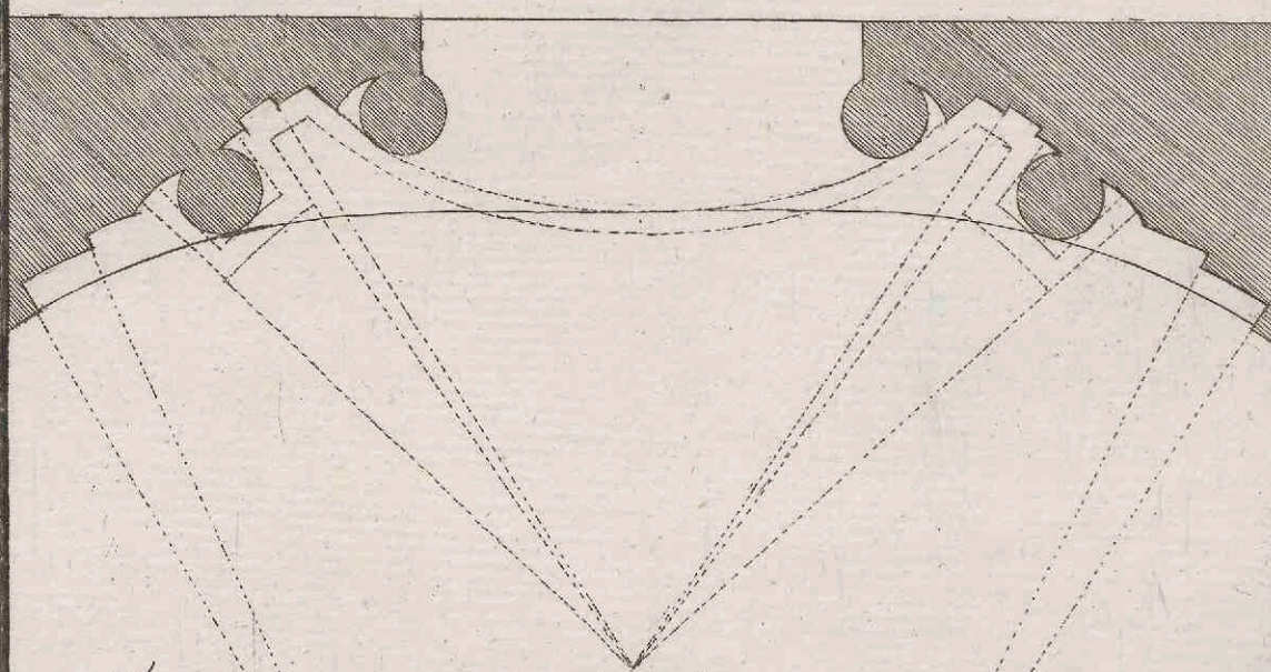
Finestra principale al primo Ordine sopra la porta della Facciata del Collegio di Propaganda Fide Architettura del Cavalier Borromini
