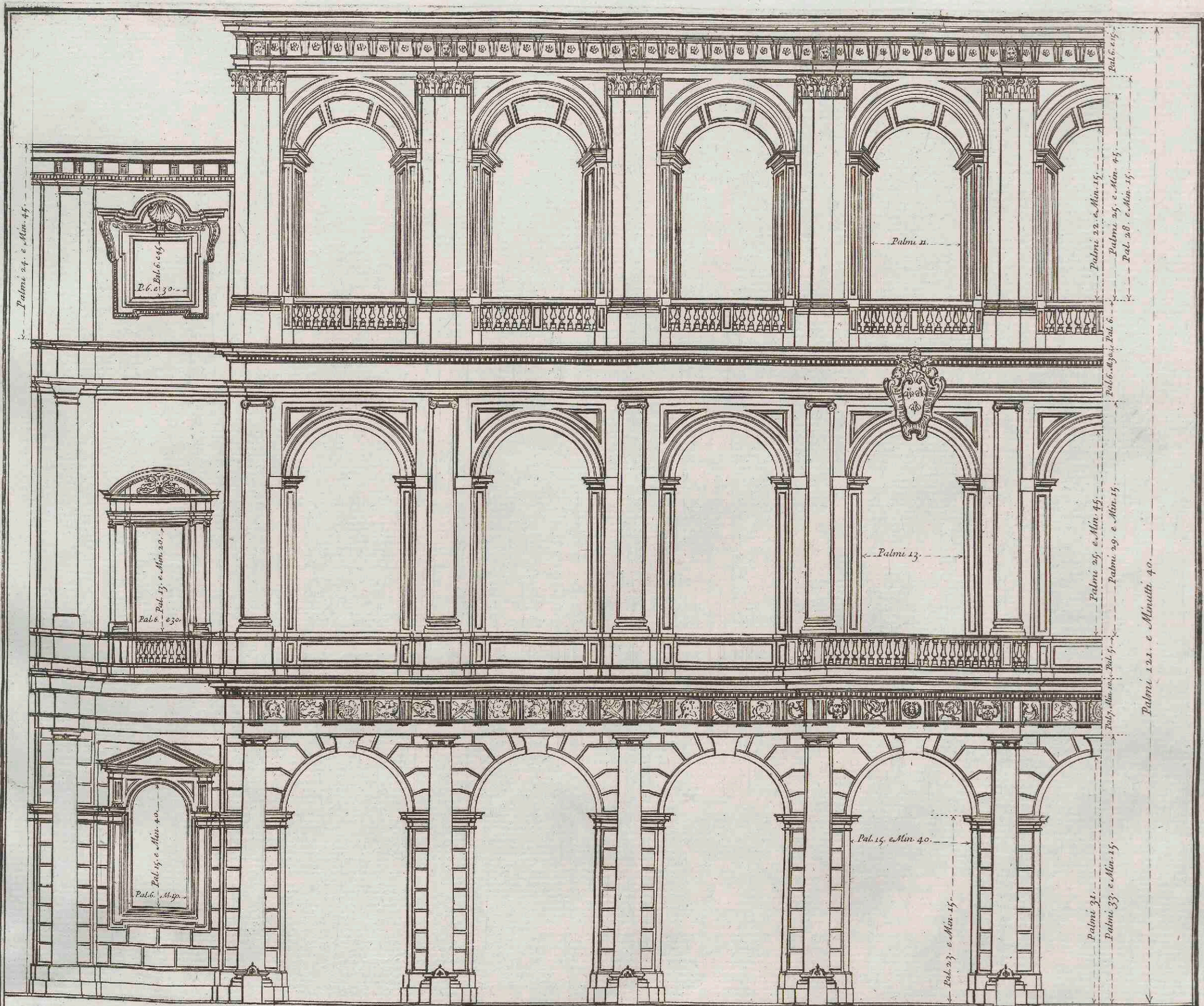
Parte del Prospetto della facciata del Palazzo Barberino del sig. ro Principe di Pelestrina, con le sue dimo- strazioni a parte nè fogli seguenti
