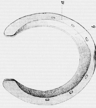
Fig. 2. RECHTER VOORRUIZER, VAN BOVEN GEZIEN. a , draagrand; b , afsteltende vlakke.
