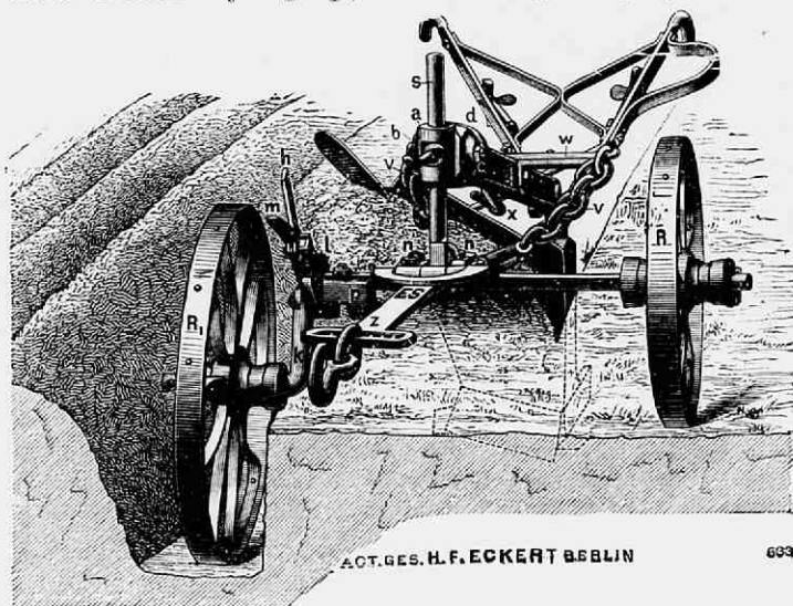
Fig. 78. Ploeg voor het bewerken van heidevelden tot bosch. Zie de beschrijving hierachter.
