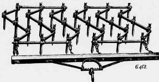
Fig. 142. Laacke's nieuwe akkereg „Adler” met verstelbare, driekantige holle tanden. A. tand van de „Adler” eg.
