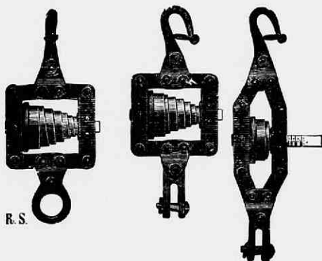
Fig. 73. Schokbreker en eenvoudige krachtmeter van R. Sack, te Plagwitz. Agent L. Nagel & Co., Arnhem.
