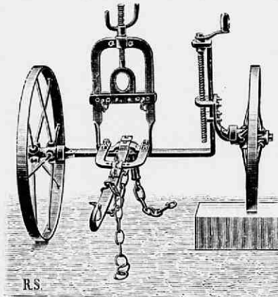
Fig. 106. Voorstel van Sack's ploeg met inrichting om het kussen en de as van het linkerrad door middel van een schroef te stellen.
