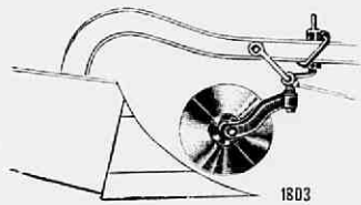
Fig. 84. Ploegboom met kouterschijf aan Eckert's ploegen.
