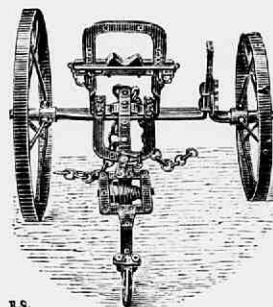
Fig. 74. Aanwijzende hoe een schokbreker en krachtmeter aan een Sack's ploeg geplaatst wordt.
