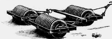
Fig. 152. Driedeelige enkele ringrol van Gross en Co. In elke rol 11—13 ringen; doorsnede der ringen 35 cM.
