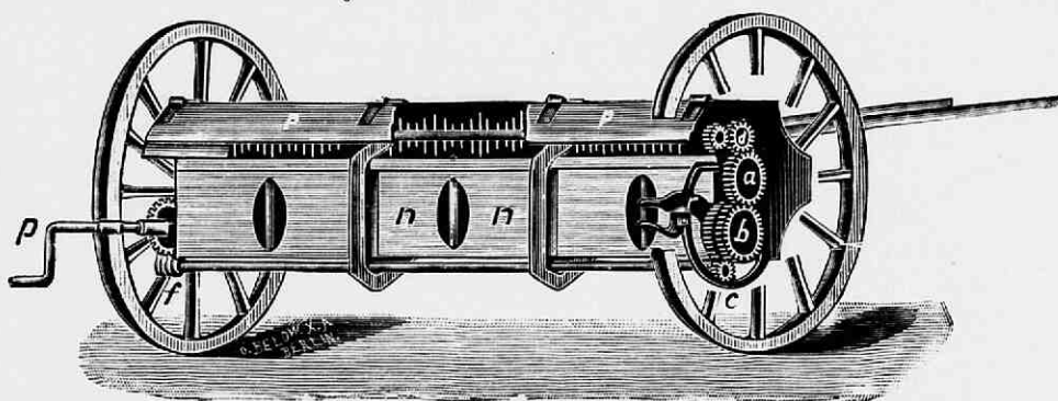
Fig. 186. Kunstmeststrooier van Schlör, Barth a/d Oostzee, van achteren gezien, om aan te wijzen hoe de as m en het rad l , Fig. 188, automatisch door middel van de raderen a , b enz. door de machine bewogen worden.
