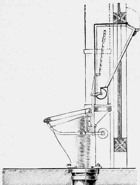
Fig. 180. Vrijstaande zittrechtter van geëmailleerd ijzer met automatische turfinolmstrooier en turfinolmhouders die van buiten gevuld kan worden.
