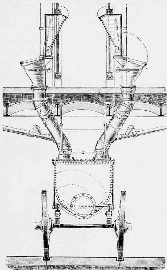
Fig. 181. Inrichting van turfmoelm-closets voor kazernes enz. met ton op radereen, van C. Maquet te Heidelberg.
