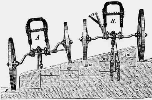
Fig. 107. Voorstel van Sack's ploeg met draai-bare as voor het ploegen op hellend terrein. In A wordt, van den toeschouwer af, de strook I en in den stad B, naar den toeschouwer toe, de strook Iα geploegd. In beide gevallen is het middelstuk der as horizontaal en even hoog geplaatst. De verplaatsing der assen geschiedt met den hefboom α.
