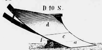
Fig. 92. Sack's ploeglichaam met lang rister voor zware kleigronden. Het rister bestaat uit verschillende platen a , c , d , en een strijkijzer b ; f , landzijde; g , ploegzool.
