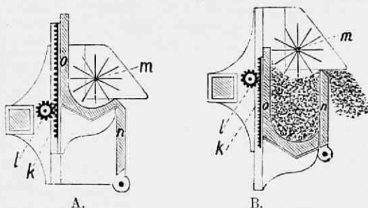
Fig. 188. Idem in doorsnede; A als de bodem van den bak in zijn hoogsten stand en nagenoeg ledig is, B. in zijn laagsten stand met gevulden bak: m , as met pinnen die de mest uitstrooien: o , het beweegbare deel van den bak, dat door de getande staaf k en het tandrad l op en neer kan worden bewogen.
