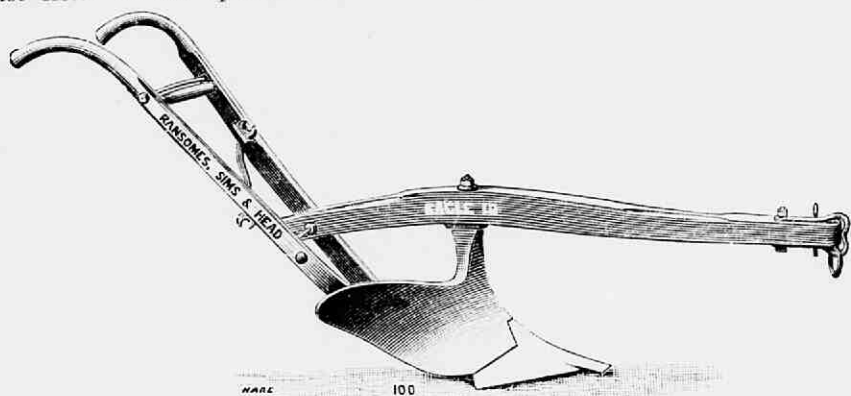
Fig. 100. Ransomes' Engelsch-Amerikaansche balansploeg, met hoofd en rister, zool en molbord uit één stuk. Ploegen van 7—22 cM. diep en 13—30 cM. breed.
