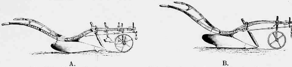
Fig. 86. Howard's ploegen van verschillende afmetingen en zwaarte; Agent wed. Massée en Zoon te Goes; ploegen van 7 tot 23 c.M. diep; A met kouter, voorschaaar en twee wielen, B met kouter en één wiel; kunnen ook als balansploeg zonder wielen genomen worden.
