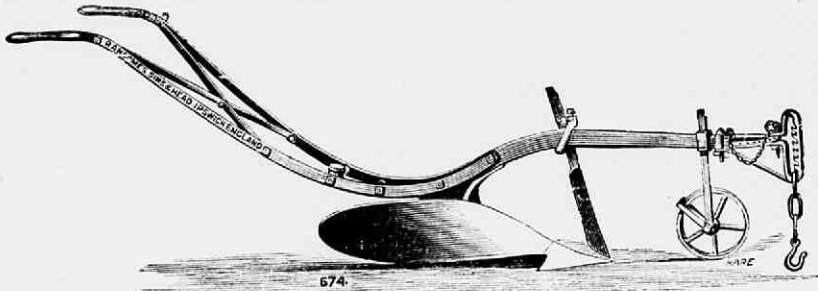
Fig. 82. Ransome's ploeg, geschikt voor lichte gronden, met één wiel, kan ook als balansploeg gebruikt worden; met hoofd of raam (frame) van smeed- of gietijzer. Voor het dieper of minder diep ploegen (van 8 tot 15 c.M. diepte bij 15 tot 18 c.M. breedte der voren) kunnen verschillende scharen genomen worden.
