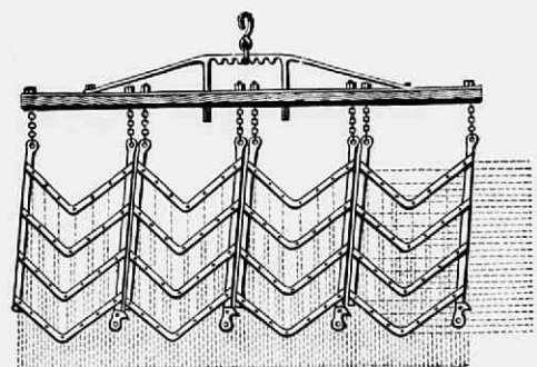
Fig. 141. Laacke's eg voor fijne verkrumming van den grond met dubbele werking. A. tand.
