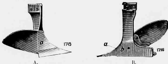
Fig. 116. Ploeghoofd met rister van Eckerts ploegen, A. van rechts, B. van links gezien. Het bovenstuk a en de landzijde en zool b zijn met pantserplaten van glashard staal voorzien, die het hoofd voor slijting beschermen.
