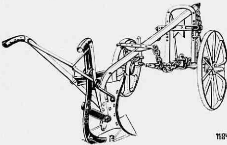
Fig. 165. Grondwoeler (Grubberfuss) van Eckert's éénscharige ploegen.
