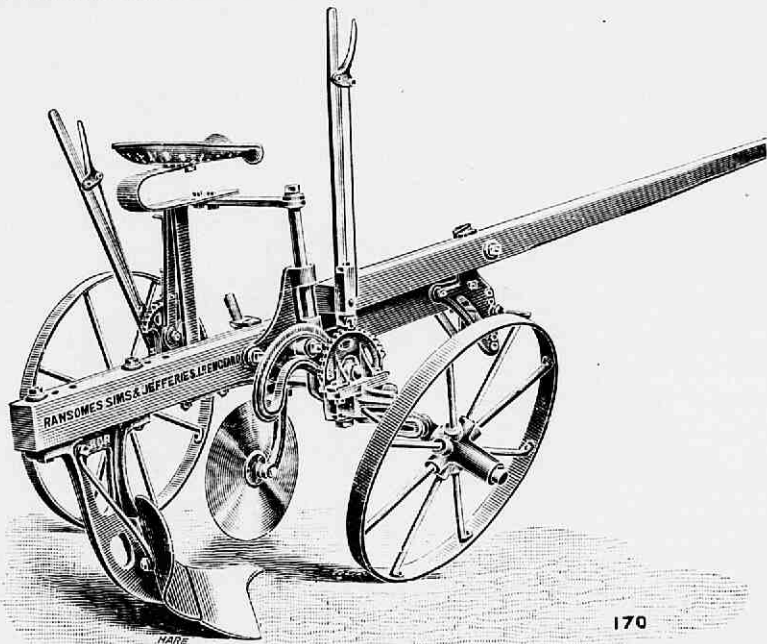
Fig. 113. Ransomes' Sulky-ploeg met zitplaats voor den ploeger. De ploeg kan met den hefboom naast den ploeger door dezen of ook automatisch door de trekdieren buiten het werk gezet, dat is de boom met de daaraan bevestigde huizen opgebeurd worden. De diepte der voren kan door den ploeger van zijne zitplaats worden geregeld. Zij ploegen 10 tot 18 cM. diep en 36-45 cM. breed, maar kunnen ook als tweehuizige ploegen geleverd worden en dan is, bij dezelfde diepte, de breedte 30 cM.
