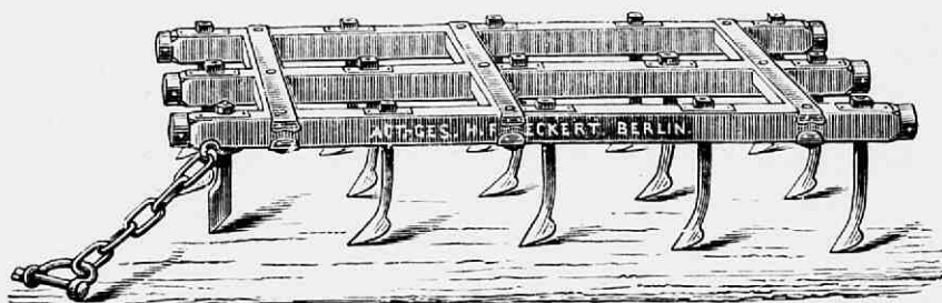
Fig. 157. Kruimelaar (Krümmer) van Eckert; Agent Kouveld te Amsterdam; worden ook driehoekig geleverd.
