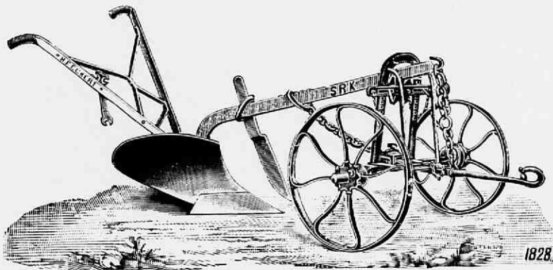
Fig. 109. Eckert's stalen ploeg voor gronden van gemiddelde zwaarte, agent Ch. R. Kouveld, Amsterdam, met voorstel en kouter en Ruchadler-risten; kunnen ook met schroefvormig rister genomen worden; ploegen 26—28 cM. breed en 20—26 cM. diep.
