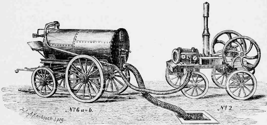
Fig. 183. Latrinen luchtpomp (systeem Lenoir) van Knobloch, Leipzig, agent Ch. R. Kouveld, Amsterdam, voor het reukloos ledigen van secreetputten, gierputten enz.: rechts wagen met luchtpomp en manometer, kachel met schoorsteen en luchtbuis; links: aanvoerbuis voor de beer en beerton met peilglas.
