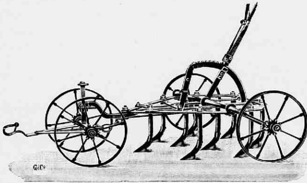
Fig. 158. Stelbare en op raderen vervoerbare cultivator of kruimelaar (Krümmer) van Gross en Co. te Leipzig-Eutritzsch.
