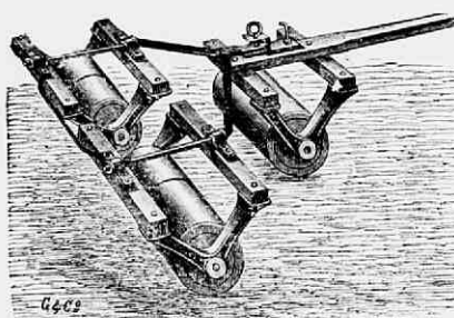
Fig. 145. Driedeelige gladde rol met düsselboom van Gross en Co. te Leipzig-Eutritsch, van hout (of ijzer): die van hout 45 en 50 cM. en die van ijzer 40 cM. in middellijn. Lengte 2.00 à 2.30 cM.
