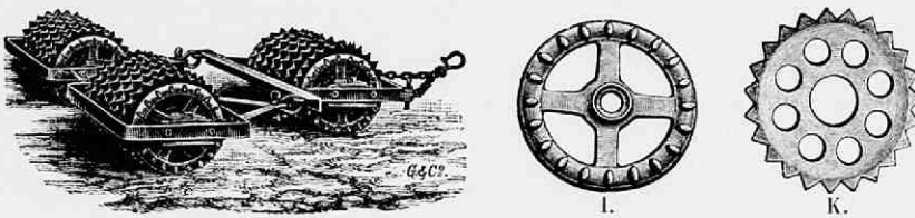
Fig. 155. Gecombineerde Croskill- en Cambridge-rol. Van ringen 1 7 à 8 en van ringen K 6 à 7 in één rol.
