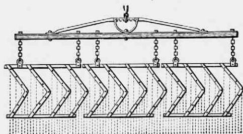
Fig. 140. Laacke's eg voor fijne verkrumming van den grond met enkelvoudige werking. A. tand.
