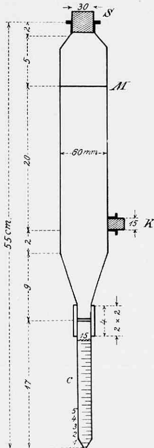
Fig. 71. Slibtoestel van Sikorsky. M, merk; S en K, caoutchouc-stoppen; C, verdeelde buis.
