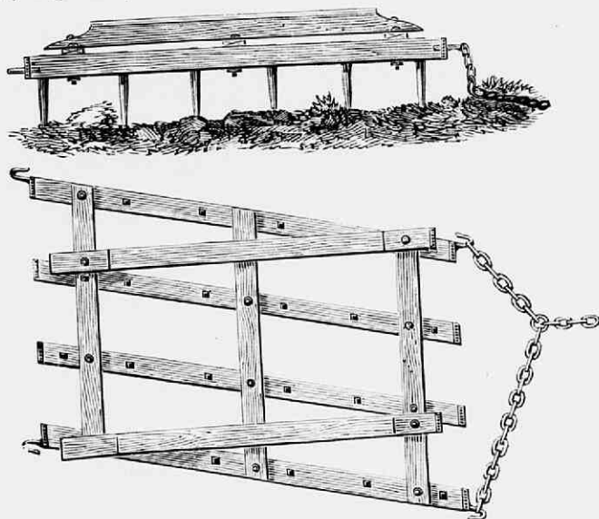
Fig. 129. Parallellogramvormige egge of eg van Valcourt.
