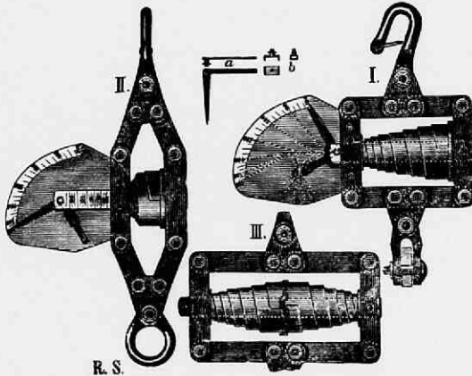
Fig. 75. Schokbreker en krachtmeter met wijzer van R. Sack, te Plagwitz. Agent L. Nagel & Co., Arnhem: I in rust, II samengedrukt, III met dubbele veer. De wijzerplaat is aan het raam, de staaf, aan welks niteinde de gebroken hefboom als wijzer zit, aan de veer bevestigd. In de wijzerplaat is eene gleuf, b , waarin de arm a van den hefboom zich beweegt 1) .
