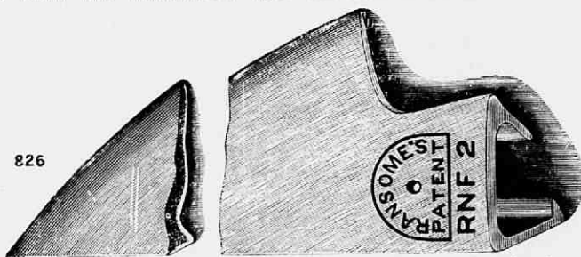
Fig. 115. Ransomes ploegschaar, doorgebroken om de geharde onderzijde, voorgesteld door de witte lijn, te doen zien.
