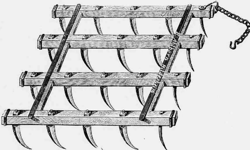
Fig. 159. Schotsche lepelegge van Ahlhorn te Hildesheim.
