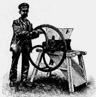
Fig. 189. Kunstmestbreker geleverd door de wed. Massée en zoon te Goes.
