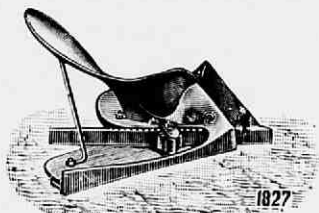
Fig. 117. Inrichting der beetel aan Eckert's ploegen, van onderen gezien. De beetel steekt ongeveer 3 cm. voor de schaar uit en is aan beide einden gescherpt, zodat zij omgekeerd kan worden.
