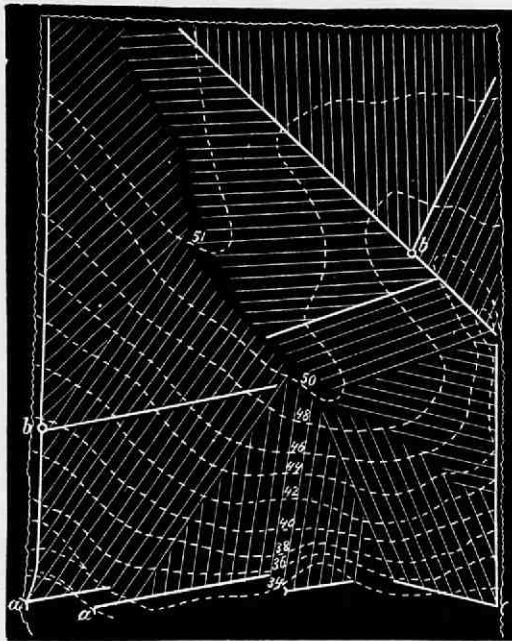
Fig. 75. Drainageplan eener moerassige weide (Crevillar Dept. du Nord) op 0.0002; a , uitloopen in het laagste gedeelte van het terrein; b , kijkgaten om te kunnen zien waar de buizen verstopt zijn. De kromme stippellijnen verbinden de plaatsen van gelijke hoogte, door de daarbij geplaatste cijfers in meters boven de oppervlakte der zee aangegeven. De evenwijdige lijnen zijn zuigdrains, de andere hoofddrains.
