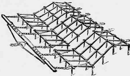
Fig. 133. Howard's origineele zig-zag eg. Agent voor deze en andere eggen van Howard, wed. Massée en zoon te Goes.
