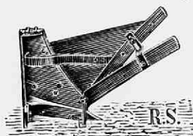
Fig. 93. Ploeglichaam met verstelbaar strijkijzer (zie Fig. 92), van achteren gezien. Van R. Sack, Leipzig-Plagwitz, Agent L. Nagel en Co., Arnhem.
