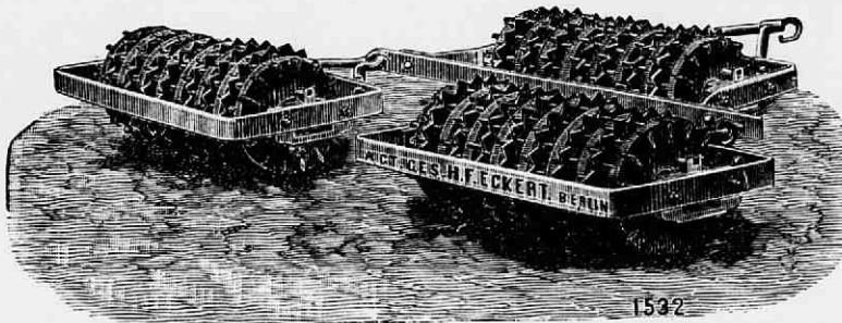
Fig. 151. Kluitenbreker of Cambridge rol van Eckert, Agent Kouveld te Amsterdam. De breedere gladde ringen zijn 38 cM. in middellijn en 8 cM. breed, de smallere getande ringen 42 cM. in middellijn en 2 cM. breed. Beide draaien los om de as, maar de tweede hebben in het midden eene grootere opening, die haar eene grootere speelruimte om de as veroorlooven.
