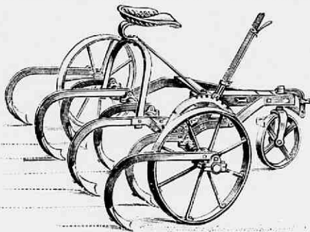
Fig. 162. Howard's cultivator voor het uittrekken en afsnijden van distels.
