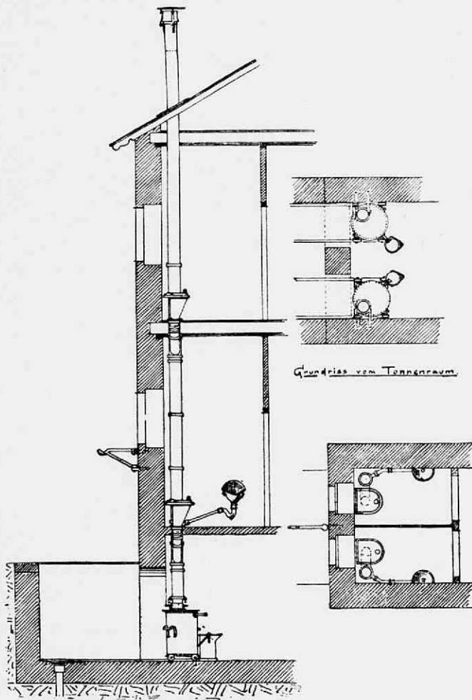
Fig. 179. Inrichting van het Heidelberger tonnenstelsel voor twee verdiepingen met urinoir en luchtbuis met ventilator. Grundriss vom Tonnenraum is platte grond van het tonnenhok in het sous-terrein.
