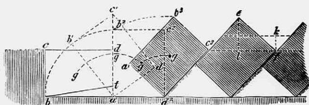
Fig. 123. Voorstelling, hoe de vurg bij het ploegen gekeerd wordt. abcd , doorsnede der vurg; ab^1c^1d^1 , ab^2c^2d^2 en ab^3c^3d^3 de standen, die zij achtereenvolgens heeft; g zwaartepunt.
