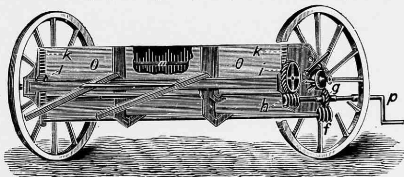
Fig. 187. Idem van voren gezien. De kruk p en de daarmede in verbinding staande deelen dienen om, als de bak ledig is, den beweegbaren bodem naar beneden te brengen.
