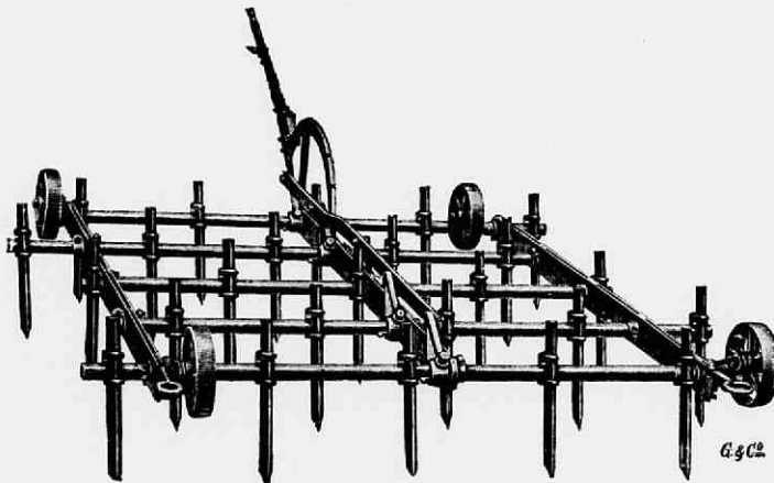
Fig. 143. Eg met verstelbare tanden van Gross en Co. te Leipzig-Eutritsch. De tanden zijn hier verticaal of in haar hoogsten stand geplaatst en werken dan 20—25 cM. diep. Zij kunnen echter ook schuin geplaatst worden en werken dan ongeveer 15 cM. diep. Buiten werking gesteld zijn zij horizontaal geplaatst, zie Fig. 144.
