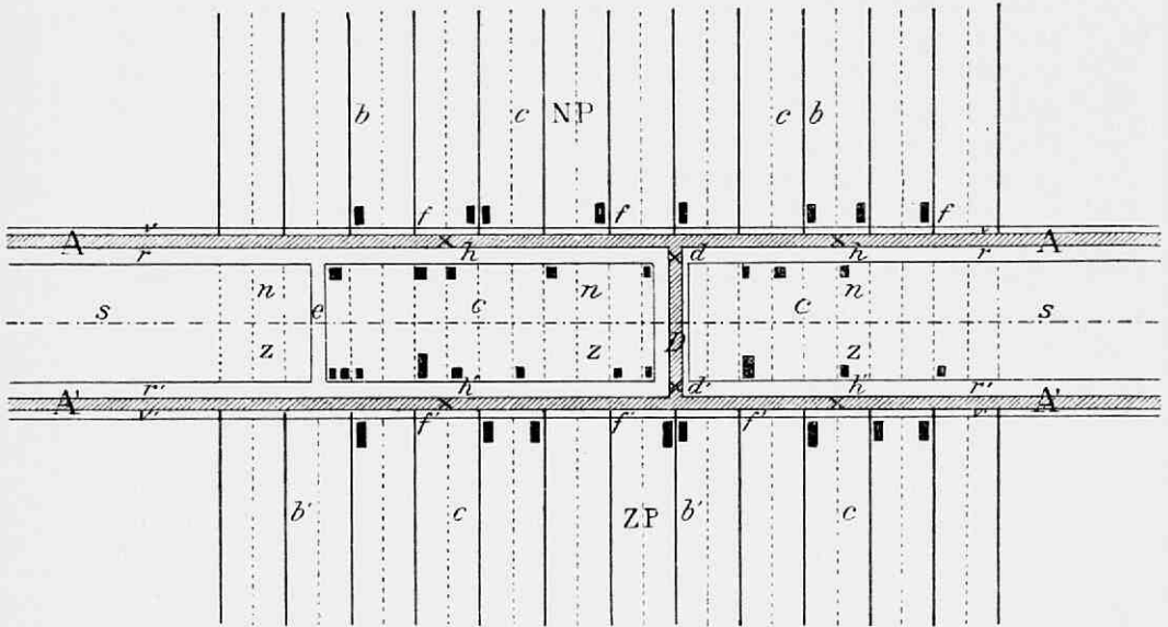
Fig. 79. Schematische voorstelling van eene veenkolonie volgens het tweekanalenstelsel: AA en A'A', evenwijdige hoofddeepen, door één of meer dwarsdiepen D verbonden, met wijken bb en b'b'; NP, noorderplaatsen; ZP, zuiderplaatsen; cc, zwetsloten tusschen de plaatsen; ss scheisloot tusschen NP en ZP; nn, noordervooraffen; zz, zuidervooraffen; rr en r'r', rijwegen over de vooraffen met dwarslanen e en draaien dd' over het dwarsdeep; vv en v'v', breede voetpaden met batten ff en f'f' over de wijken; hh en h'h', hoofddraaien over AA en A'A', voor verbinding van vv met rr en v'v' met r'r', meestal vermeerderd met eigen draaien; boerenplaatsen langs vv en v'v'; woningen met tuinen voor neringdoenden langs rr en r'r' op de vooraffen.
