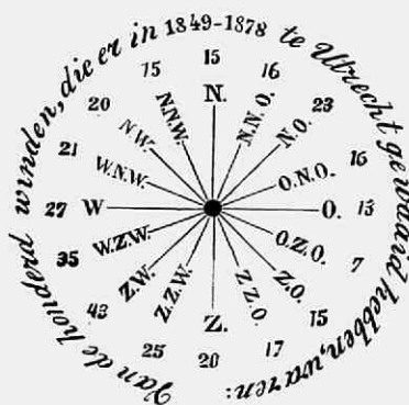
Fig. 4. Verhouding tusschen het aantal winden van 1849—1878 te Utrecht in honderdtallen.
