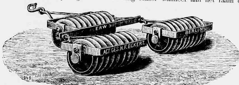
Fig. 150. Eckert's driedeelige ijzeren ringrol, Agent Kouveld te Amsterdam. De ringen zijn 34 cM. in middellijn en hebben eene breedte van 8 cM. Zij zijn draaibaar om de ijzeren as, waardoor zij zich zelve schoonhouden.
