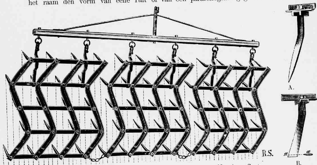
Fig. 132. Zig-zag eg van R. Sack, met kromme tanden. Agent Nagel en Co te Arnhem. A. afzonderlijke tand met doorsnede der lengte- en dwarsbalken; B. mesvormige tand, a . dwarsdoorsnede.
