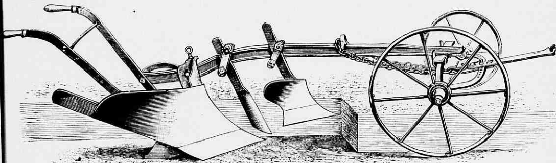
Fig. 112. Boog-asploeg van Howard, met boogvormige as in het voorstel, stelschroef, voorschaaar en kouter.
