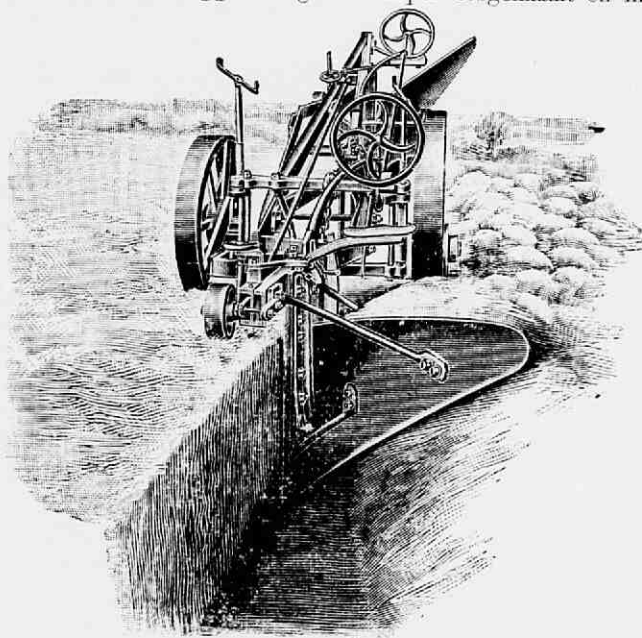
Fig. 170. Fowler's stoomploeg voor diepe grondbewerking bij heideontginning, den wijnbouw enz. in gebruik, met één ploeg-lichaam, in werking.
