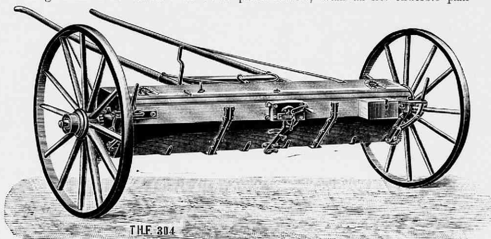
Fig. 190. Flöther's kunstmeststrooier. Agent wed. Massée en zoon te Goes. 1 glad is en door veeren en stelbouten ruimer of nauwer gesteld kan worden, terwijl het bovenste paar van tanden is voorzien welke in een rooster grijpen en zoo de brokken verbreken.
