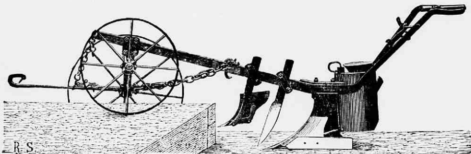
Fig. 103. Sack's Universalploeg met waterleiding van de landzijde gezien. De waterbak is van een kraan voorzien, waaraan een caoutchoucuis bevestigd is die het water naar het rister leidt.
