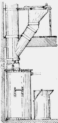
Fig. 175. Eenvoudige verbinding van een Heidelberg ton met de valbuis, zonder siphon. De zittrechters is van oudere constructie met omschieten hout.
