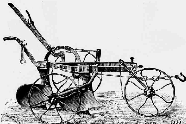
Fig. 119. Eckert's tweescharige ploeg, worden ook driescharig geleverd. Ploegen 4—18 cM. diep en 48—72 cM. breed. Agent Kouveld te Amsterdam.
