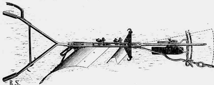
Fig. 104. Sack's Universalploeg voor het ploegen van smalle strooken tusschen greppels van boven gezien. De ploeg is gesteld voor het afploegen der laatste vurg aan de greppels.
