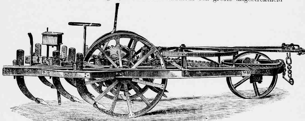
Fig. 169. Zich zelve lichtende zoogenaamde „turning” stoomcultivator van John Fowler & Co. te Maagdeburg, met 3 tot 13 tanden.
