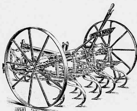
Fig. 160. Ransomes' cultivator, Bamford's patent, met zich zelf scherpemde omkeerbare messen aan veerkrachtige ijzers bevestigd die door een hefboom en door veeren matig in den grond gedrukt worden.
