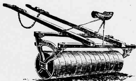
Fig. 146. Howard's segment-rol, 50—100 cM. in diameter en 2.40 M. lang. Agent wed. Massée en Zoon te Goes.
