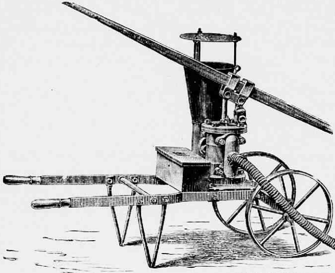
Fig. 184. Eenvoudige handluchtpomp voor het ledigen van secrete- en gierputten van Knobloch te Leipzig. Agent Kouveld, Amsterdam.
