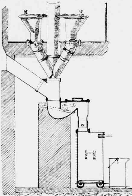
Fig. 178. Inrichting van het Heidelberger tonnenstelsel voor twee woningen met siphon en luchtbuis.
