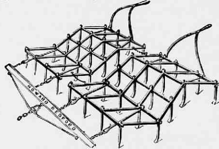
Fig. 134. Howard's diepgaande eg met staarten.
