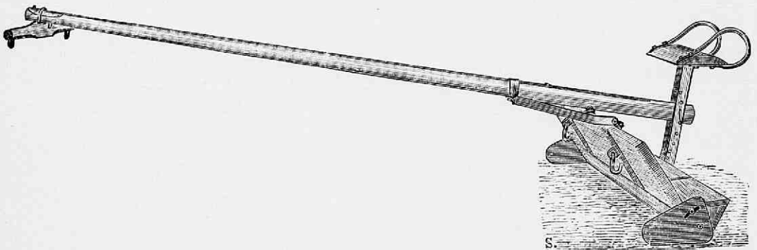
Fig. 166. Sack's akkersleep, Agent L. Nagel en Co. Arnhem.
