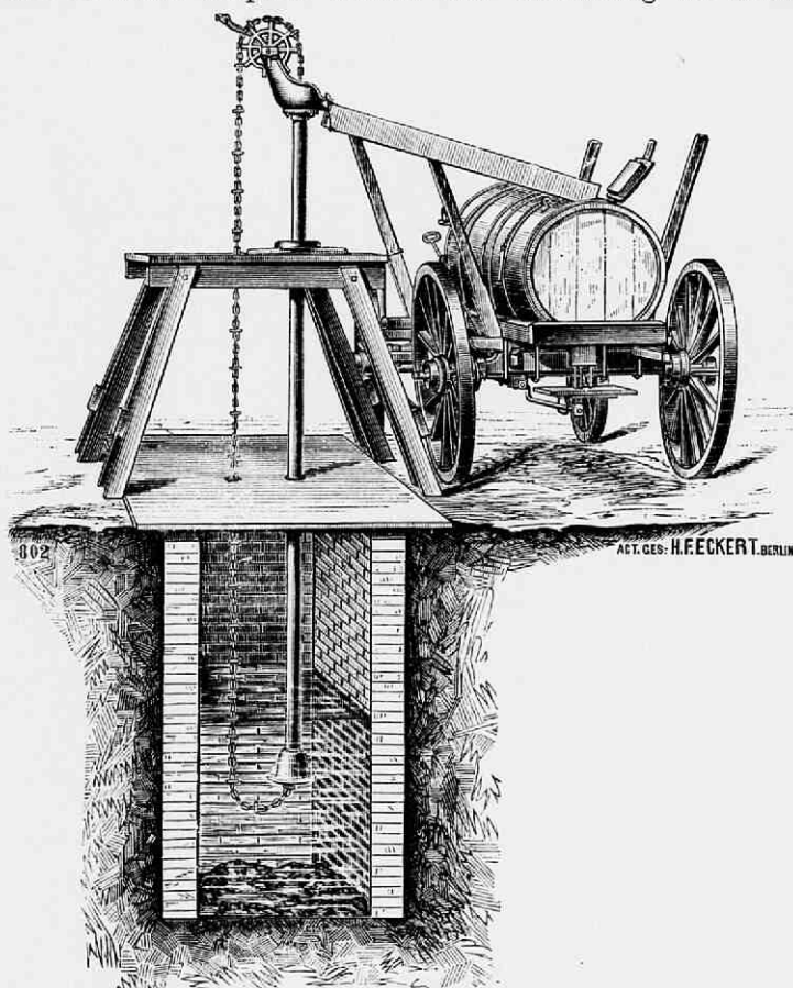
Fig. 192. Gemetselde gierput met kettingpomp van Eckert te Berlijn, Agent Ch. R. Kouveld te Amsterdam.
