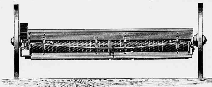
Fig. 191. Kunstmeststrooier volgens het octrooi van Schwartz. Agent wed. Massée en zoon te Goes.
