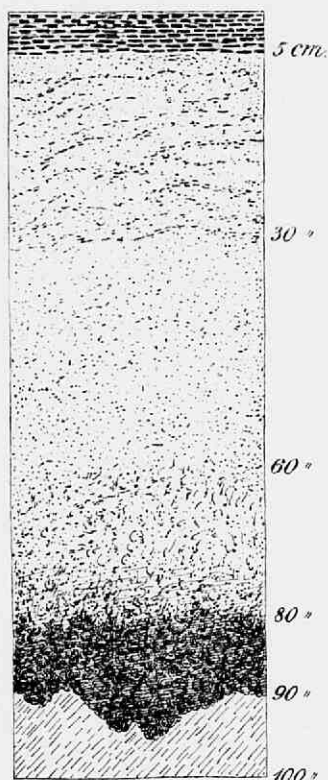
Fig. 72. Profiel van eene zandoerbank uit het Barrewinkelveld onder Apeldoorn: tot 5 cM. turfachtige humus; 5—60 cM. uit geïloegd grijs zand, waarvan tot 30 cM. gemarmerd; 60—80 cM. begin der bankvorming wel geel gekleurd maar nog niet hard; 80—90 cM. harde oerbank; 90—100 cM. ondergrond.
