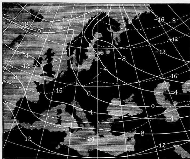
Fig. 2. Zomer- en wintertemperatuur in Europa.
