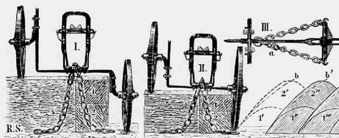
Fig. 105. Voorstel van Sack's diepploeg: I, in zijn diepsten; II, in zijn minst diepen stand; III, Regulateur van boven gezien. Daaronder aangeduid hoe de grond wordt omgewerkt. a, schroef met dubbele moer om de linker-ketting, aan den dwarsbalk op den ploegboom bevestigd, langer of korter te maken. 1, bovenste, 2, onderste laag omgeploegde aarde; de stippellijnen bij b b' wijzen aan hoe de omgeploegde vurg er uitziet als het strijkijzer e, zie Fig. 92, gebruikt wordt.
