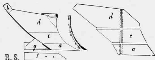
Fig. 118. Vervangbare deelen aan Sack's ploeghoofd, I, verbonden, II, afzonderlijk: a , schaar; c , middelplaat; d , bovenplaat; f , molbord of landzijde; g , zool met schroef; h , verbindingsplaat.
