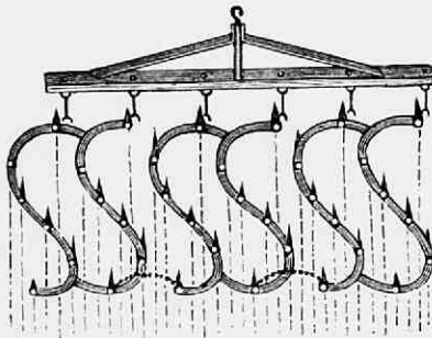
Fig. 136. Laacke's S-vormige akker-eg, 3 tweebalkige gekoppeld, worden ook drie- en vierbalkig en met rechte en kromme tanden geleverd door Gross en Co. te Leipzig-Eutritzsch.
