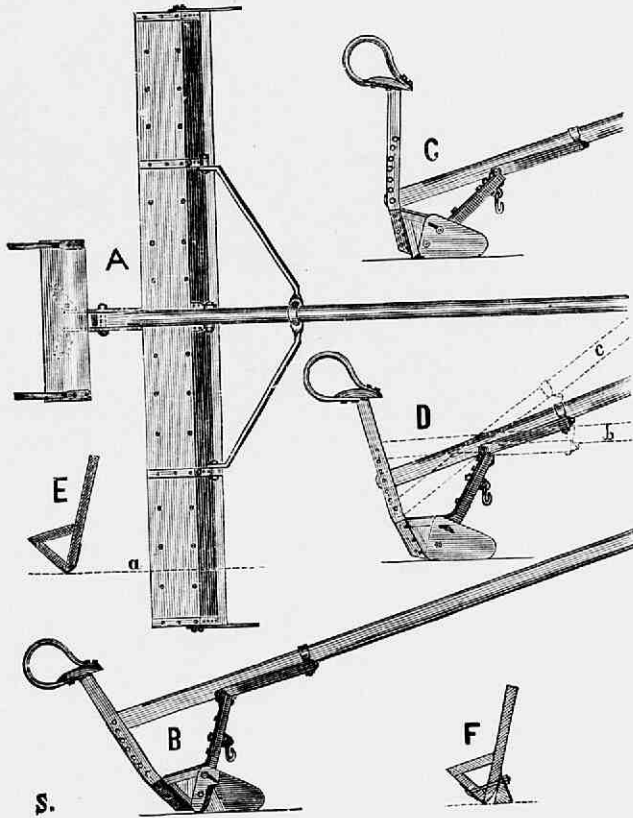
Fig. 167. Sack's akkersleep: A, van boven gezien; B, C, D, van ter zijde gezien; aan deze figuren ziet men dat de disselboom verplaatsbaar en daardoor de drukking meer of minder groot gemaakt kan worden; E, doorsnede volgens a ; F, dezelfde doorsnede, maar hier nog van eene lijst voorzien om op zeer oneffen terrein of op wegen den grond vlak te maken.
