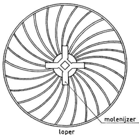
Molensteen. Het maalvlak van de loper. Het molenijzer dient voor de bevestiging van de molensteen aan de aandrijf-as.
