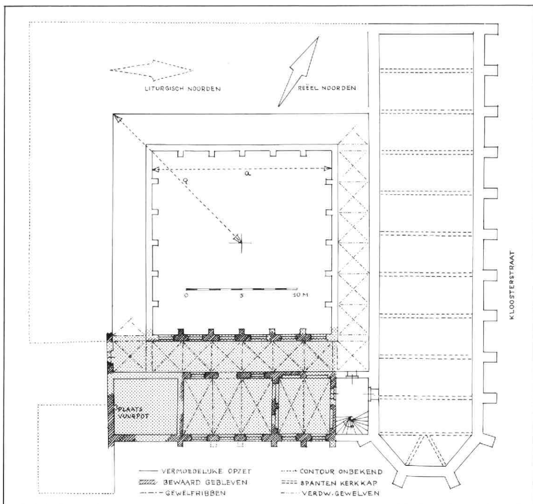
Afb. 7. Reconstructie plattegrond. Opzet van de kerk, afgeleid uit het bewaard gebleven bestek van de herstelling na de brand van 18 mei 1537. Het bewaard gebleven deel van de kloostergang laat zien, dat deze voldeed aan de al in de 13 e eeuw vastgelegde regel: halve diagonaal van de gang = binnenmaat pandhof – Villard de Honnecourt, zie publikatie Hahnloser, Wenen 1935, p. 107, 39 K. Het betreft hier een iets later toegevoegde tekening – (tek. G. Berends/C.L. Temminck Groll).
