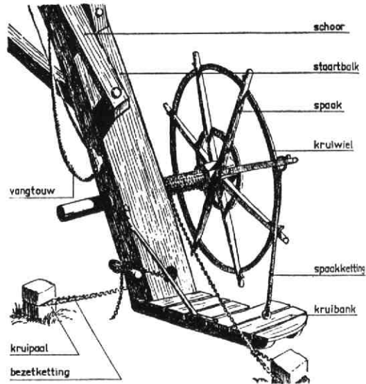
Het kruirad of kruiwiel.
