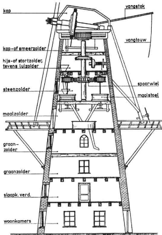
Doorsnede van een stellingmolen.
