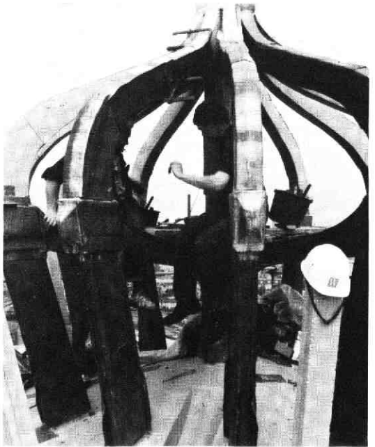
Het opnieuw aanbrengen van de loodbekleding om het beton van de keizerskroon.
