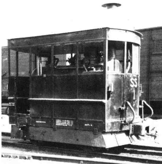
De Merryweather locomotief SS1 welke gebouwd en in dienst is gesteld in 1878 voor de dienst op de tramlijn Den Haag-Scheveningen.
