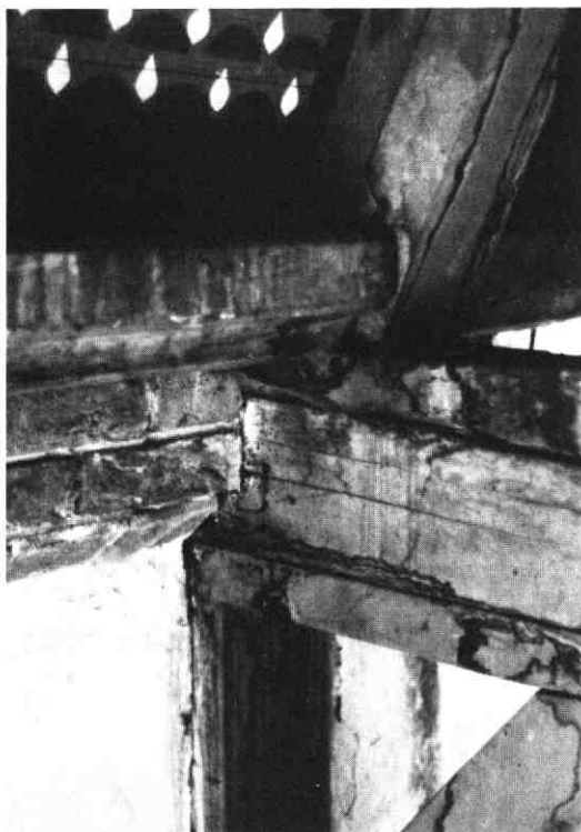
Een, door inwateren sterk aangetaste, houten dakvoetconstructie in het koor voor de restauratie.
