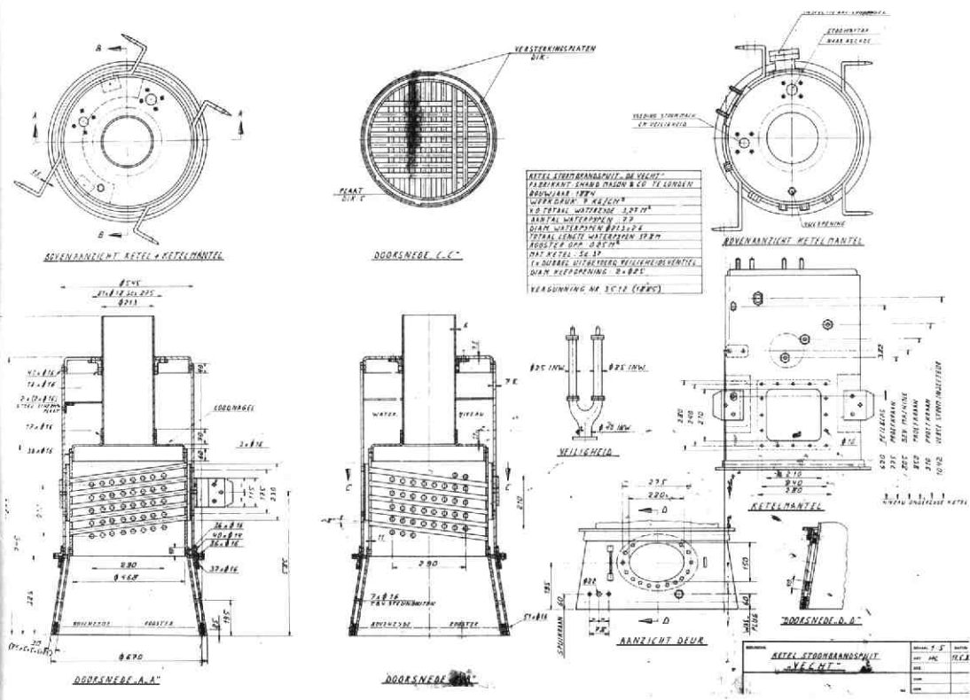
De door de werkgroep gemaakte tekening van de ketel.
