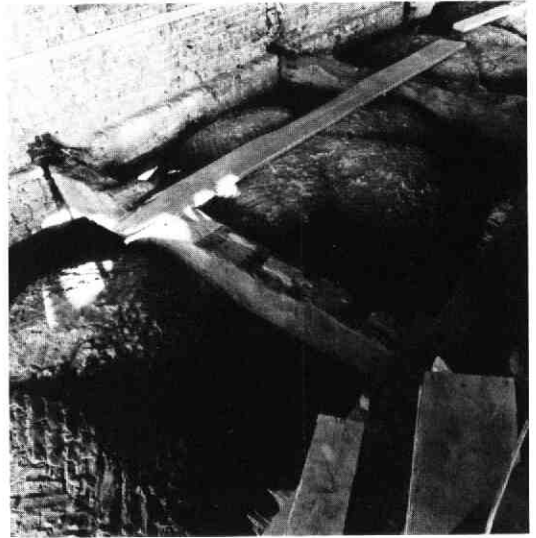
Afb. 15. Moerbinten boven de gewelven van de kloostergang, met inkepingen voor de kinderbinten. (foto Paul van Vliet, 1984).
