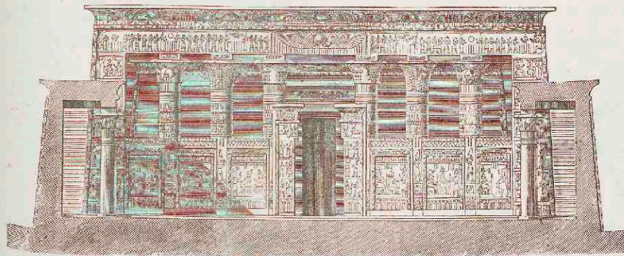
3. Tempel te Edfoe; dwarsdoorsnede.
