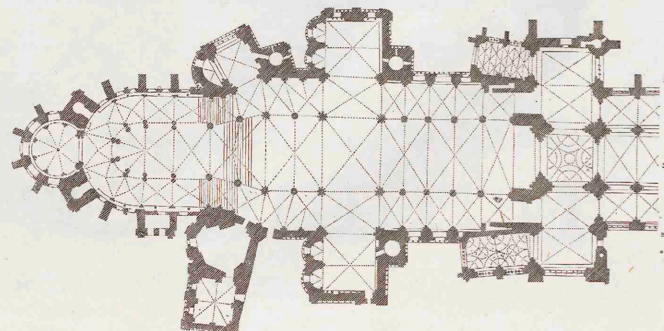
8. Kathedraal te Canterbury. Oostzijde. 1174—1185.
