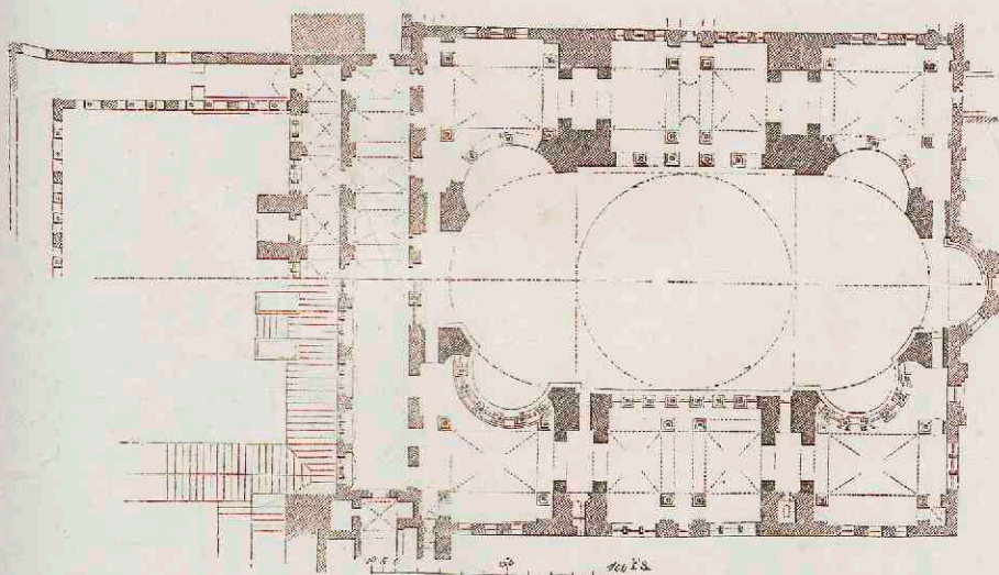
2. Plattegrond der Sofiakerk.
