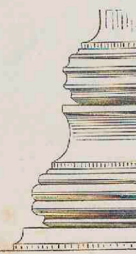
18. Zuilvoet. Van de oostelijke hal van het Erechtheion.
