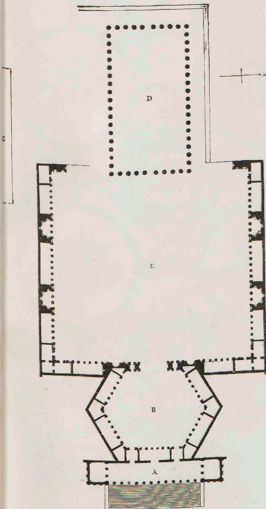
1. Tempel te Heliopolis. (Baalbek.) A. Voorgaanderij. B. Eerste voorhof. C. Tweede voorhof. D. Tempel van Baal-Helios. E. Tweede tempel.
