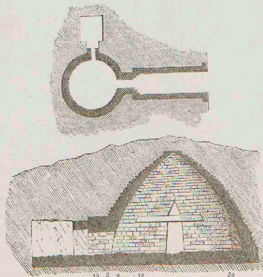
4. Schatkamer te Mukene.
