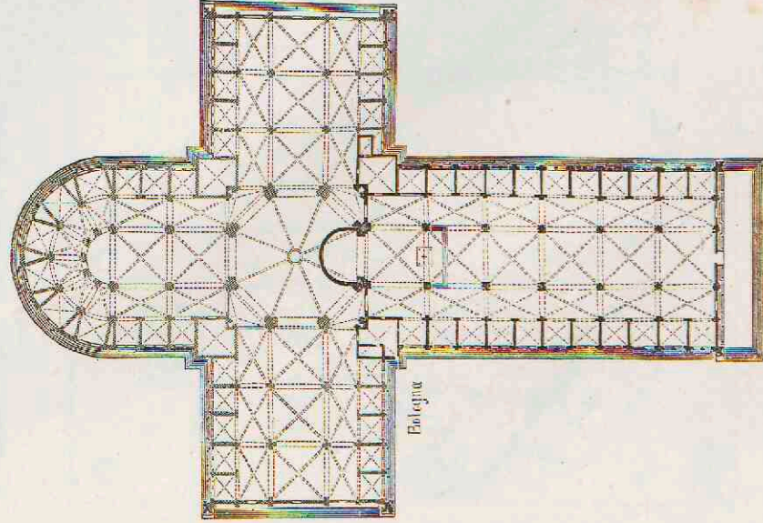
9. S. Petronio te Bologna. Begonnen 1390.
