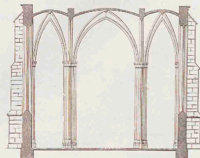
7. Dwarsdoorsnede van een schip.
