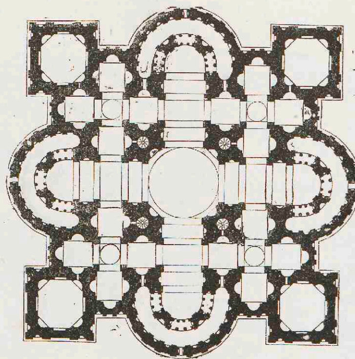
2. Peruzzi's ontwerp voor den S. Pieter.
