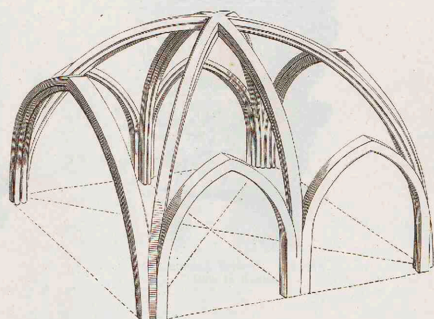
4. Constructie van een zeshoofdig gewelf.
