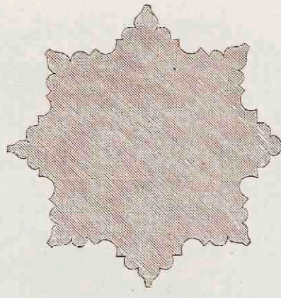
8. Plattegrond van een pijler der Jacobikerk te Rostock. Baksteenbouw.
