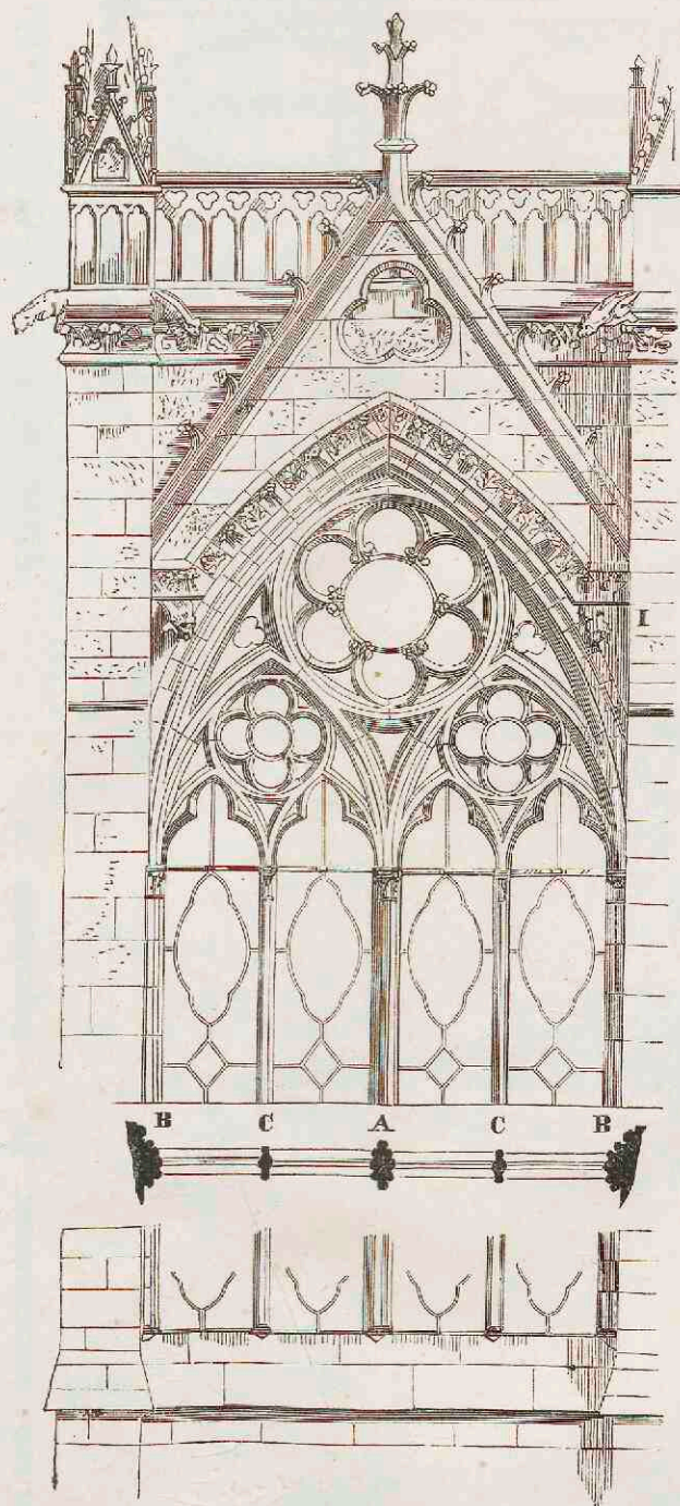
1. Venster met puntgevel (windberg). Sainte chapelle te Parijs.
