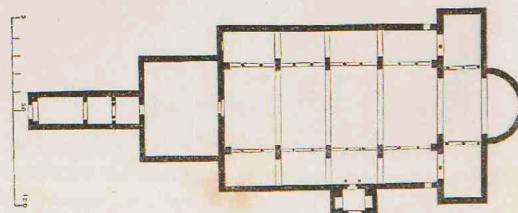
6. S. Prassede te Rome. 9 e eeuw.
