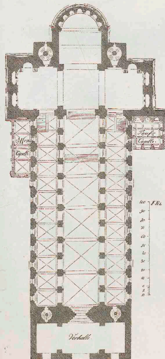
3. Dom te Spiers. (Zie pl. 54, fig. 6.)
