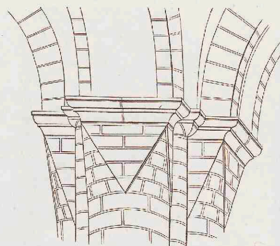
3. Kapiteel te Ratzeburg.
