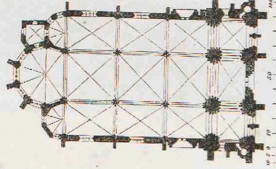
10. Dom te Minden. Het schip uit de helft der 13 e eeuw.
