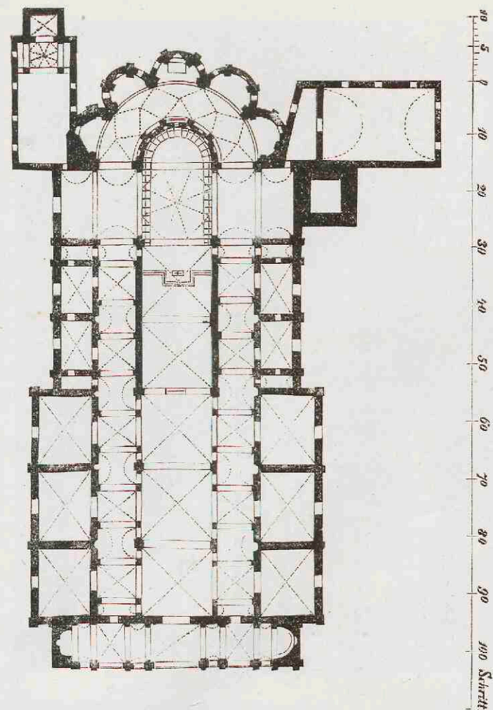
1. Kerk in S. Benedetto, gebouwd door Giulio Romano.
