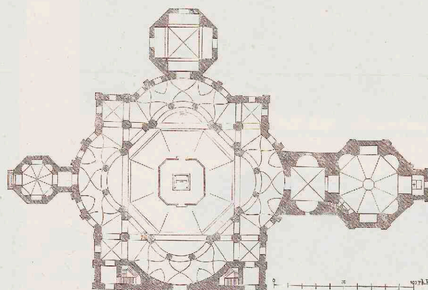
3. S. Lorenzo te Milaan. 4e — 5e eeuw.
