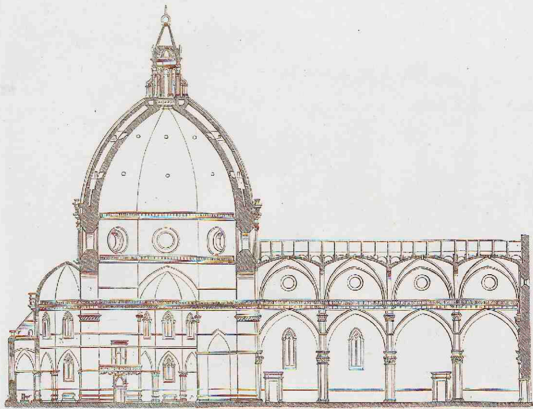
1. Dom te Florence. Lengtedoorsnede. Begonnen 1294 door Arnolfo di Cambio.
