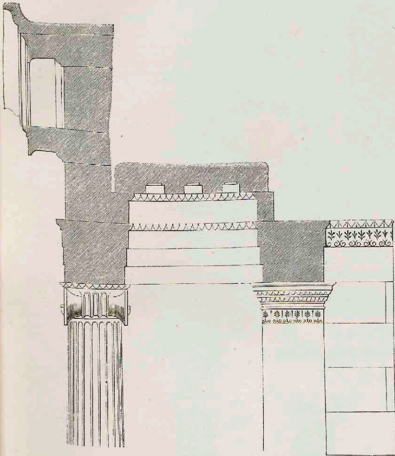
2. Voorgaanderij (prostasis) van den tempel der Nike. Doorsnede.
