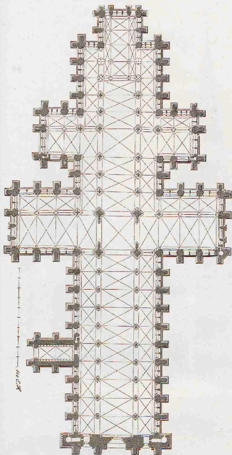
1. Kathedraal te Salisbury. 1220—1258. (Vergel. fig. 10.)
