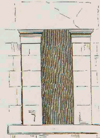
14. Venster van de propulaïen te Athene.
