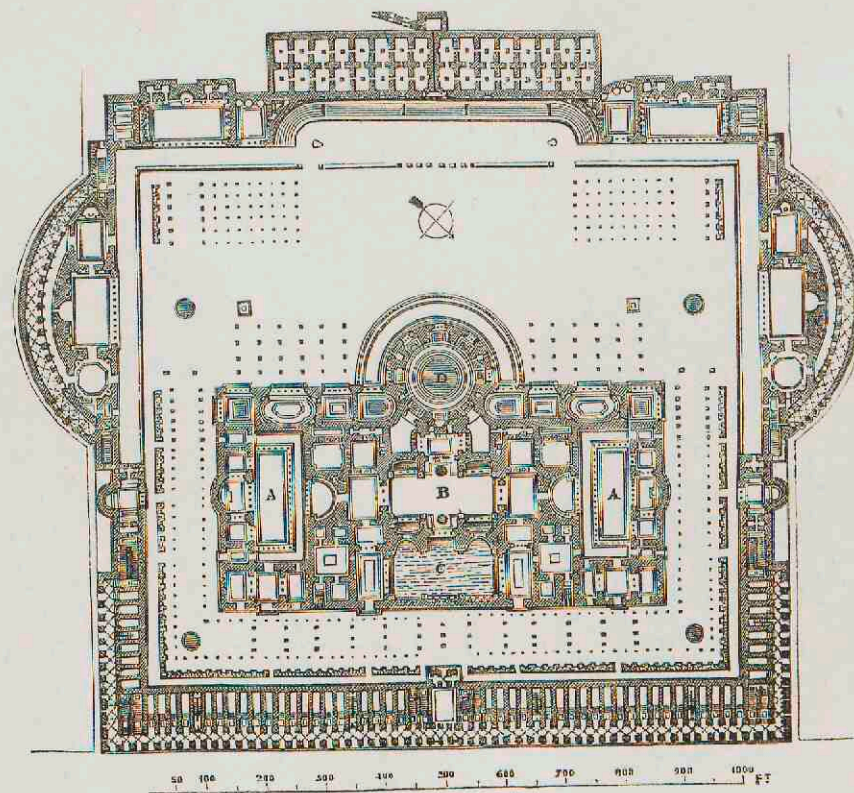
5. Plattegrond der thermen van Caracalla.
