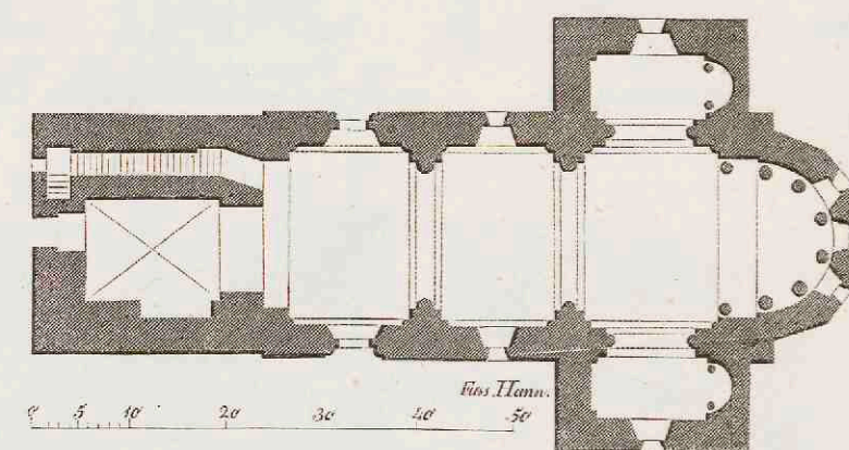
6. Kerk te Idensen.
