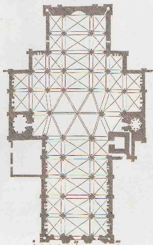
6. Dom te Sienna.
