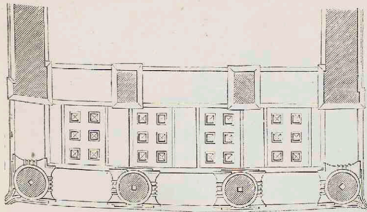
1. Tempel der Nike apteros (ongevlengelde overwinning) te Athene. Plattegrond der voorhal.
