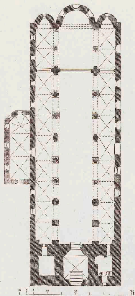
2. Dom te Seccau. Gebouwd na 1145.
