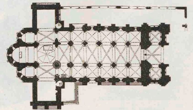
7. S. Vincente te Avila. Na 1150.
