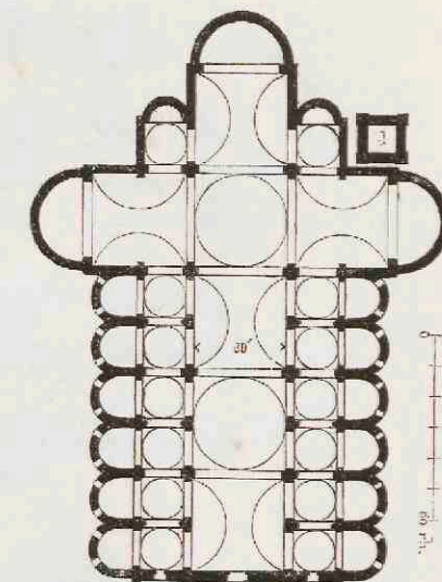
8. S. Benedetto te Ferrara.
