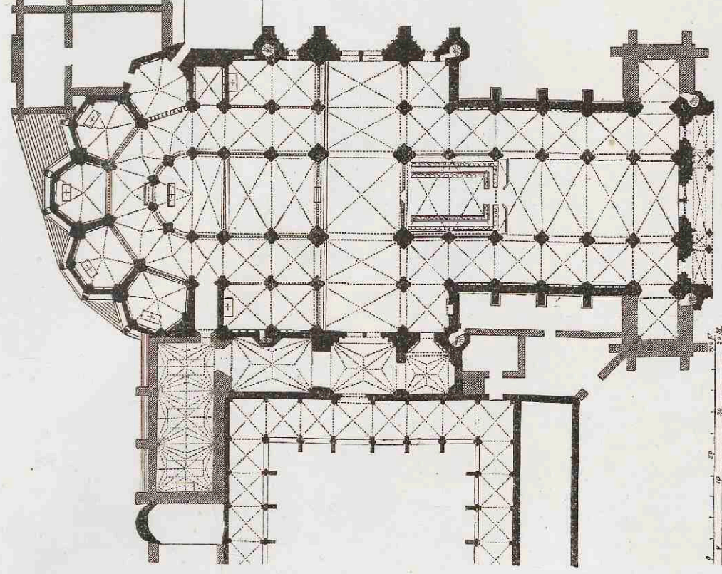
2. Kathedraal te Leon. Gebouwd sedert 1250.
