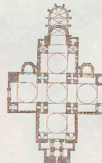
7. S. Front te Périgueux. Fig. 6.
