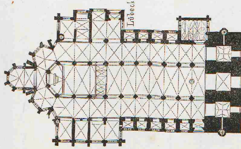
6. Mariakerk te Lübeck. Gesticht 1276.
