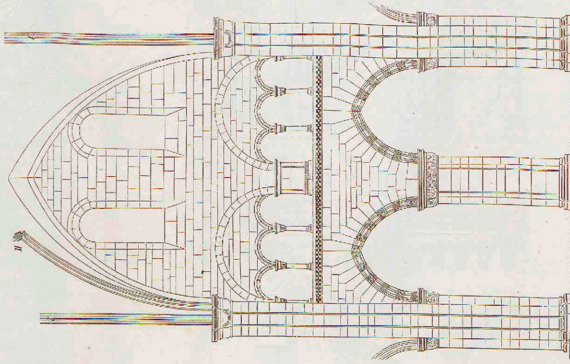
1. Kathedraal te Bazel. Onstr. 1200.
