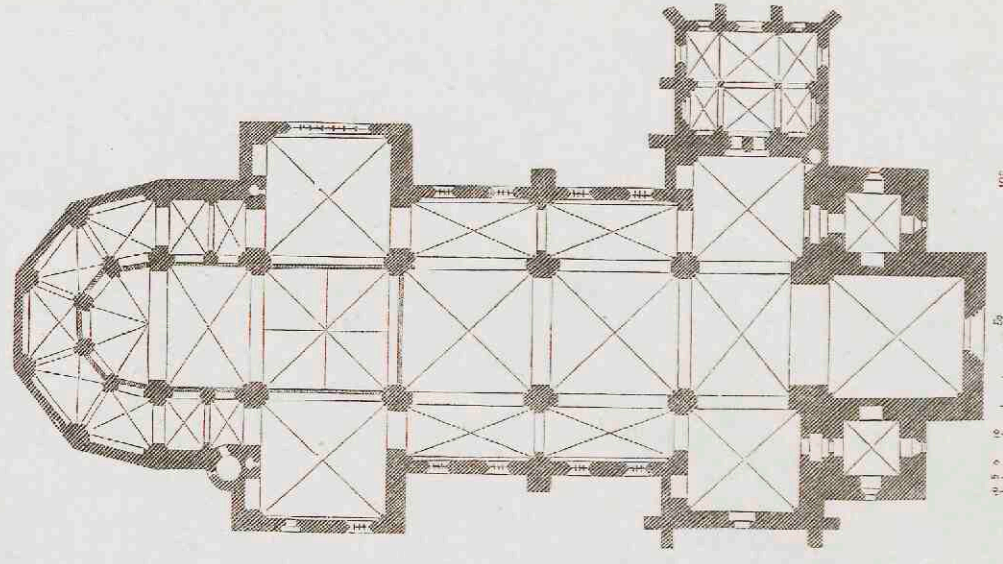
11. Dom te Münster. 1225—1261.
