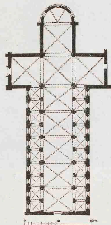
6. Plattegrond der kerk van Dobrilugk.
