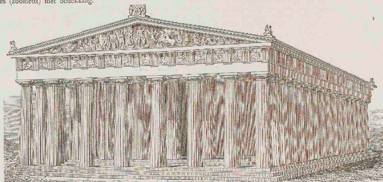
4. Het parthenon te Athene, gewijd aan Athena; voltooid 438 v. Chr. onder Perikles; gebouwd door Iktinos en Kallikrates.
