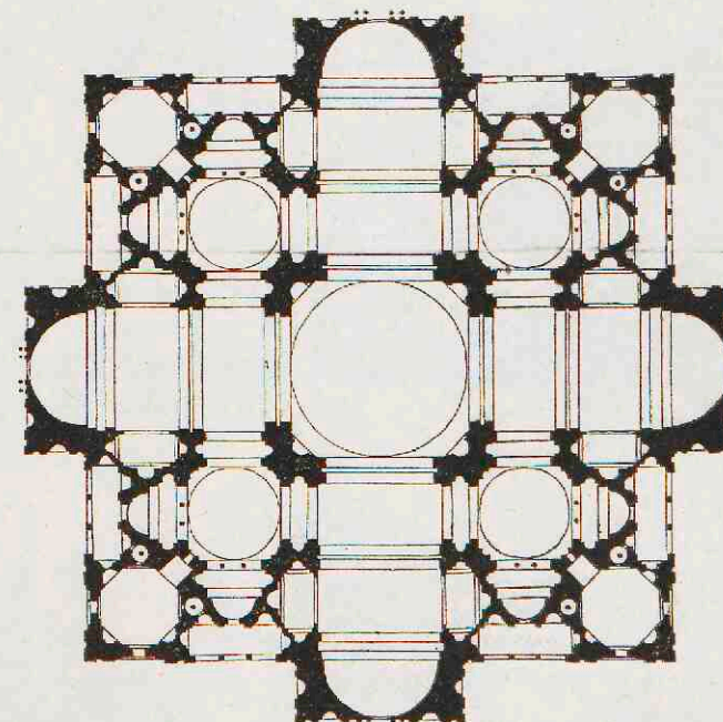
4. Bramante's ontwerp voor den S. Pieter.
