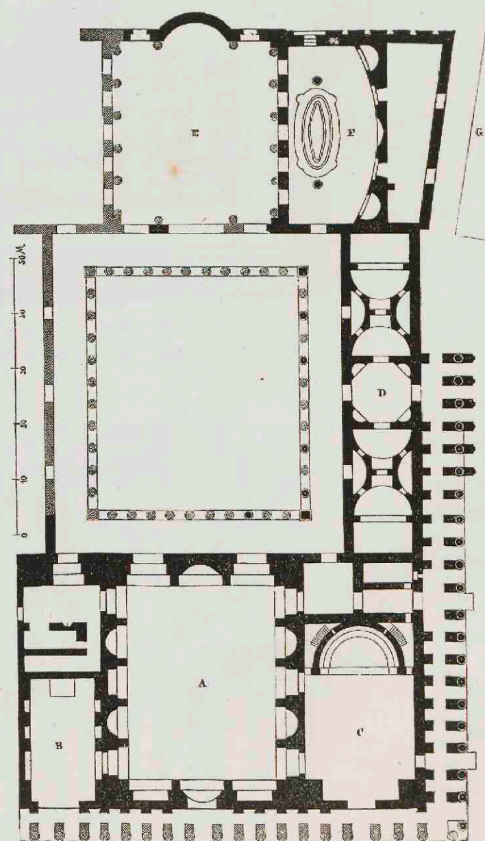
6. Plattegrond van het paleis der Flavii. A. Tablinum. B. Lararium. C. Basilica. D. Atrium. E. Eetzaal (occur). F. Nymphaeum. G. Tempel van Jupiter victor.
