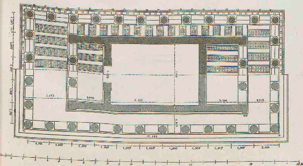
7. Zoldering van den Nemesionstempel te Rhamnos. (Vergel. plaat 1, fig. 2.)
