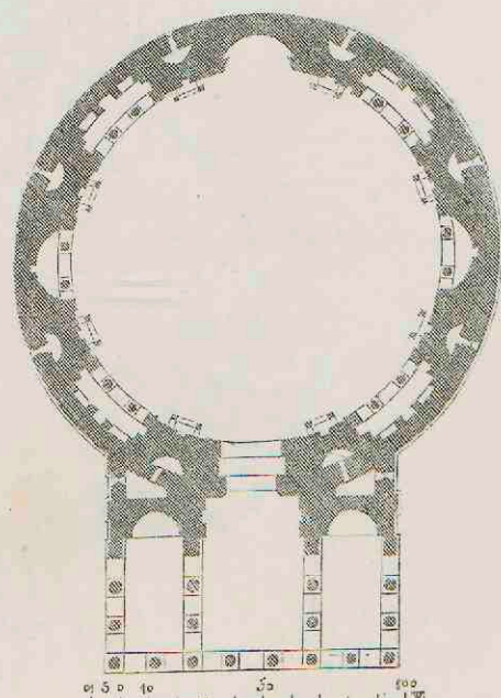
12. Plattegrond van het pantheon.
