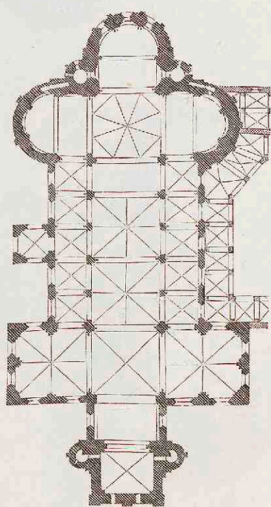
4. Apostelkerk te Keulen. (Zie pl. 54, fig. 1.)
