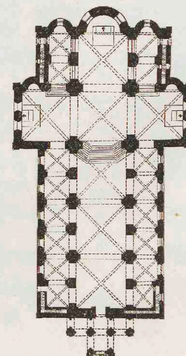
5. Kerk te Ellwangen.
