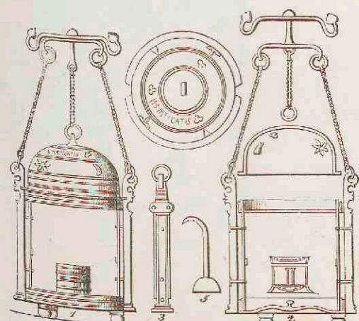
6. Bronzen lantarens, en doorsnede. Pompei.
