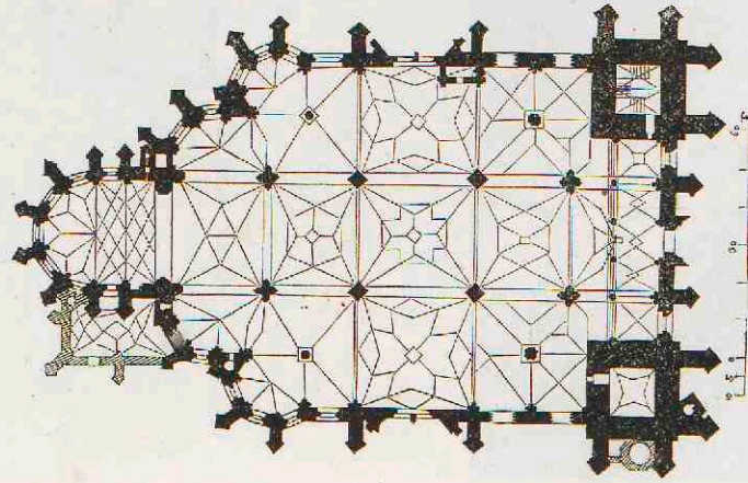
9. Dom te Kaschau. 14 e eeuw.
