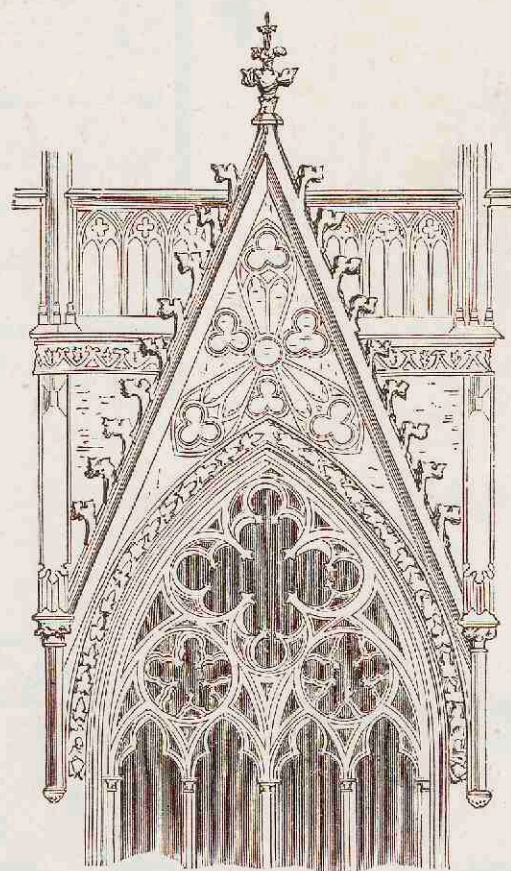
2. Puntgevel (frontaal of windberg) van den dom te Keulen.
