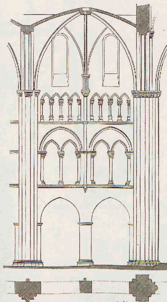
7. Travée in den dom van S. Joris te Limburg. (Overgangsstijl.)
