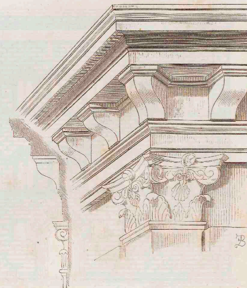
12. Kroonlijst van de cancellaria te Rome.
