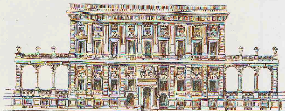
8. Paleis Tursi Doria te Genua. Gevel. Door Rocco Lurago. Einde der 16e eeuw.
