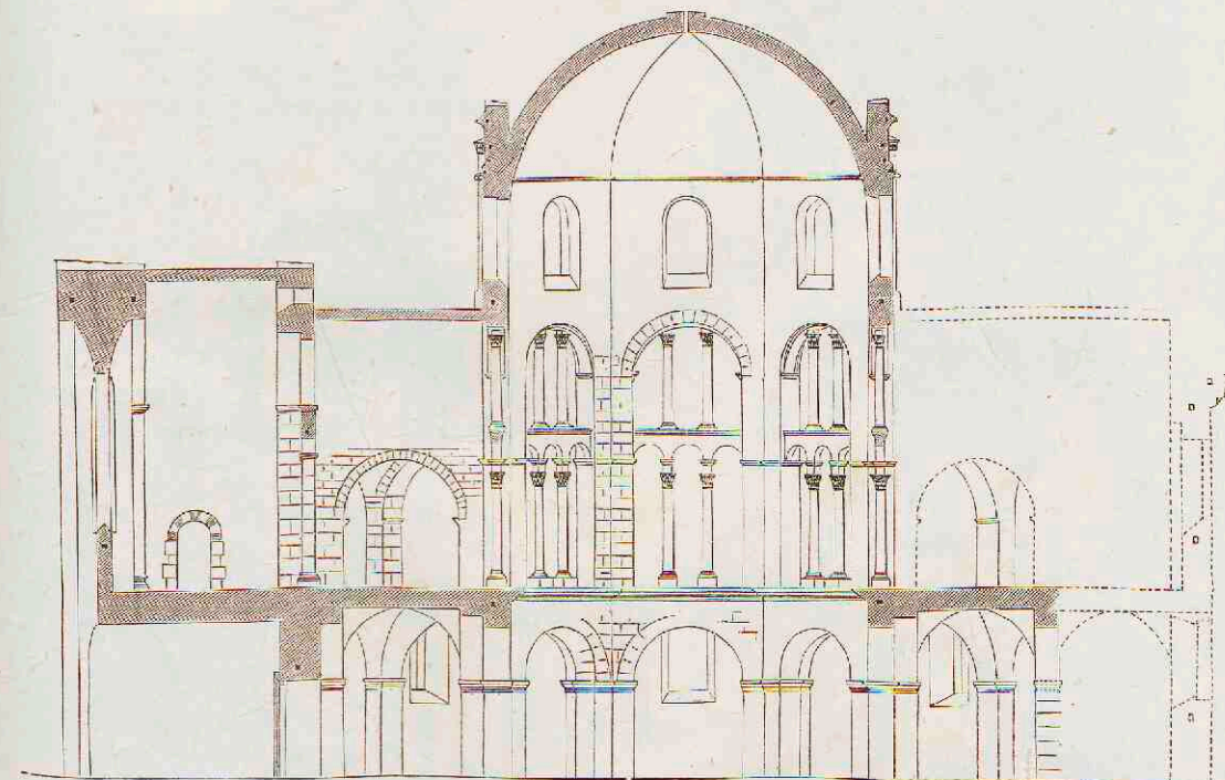
2. Paleiskapel van Karel den Grooten te Aken. Omstr. 800. Doorsnede van den bovenbouw en de krocht.
