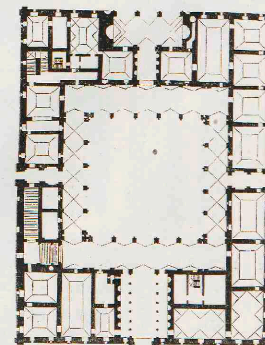
10. Paleis Farnese te Rome. (Vergel. pl. 97, fig. 1 en pl. 100, fig. 4.)
