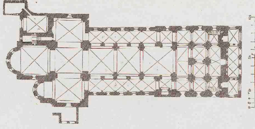
7. Dom te Soest. Omstr. 1200.
