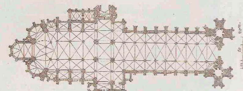
7. S. Ouen te Rouaan. 14 e eeuw.
