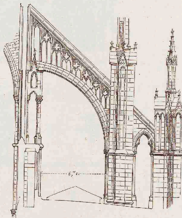
11. Schraagpijlers en bogen van het koor der kathedraal te Amiens.
