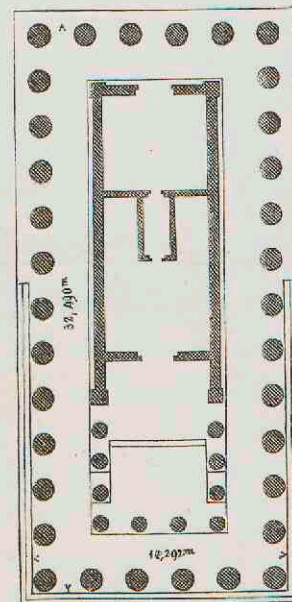
2. Demetertempel te Paestum.
