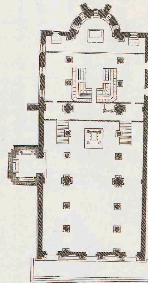
3. S. Miniato bij Florence.
