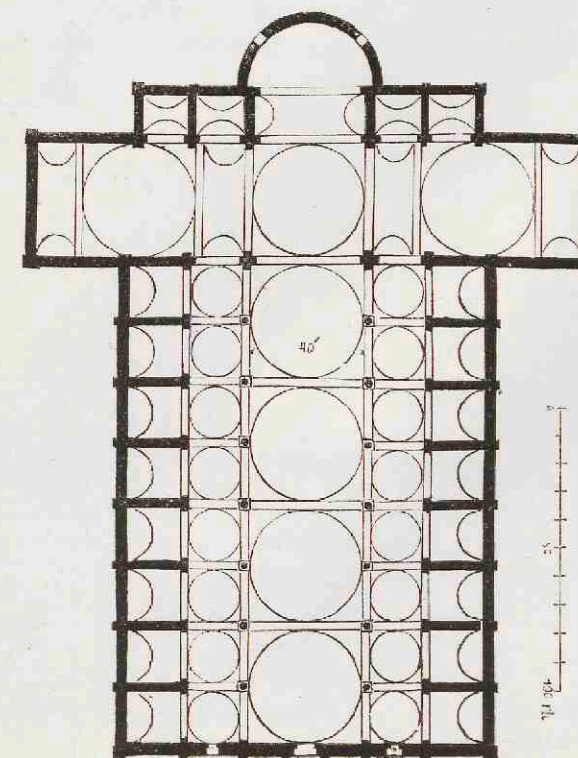
12. S. Francesco te Ferrara. (Vergel. pl. 99, fig. 7.)
