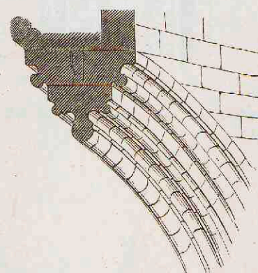
16. Kathedraal te Nevers, 1230—1250.
