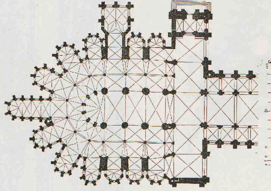
3. Kathedraal te Le Mans. Koor aangebouwd in 1217.
