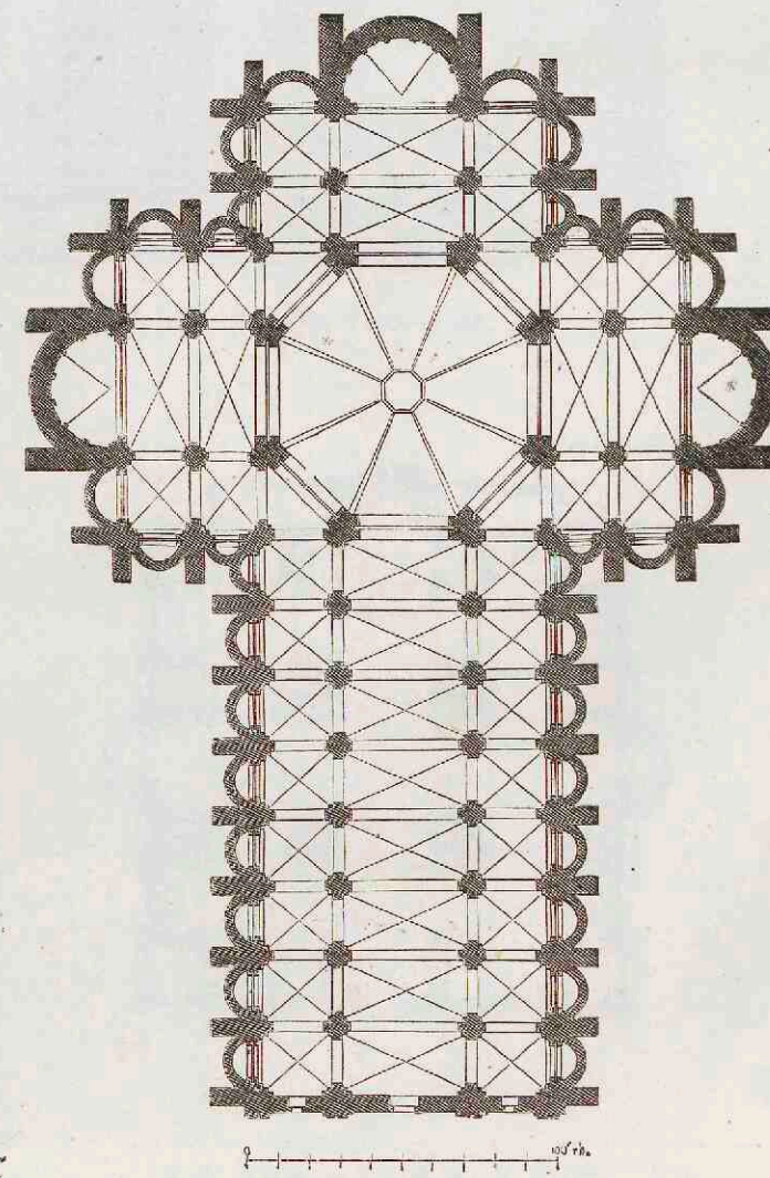
5. Dom te Pavia. Plattegrond. Ontwerp van Bramante omstreeks 1490.
