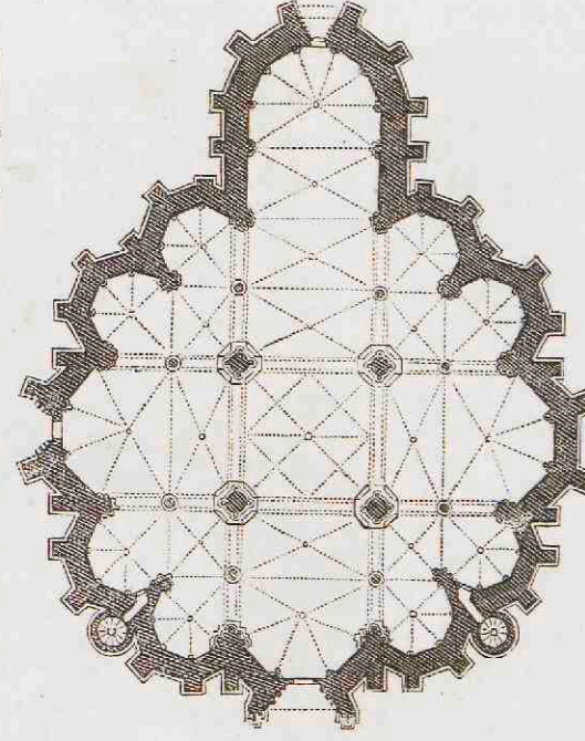
11. Kapittelkerk te Xanten. Koor 1263 begonnen.
