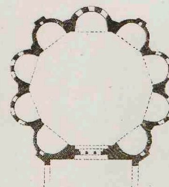
3. Zoogenaamde tempel van Minerva medica te Rome.
