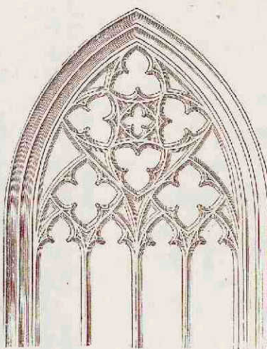
5. Wiesenkerk te Soest. Omstreeks 1350.
