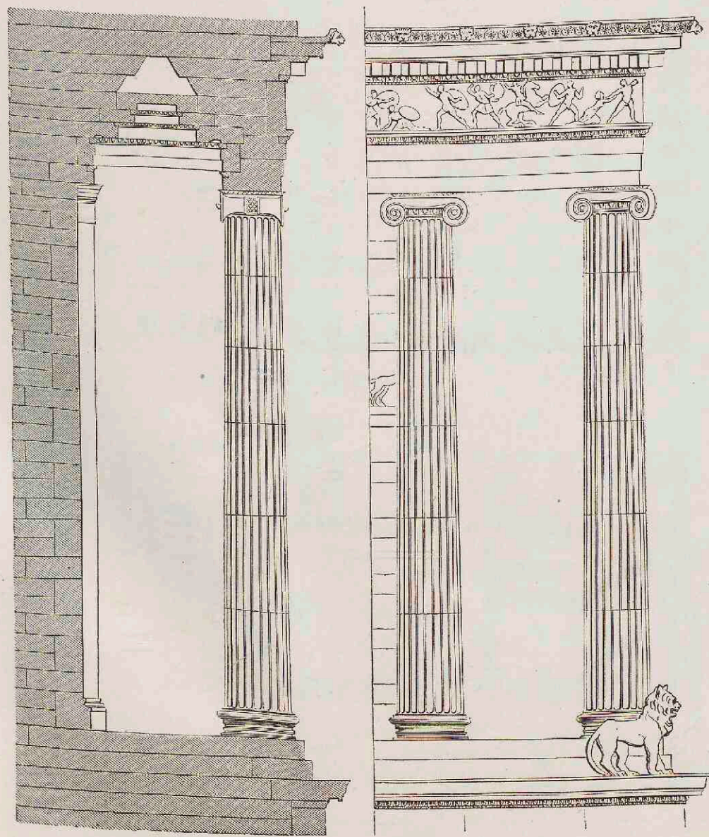
2. Zuilengang van het Mausoleion; doorsnede en opstand.
