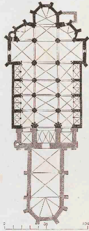
6. Katharinker te Oppenheim. 1262—1317.
