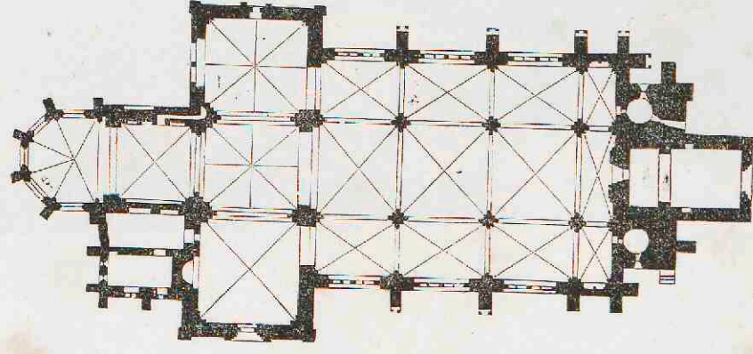
7. Kloosterkerk te Dargun. 14 e en 15 e eeuw.
