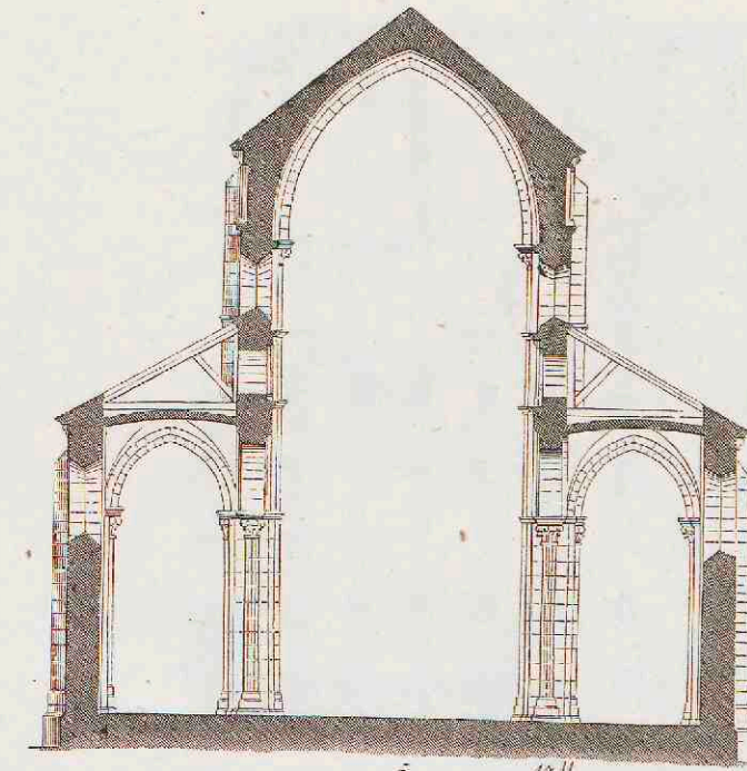
8. Dom te Autun. Dwarsdoorsnede. Begonnen 1132.
