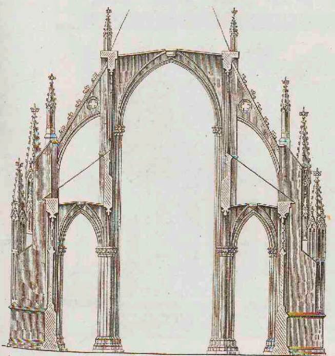
2. Dwarsdoorsnede van den dom te Halberstadt.
