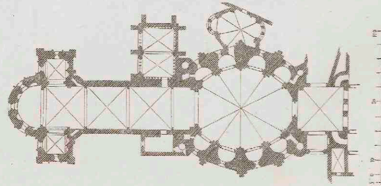
8. S. Gereon te Keulen. De tienzijdige koepelbouw der westzijde is van 1212—1227 in den overgangsstijl aan de romaansche basilica bijgebouwd.
