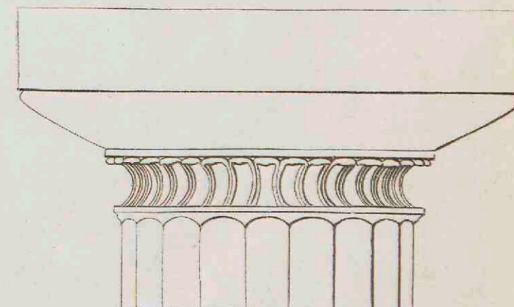
11. Tempel van Demeter te Paestum.
