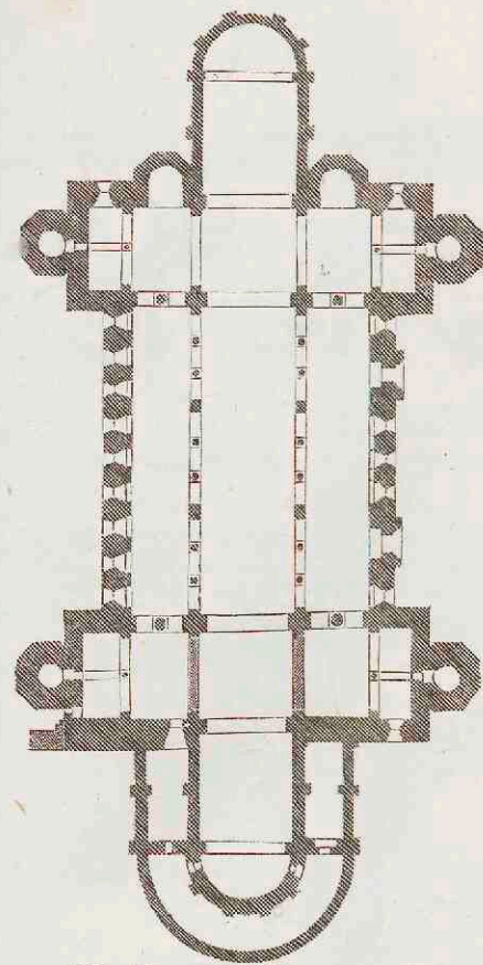
1. S. Michiel te Hildesheim. Gesticht 1001; nieuwere bouw van 1184.
