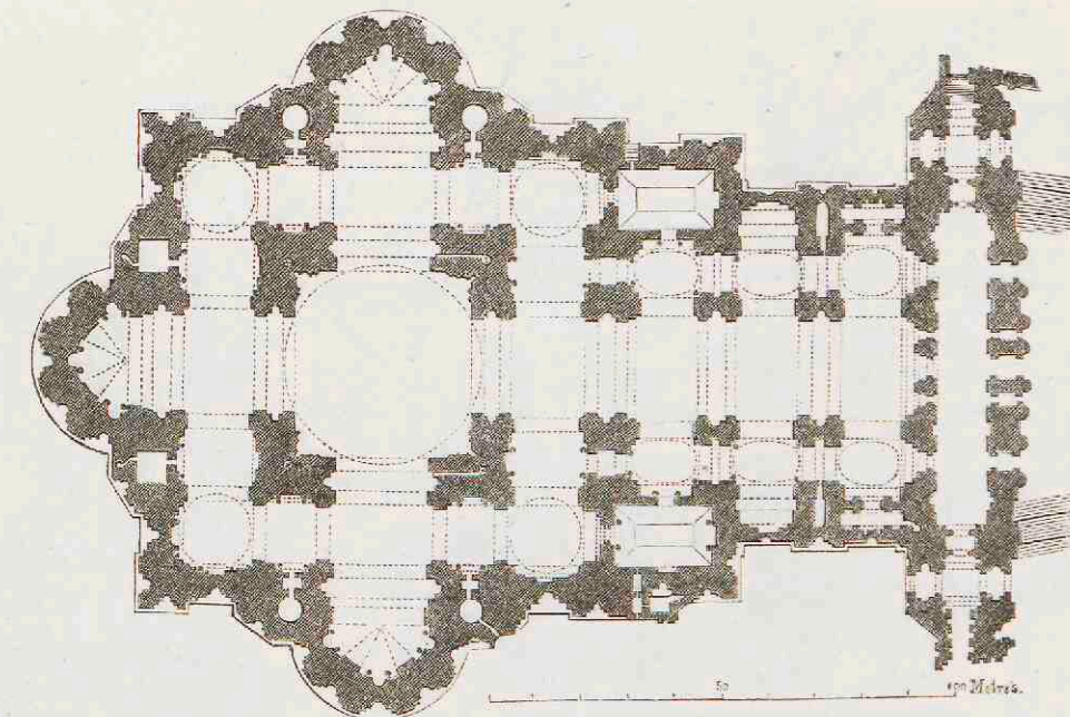
3. Tegenwoordige staat van den S. Pieter te Rome.
