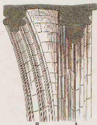
17. Sainte chapelle te Parijs, 1243—1251. A Diagonaalrib of graadboog. B Gordelrib.
