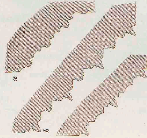
3. Portaalprofielen van kerken te Rostock. Baksteenbouw.
