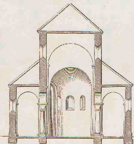
5. Dwarsdoorsnede eener romaansche basilica.
