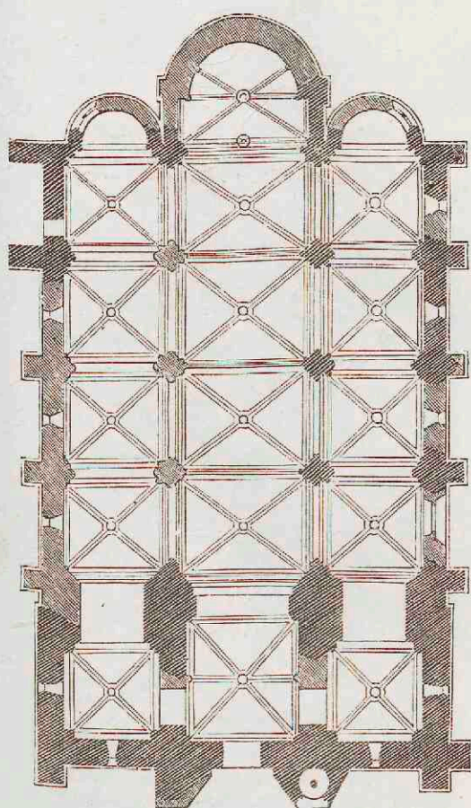
5. Kerk te Zsambek in Hongarije. Overgangsstijl.
