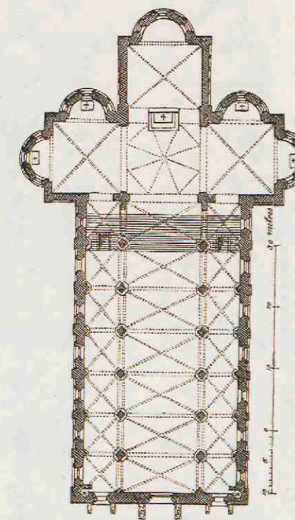
4. Dom te Parma.
