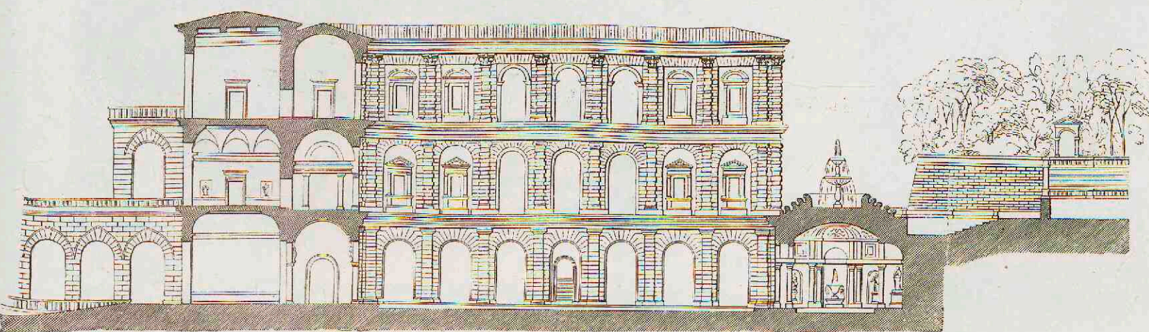
7. Paleis Pitti te Florence. Doorsnede. Geb. door Brunellesco. (Vergel. fig. 5.)
