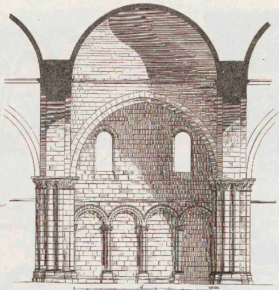
2. Kerk te Fontévrault. Deel der lengtedoorsnede. (Vergel. pl. 64, fig. 10.)
