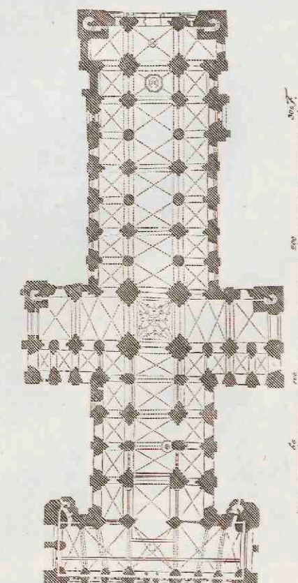
12. Kathedraal te Durham.
