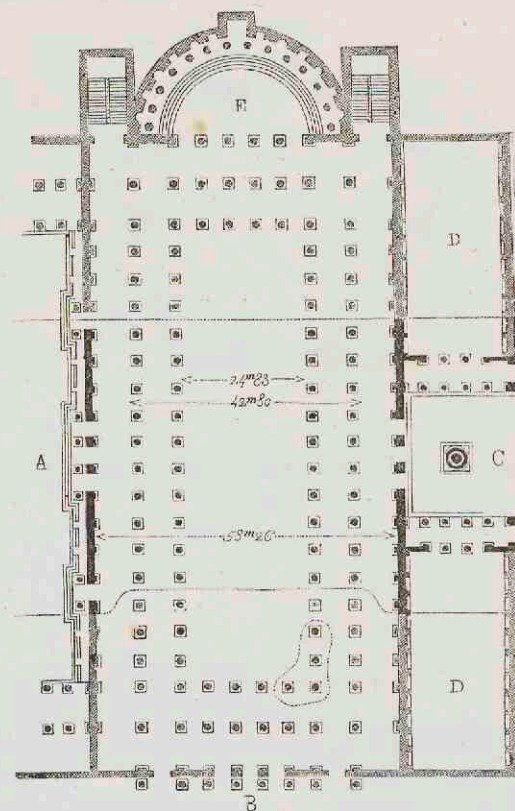
10. Basilica Ulpia op het forum van Trajanus te Rome.
