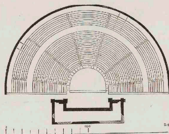
5. Schouwburg te Segesta, plattegrond.
