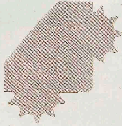
4. Plattegrond van eenen pijler der kloosterkerk te Dobran. Baksteenbouw.
