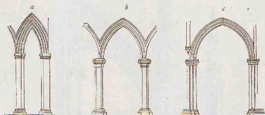
3. Spitsboogvormen. a Lancetvorm. b Gelijkzijdige boog. c Gedrukte boog.
