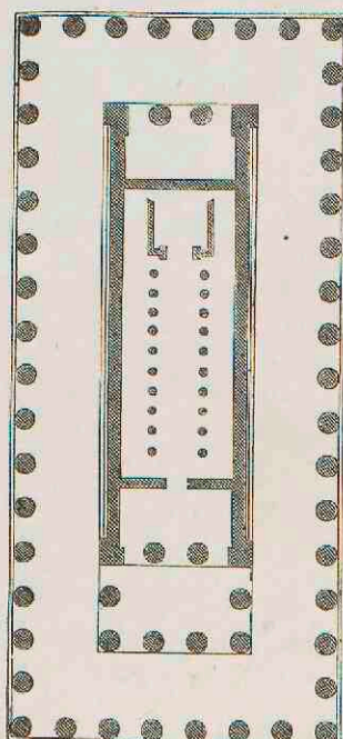
4. Zeustempel te Selinunte.
