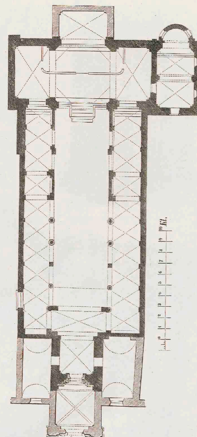
4. S. Pieter te Salzburg. Na 1127.
