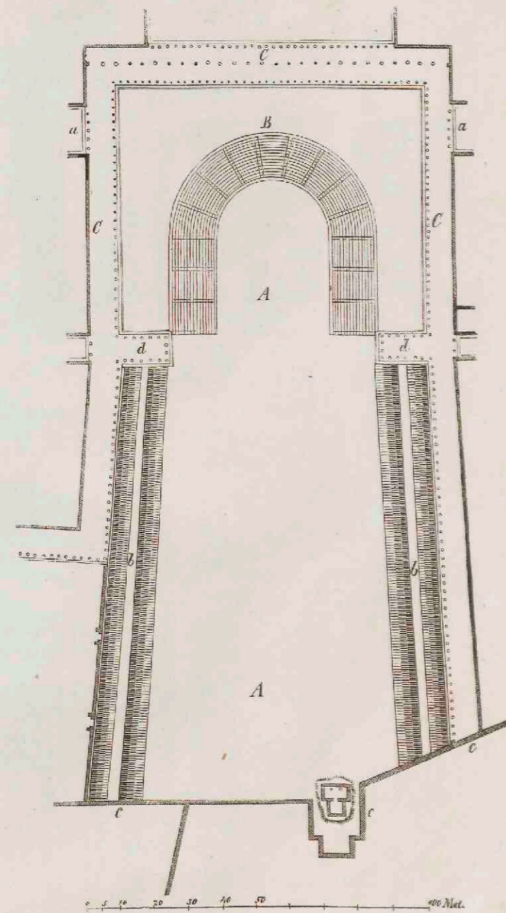
8. Stadion (renperk) te Messene.
