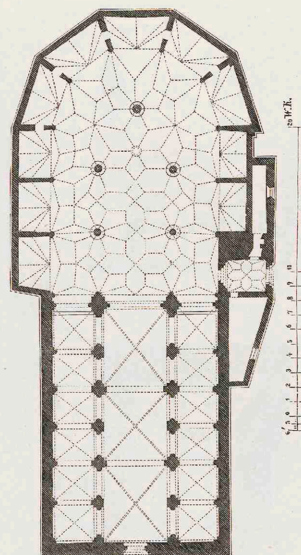
3. Franciskanenkerk te Salzburg. Overgangsstijl. 13 e eeuw.
