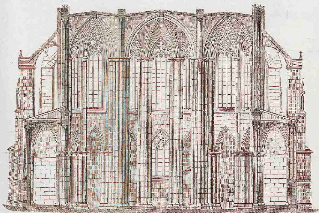
9. Koor der kerk te Zwettl. Dwarsdoorsnede. 1343—1383.
