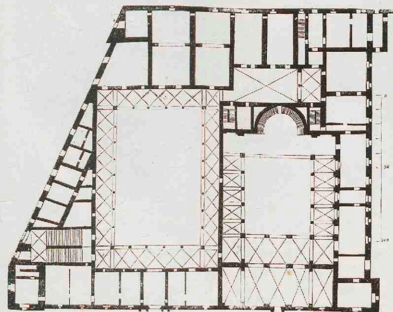
9. Paleis der Cancellaria met de kerk S. Lorenzo in Damaso. Gebouwd door Bramante. (Vergel. pl. 97, fig. 11.)
