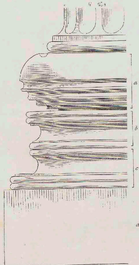
16. Van den tempel van Athene te Priëne. a. toros. b. c. trochilos. d. plinthos.
