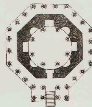
2. Plattegrond des zoogenaamden Jupitertempels te Spalato.
