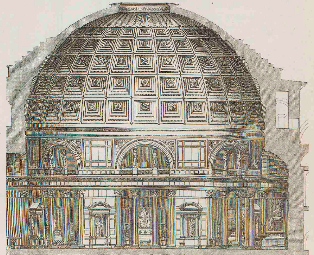
14. Doorsnede van het pantheon. Oorspronkelijke aanzicht volgens Adler.
