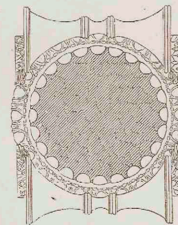
4. Horizontale doorsnede van een ionisch zuilhoofd.
