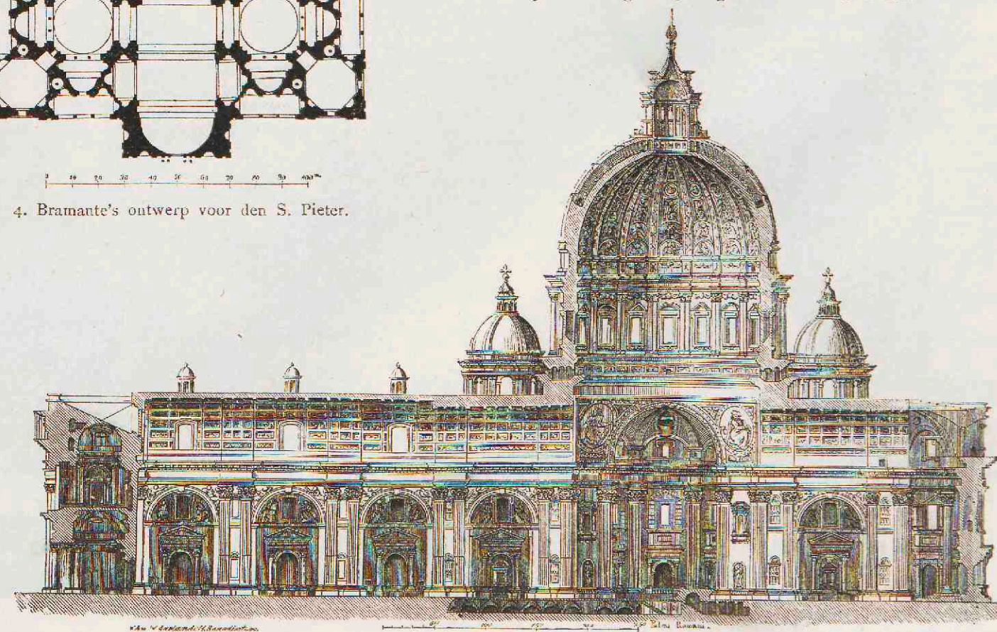
6. S. Pieterskerk te Rome, doorsnede.
