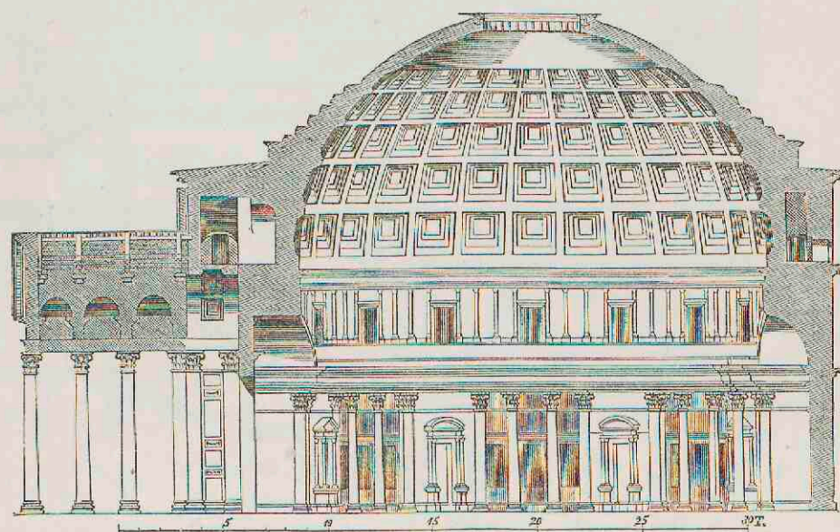
13. Het pantheon te Rome. Doorsnede. Gebouwd 26 v. Chr. hersteld 202 na Chr.
