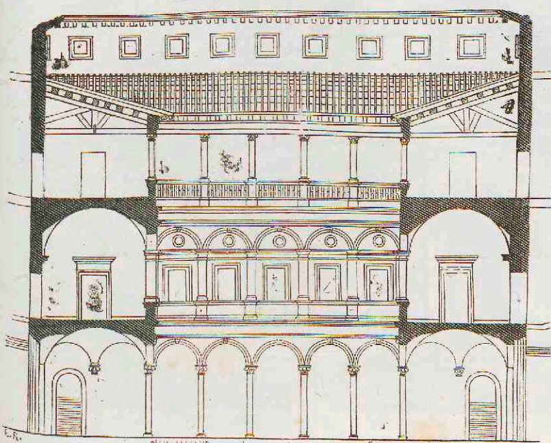
4. Palazzo Strozzi te Florence. Doorsnede van den hof. (Vergel. fig. 6.)
