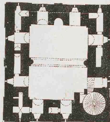
17. Burg Hedingham. 2 e verdieping. (Zie pl. 61, fig. 6 en 7.)
