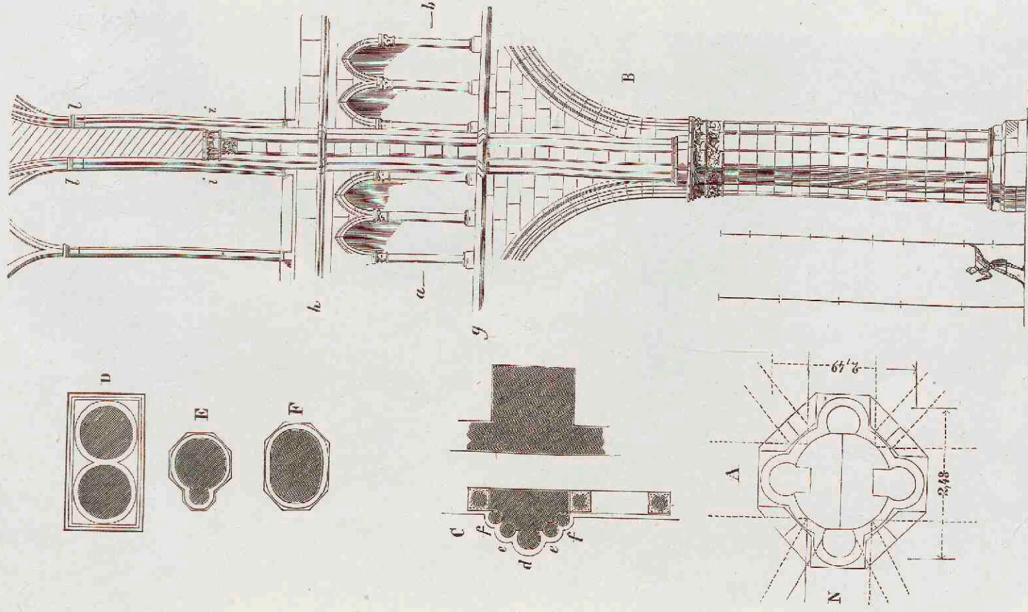
1. Schip der kathedraal te Rheims. A Ronde zuil met vier diensten. B Opstand van den pijler. C Plattegrond der diensten of muurzuiltjes. g h Lijsten. ab Nomeningang of kerktrans (inforium). D E F Plattegronden van de oudere pijlers.
