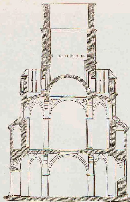
5. Dubbelkerk te Schwarz-Rheindorf. Anno 1151.
