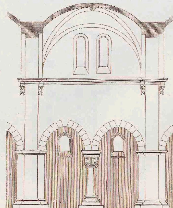
6. Kerk te Rosheim. Travée.
