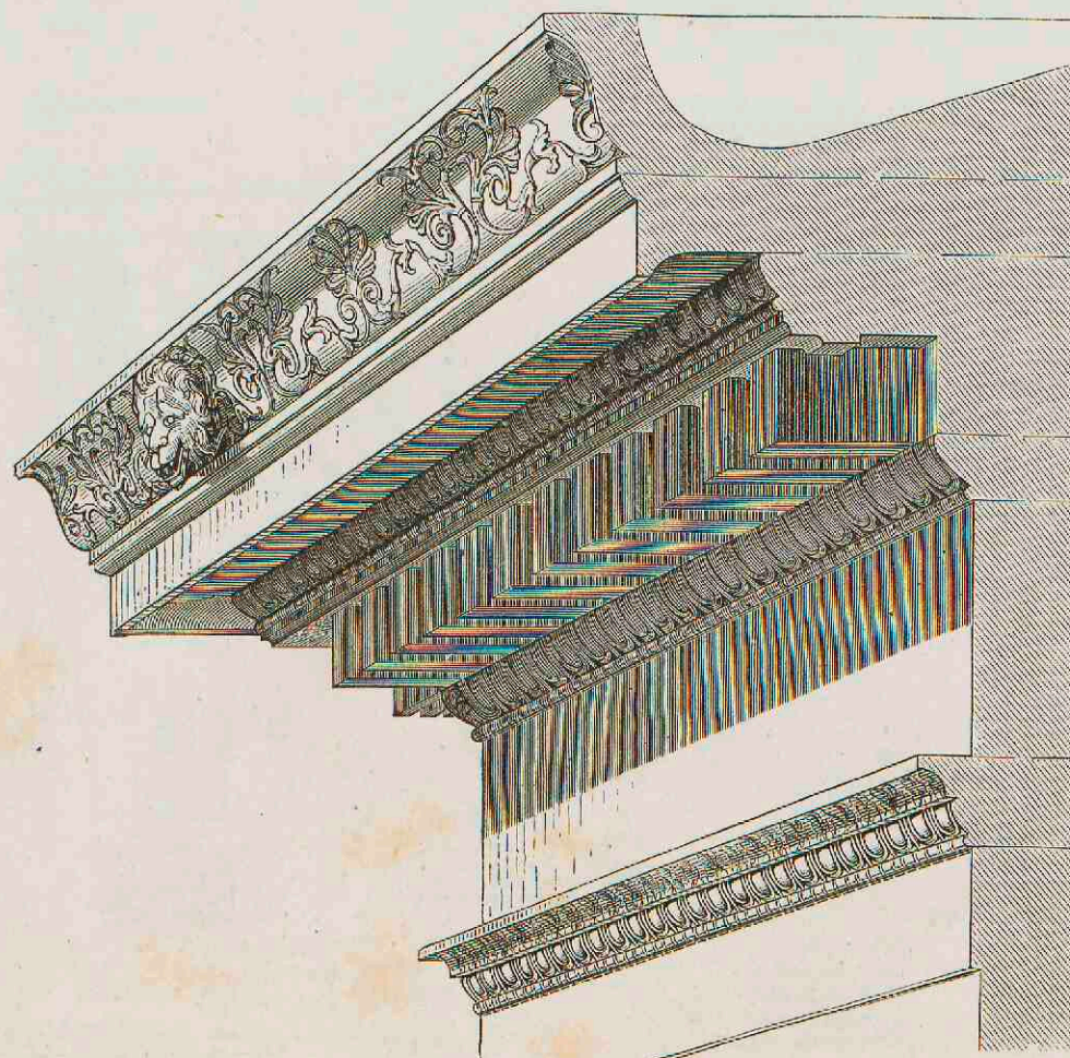
10. Ioniesch hoofdgestel met bladerlijst (kumation) en intandingen. Athenetempel te Priëne. (Vergel. fig. 2.)
