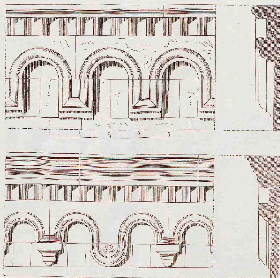
9. Fries der kerk te Schönggrabern.
