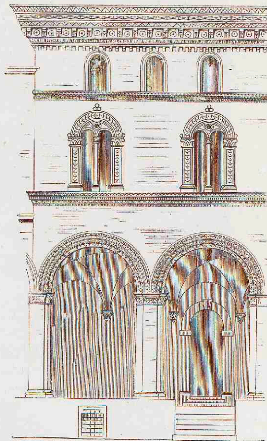
3. Paleis Fava te Bologna.
