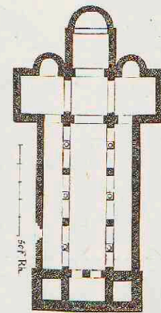
9. Kerk te Hecklingen.
