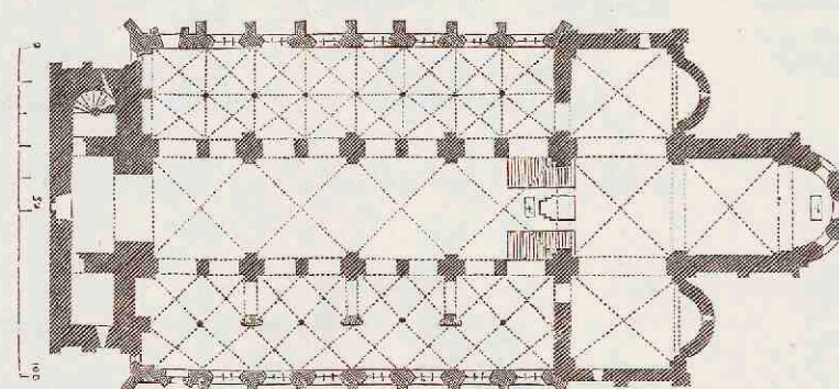
8. Dom te Brunswijk. Anno 1171. De lichter geteekende deelen zijn gothische bijbouwsels.
