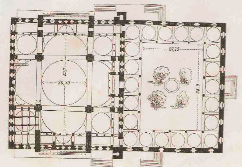
5. Moskee van Mohammed II te Constantinopel. 1463 — 69.
