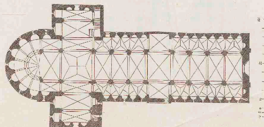
3. Plattegrond der abtdijkerk te Heisterbach.
