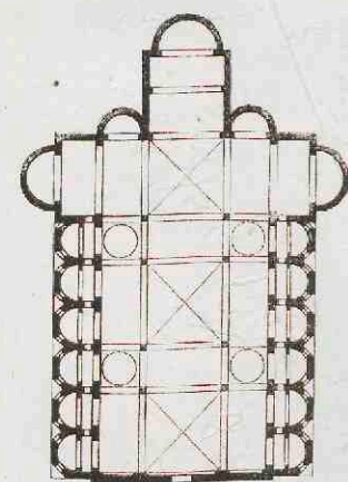
5. S. Sepolcro te Piacenza.
