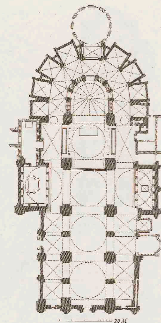
4. S. Antonio te Padua. Begonnen 1231, voltooid in de 14 e eeuw.
