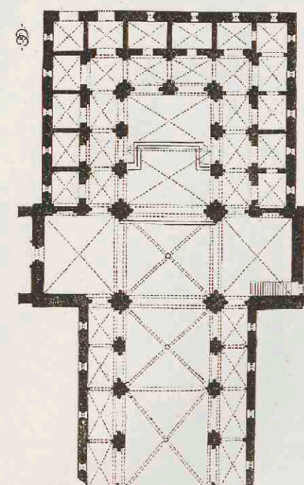
11. Kerk te Riddagshausen. Anno 1275. Cistercenser bouwwerk met rechthoekige koorsluiting.
