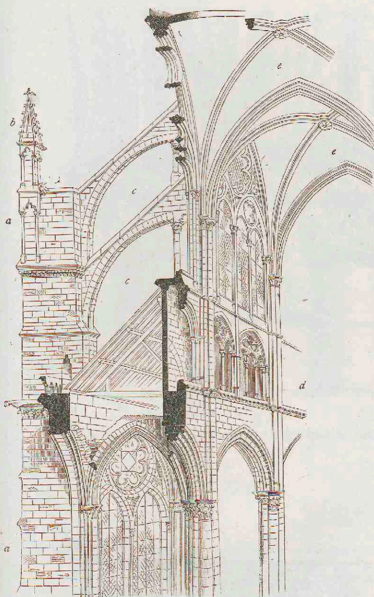
1. Dwarsdoorsnede der kathedraal te Amiens. aa Schraagpijlers. b Fialen. cc Schraagbogen. d Triforium. ee Kruisgewelven. (Vergel. pl. 69, fig. 2.)
