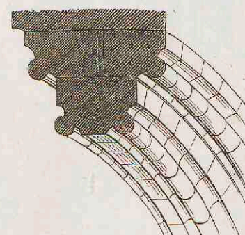
15. Kathedraal te Parijs. 1200—1230.
