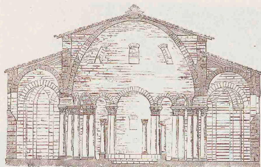
2. S. Maria maggiore bij Nocera. 6e eeuw. Doorsnede.
