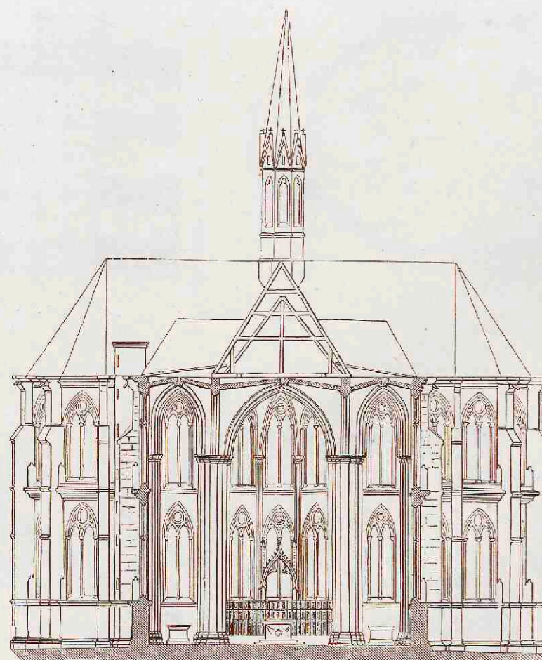
6. Elisabethkerk te Marburg. Dwarsdoorsnede.
