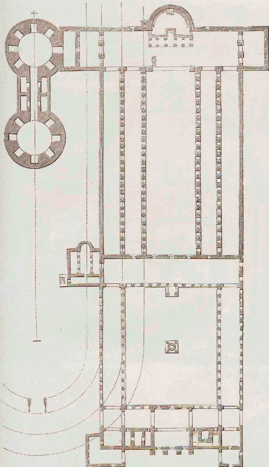
1. Plattegrond der oude Petruskerk te Rome. Geb. onder Constantijn den Grooten. De gestipte lijnen duiden de plaats van den vroegeren circus van Nero aan. (1 decem = 100 voet.)
