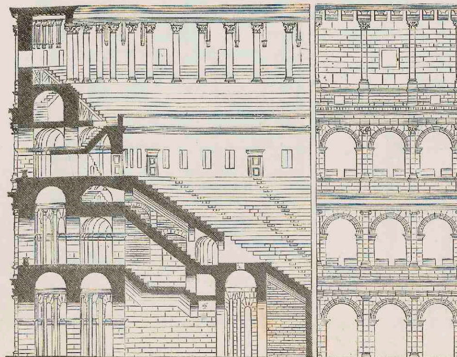
7. Colosseum: doorsnede en opstand. Begonnen onder Vespasianus, voltooid onder Titus, 80 v. Chr.
