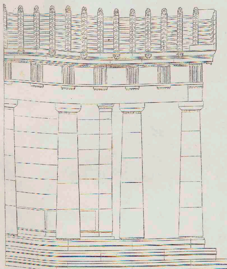
2. Tempel van Nemesis te Rhamnos. Gedeelte der zijde. (Vergelijk fig. 7 van plaat 8.)
