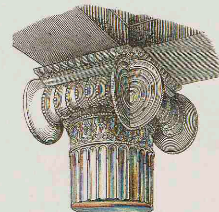
7. Binnenzijde van een ioniesch hoekkapiteel.
