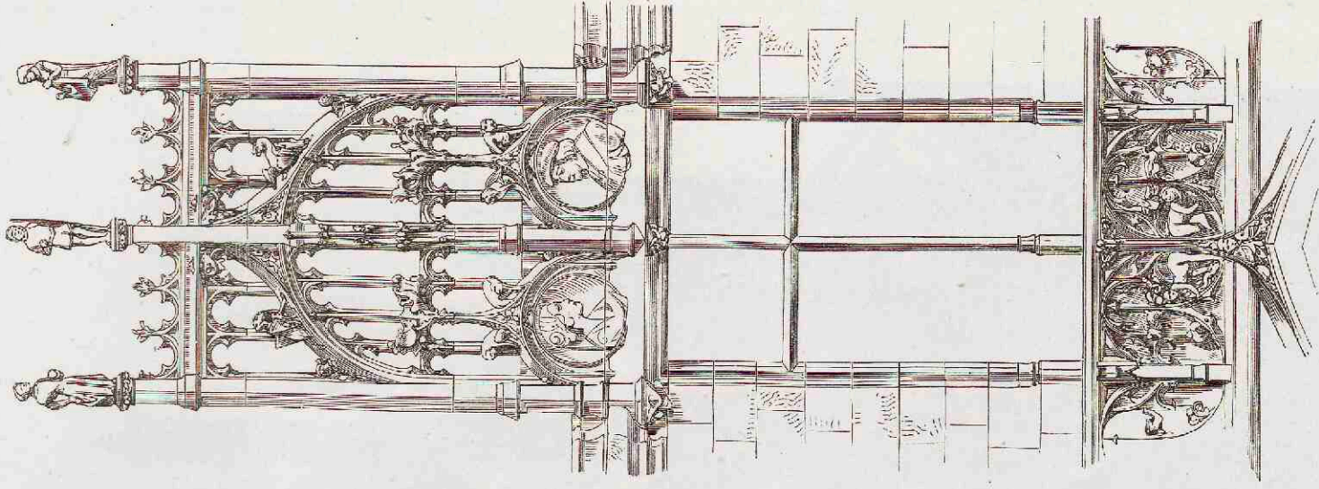
3. Venster van het hôtel de la Trémouille.
