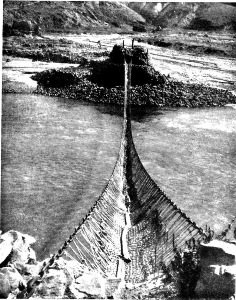
EEN KETTINGBRUG OVER DE TSANG-PO, TIBET.
