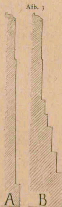
Doorsneden van absis en koortoren A over A-B, B over C-D van afb. 2
