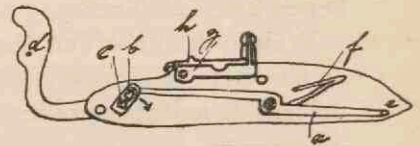
Lontslot
