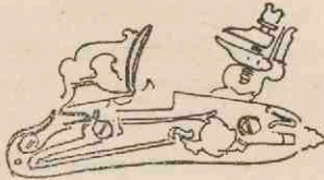
Snaphaanslot (binnenzijde)
