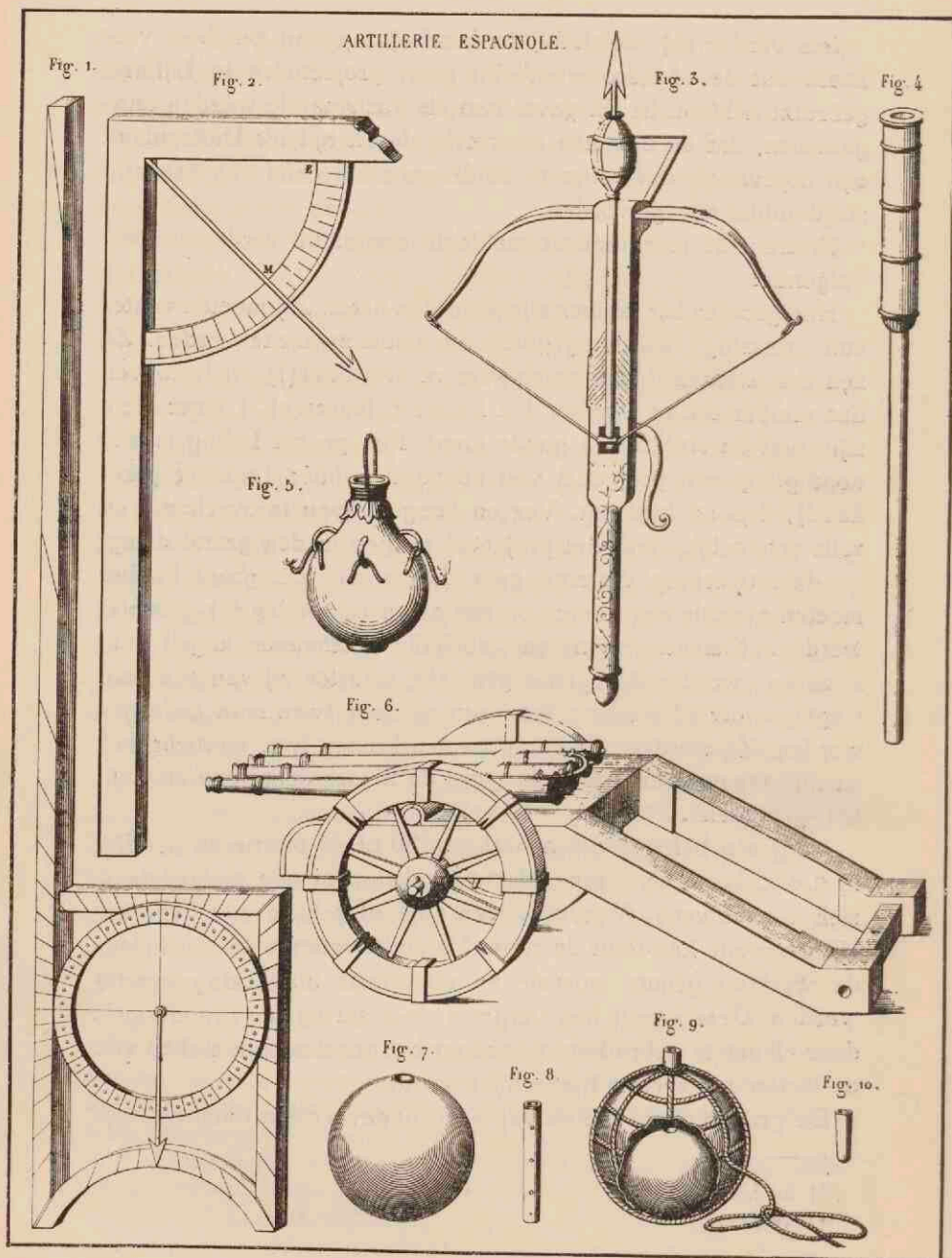
Uit: Ufano . 1, 2. quadranten (de lange arm wordt in den vuurmond gestoken); 3. voetboog met vuurpijl; 4. vuurkolf; 5. vuurpot; 6. orgelgeschut; 7, 8. bom met buis; 9, 10. brandkogel met granaat en buis.
