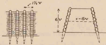
Bekleeding van rijshout.
