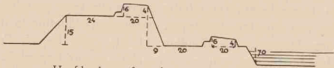
Hoofdwal met faussebraye volgens Marolais.
