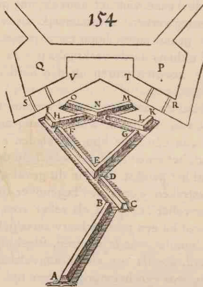
Algemeen beloop der approches volgens Marolais.
