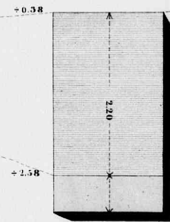
Boring N°28 bij Pilot 169. (Op den noordelyken oever van de Karsmeelkduid)
