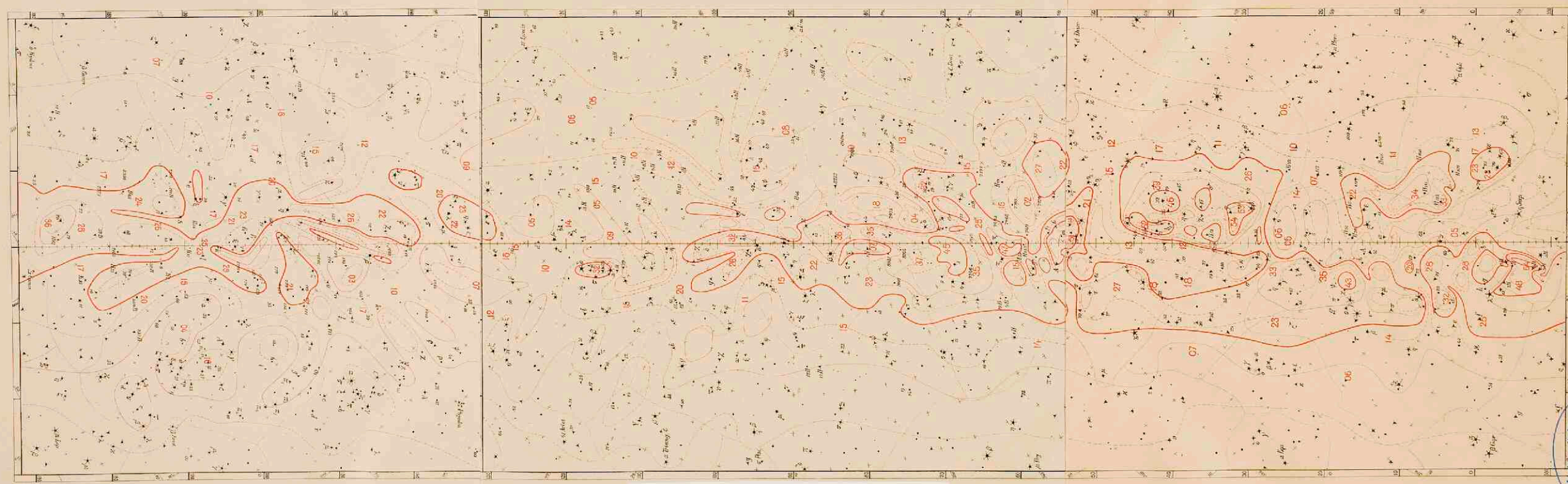
Isophoten van de Noordelijke Melkweg volgens Pannekoek
