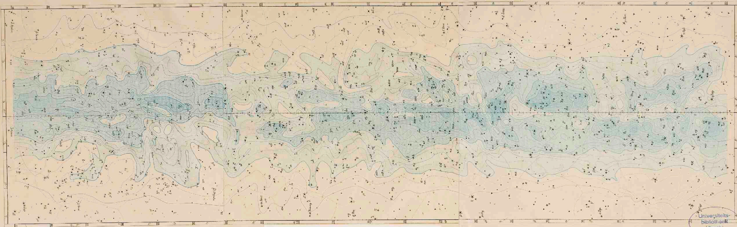
Gemiddelde isofoten van de Noordelijke Melkweg volgens Pannekoek, Schmidt e.a.
