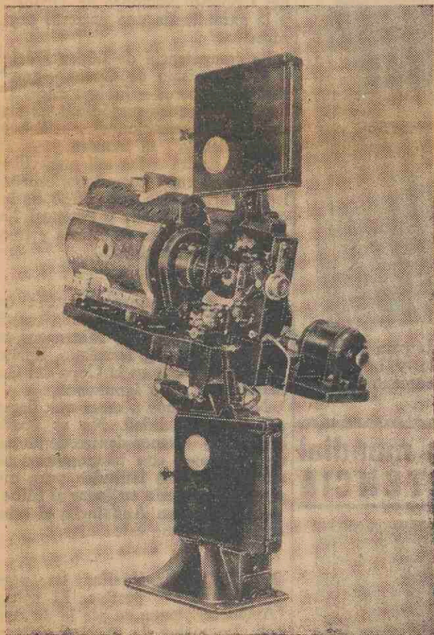
Una de las dos máquinas con linterna de alta intensidad y regulación automática de los carbones.
