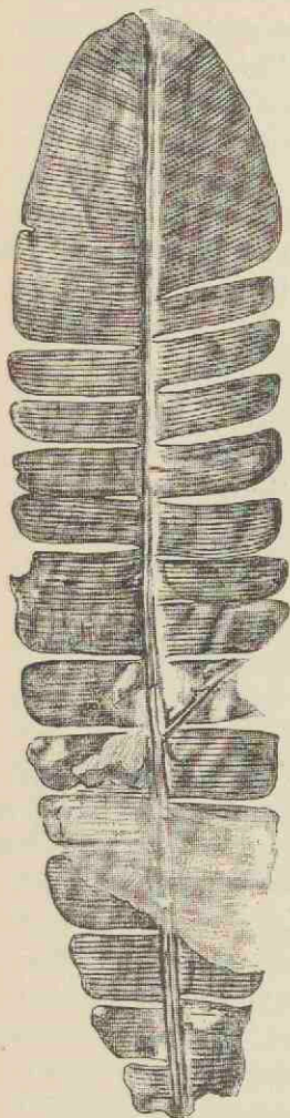
FIG. 615. Pterophyllum ( Anomozamites ) Nilssoni . (British Museum, 39,306; nat. size.)
