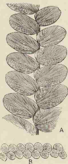
FIG. 606. A, Otozamites Beani . B, Otozamites Bunburyanus .
