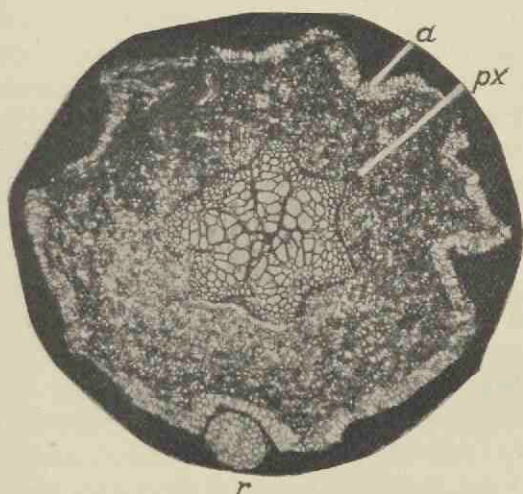
FIG. 410. Lyginopteris oldhamia , young root. \times 30 . (Kidston Coll. 403.)
