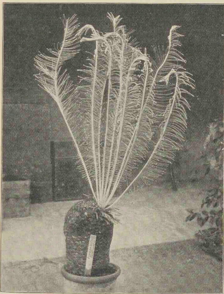
FIG. 382. Encephalartos Ghellinckii . ( \frac{1}{11} nat. size.)
