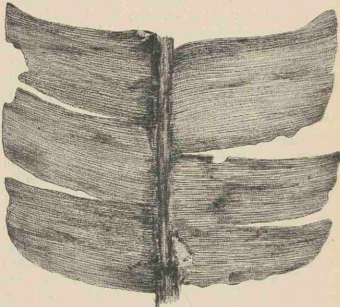
FIG. 622. Nilssonia compta . (Whitby Museum; nat. size.)
