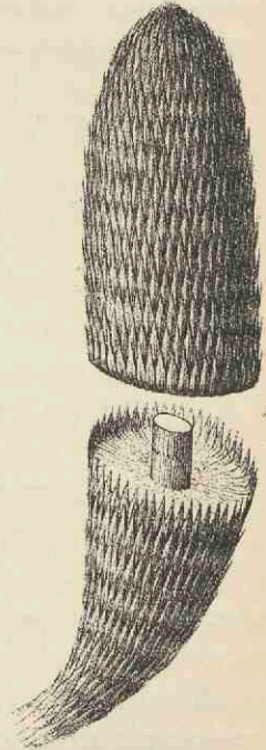
Fig. 118. — Macrostachya carinata Ger-mar (sp.), du Stéphanien. Epi de fructification, réduit aux \frac{3}{4} de grand. nat. (d'après Grand'Eury).
