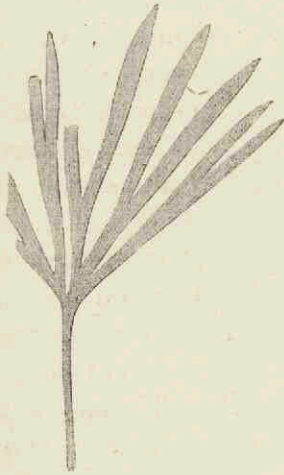
Fig. 180. — Baiera gracilis Bunbury, du Jurassique d'Angleterre. Feuille réduite aux \frac{2}{3} de grand. nat. (d'après Saporta).
