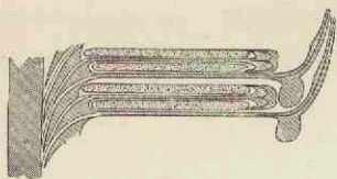
Fig. 120. — Cheirostrobos petty-curensis Scott, du Culm d'Angleterre. Coupe longitudinale schématisée d'un épi de fructification, grossie 2 fois (d'après Scott).
