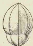
Fig. 150. — Codonospermum anomalum Brongniart, du Stéphanien. Graine, de grand. nat.
