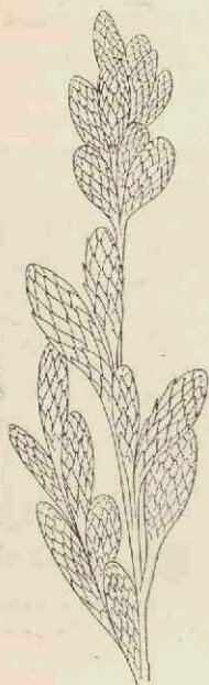
Fig. 201. — Rhizocaulon polystachyum Saporta, de l'Oligocène inférieur de Provence. Inflorescence, grand. nat. (d'après Saporta).
