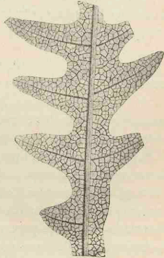
Fig. 91. — Dictyophyllum Nilssoni Brongniart (sp.), du Rhétien. Portion de penne, réduite aux \frac{3}{4} de grand. nat. (d'après Nathorst).
