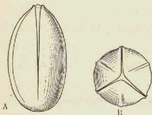
Fig. 149. — Trigonocarpus Næggerathi , Sternberg (sp.), du Westphalien. Graine réduite aux \frac{3}{4} de grand. nat. : A, vue de côté; B, vue en dessus.
