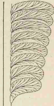
Fig. 84. — Nevropteridium imbricatum Schimper et Mougeot (sp.), du Trias inférieur. Base d'une fronde, légèrement grossie (d'après Schimper et Mougeot).
