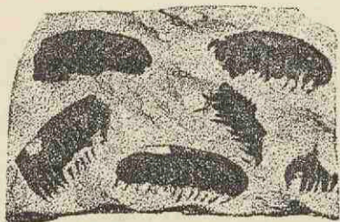
Fig. 83. — Linopteris Germari Giebel (sp.), du Stéphanien. Pinnules fertiles, grand. nat.
