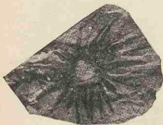
Fig. 115. — Phyllotheca Rallii Zeiller, du Westphalien d'Asie Mineure. Gaine foliaire appartenant à un rameau, grand. nat.
