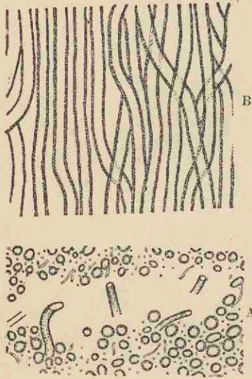
Fig. 7. — Nematophycus Loganii Dawson (sp.), du Silurien et du Dévonien inférieur du Canada. Coupes transversale (A) et longitudinale (B), grossies (d'après Dawson).
