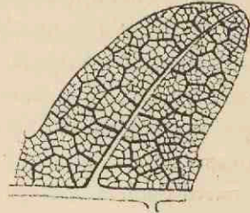
Fig. 20. — Dietyoptéridée. Fragment de penne, grossi (d'après Schenk).
