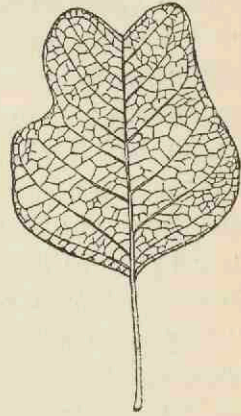
Fig. 208. — Liriodendron Meekei Heer, du Crétacé du Groënland. Feuille réduite à 1/2 grand. nat. (d'après Saporta et Marion).
