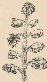
Fig. 31. — Crossothecca Crepinii Zeiller, du Westphalien. Portion de penne fertile, grossie 2 fois et demie.
