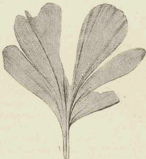
Fig. 178. — Psygmyphyllum expansum Brongniart (sp.), du Permien de Russie. Feuille réduite aux 2/3 de grand. nat. (d'après Schmalhausen).
