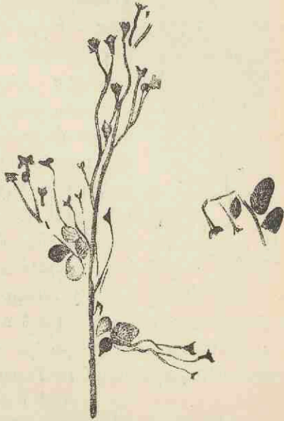
Fig. 81. — Nevrpt. heterophylla Brongniart. Fragments de pennes fertiles; grand. nat. (d'après Kidston).
