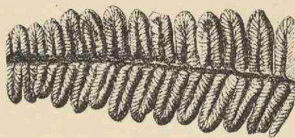
Fig. 16. — Pécoptéridée. Fragment de penne, grand. nat. (d'après Stur).
