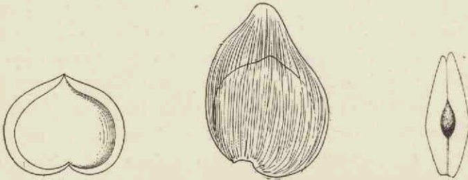
Fig. 146. — Cardiocarpus reniformis Geinitz, du Permien. Graine, réduite aux \frac{2}{3} de grand. nat.
