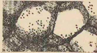
Fig. 12. — Micrococcus Guignardi Renault du Stéphanien de Saint-Etienne. Tissu cellulaire envahi par les Microcoques : très fortement grossi (d'après Renault).
