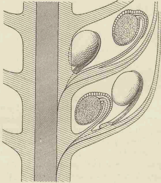
Fig. 103. — Coupe longitudinale schématique d'un épi de Sphenoph. cuneifolium , grossie 12 fois.
