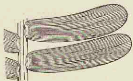
Fig. 155. — Glossozamites Zittel Schenk (sp.), de l'Urgonien des Carpathes. Fragment de fronde, réduit aux 3/5 de grand. nat. (d'après Schenk).
