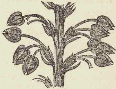
Fig. 144. — Samaropsis Pitcairnia Lindley et Hutton (sp.), du Westphalien. Fragment d'inflorescence, grand. nat. (d'après Carruthers).
