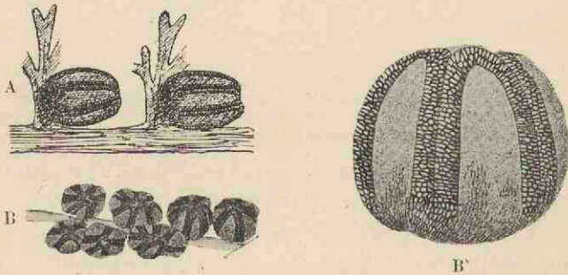
Fig. 46. — A, Corynepteris Essinghi Andræ (sp.), du Westphalien. Fragment de penne fertile, grossi 6 fois. — B, Coryn. coralloides Gutbier (sp.), du Westphalien. Fragment de penne fertile, grossi 4 fois. B', sore de la même espèce, vu de côté, grossi 28 fois.
