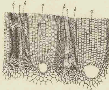
Fig. 109. — Calamodendron striatum Gotta (sp.), du Permien d'Autun. Coupe transversale, grossie, montrant deux coins ligneux : a , bois secondaire formé de trachéides rayées; b , bandes prosenchymateuses; c , rayons médullaires primaires (d'après Renault).
