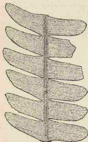
Fig. 165. — Pterozamites Müns-terii Presl (sp.), du Rhétien. Fragment de fronde, grand. nat.
