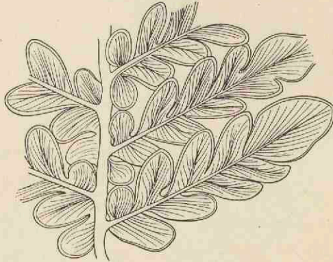
Fig. 66. — Lomatopteris ambigua Saporta, du Kimmérien. Fragment de fronde, grand. natur. (d'après Saporta).
