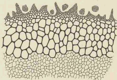
Fig 124 — Lepidod. Harcourtii Witham, du Houiller d'Angleterre. Coupe transversale montrant une partie de la moelle centrale et de l'anneau ligneux avec ses pointements trachéens et plusieurs faisceaux foliaires ; grossie 18 fois (d'après Williamson).
