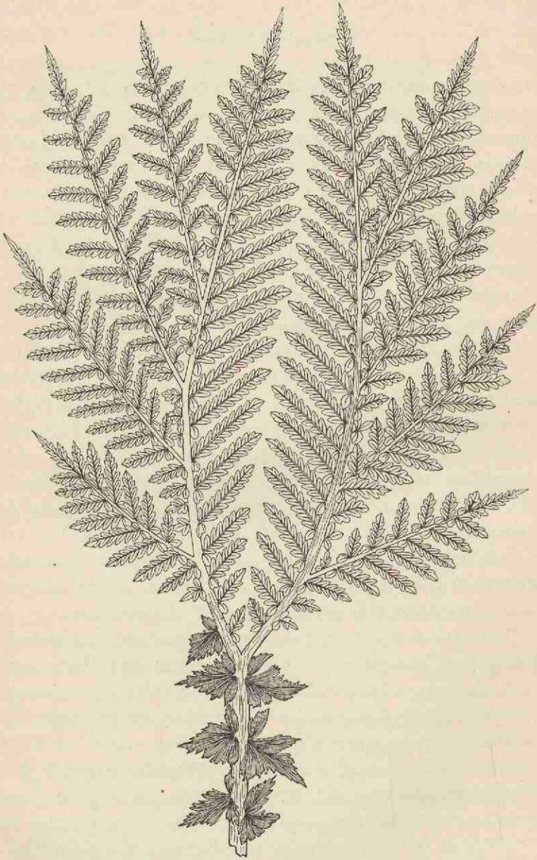
Fig. 53. — Odontopteris minor Brongniart, du Stéphanien. Portion de fronde, réduite à \frac{1}{3} de grandeur naturelle (d'après des échantillons des mines de Blanzy).
