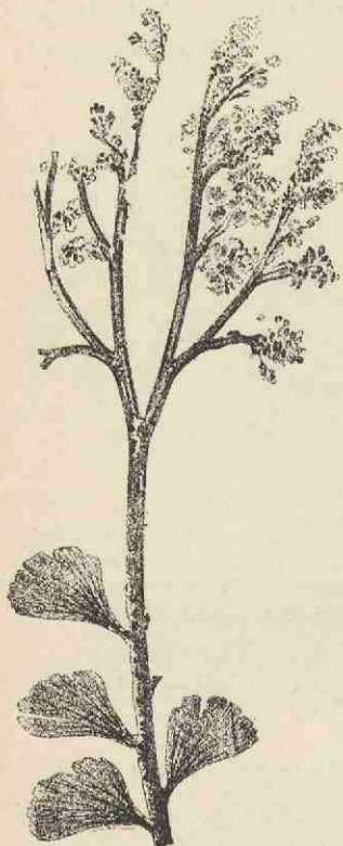
Fig. 78. — Rhacopteris paniculifera Stur, du Culm. Partie supérieure d'une fronde fertile, réduite aux \frac{2}{3} de grand. nat. (d'après Stur).
