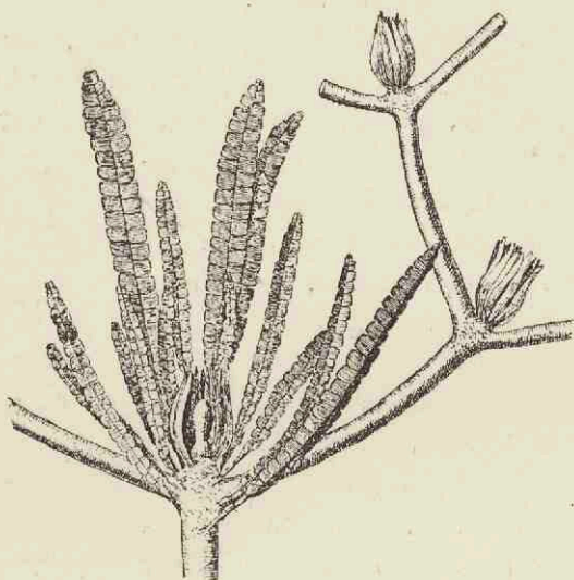
Fig. 167. — Anomozamites minor Brongniart (sp.), du Rhétien. Échantillon fructifié, partiellement restauré, réduit à \frac{1}{3} de grand. nat. (d'après Nathorst).
