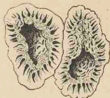
Fig. 9. — Reinschia australis Bertrand et Renault, du Kerosene Shale de la Nouvelle-Galles du Sud. Section horizontale de jeunes thalles; gross. 540 diam. (d'après C. E. Bertrand).
