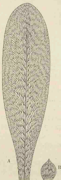
Fig. 86. — Glossopteris Browniana Brongniart, du Permotrias du Transvaal. A, fronde normale; B, fronde écailleuse; grand. nat.
