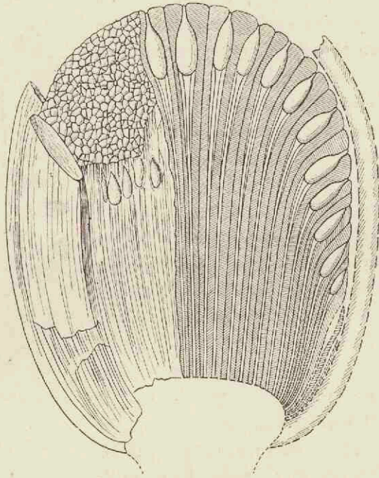
Fig. 172. — Bennettites Morierei Saprota et Marion (sp.), de l'Oxfordien. Appareil fructificateur, vu, partie extérieurement, partie en coupe longitudinale, grossi environ une fois et demie (d'après Saprota et Lignier).
