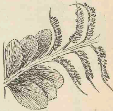
Fig. 77. — Archæopteris hibernica Forbes (sp.), du Dévonien supérieur. Portion de penne, stérile à la base, puis fertile; grand. nat. (d'après Schimper).
