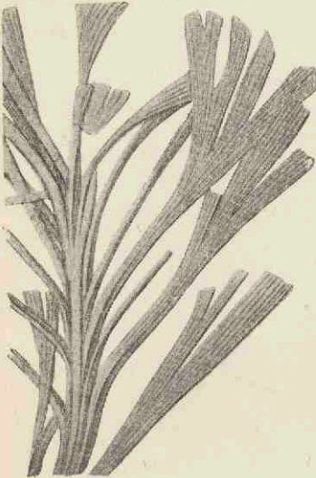
Fig. 179. — Ginkgophyllum Grasselti Saporta, du Permien de Lodève. Fragment de rameau feuillé, réduit aux \frac{2}{3} de grand. nat. (d'après Saporta).
