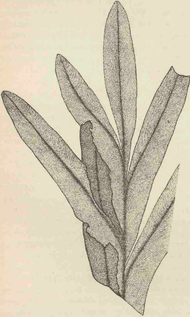
Fig. 85. — Megalopteris Hartii Andrews, du Calm de l'Ohio. Fragment de fronde réduit aux 9/10 de grand. nat. (d'après Andrews).
