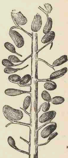
Fig. 171. — Zamiostrobus stenorrhachis Nathorst, du Rhétien de Suède. Inflorescence femelle, grand. nat. (d'après Saporta et Marion).
