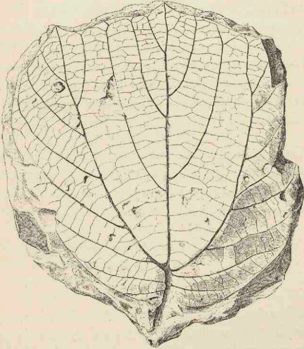
Fig. 207. — Credneria triacuminata Hampe, du Cénomaniens de Blankenburg. Feuille réduite aux \frac{2}{3} de grand. nat. (d'après Schimper).
