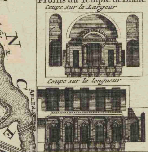
Profils du Temple de Diane coupe sur la largeur et coupe sur la longueur
