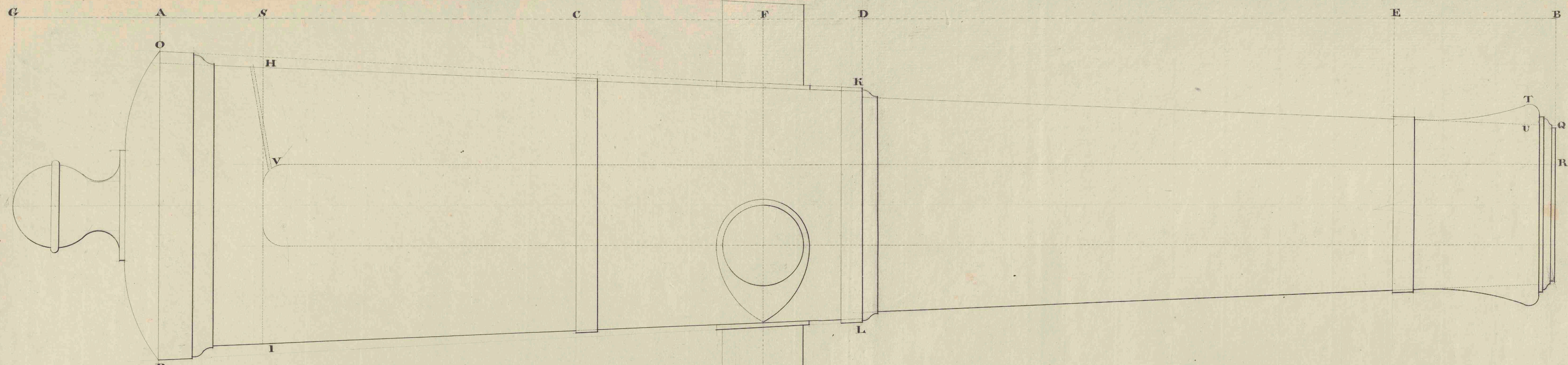
Yzer Kanon à 36 l. het 1/2 Deel van zijn Effectieve Groute
