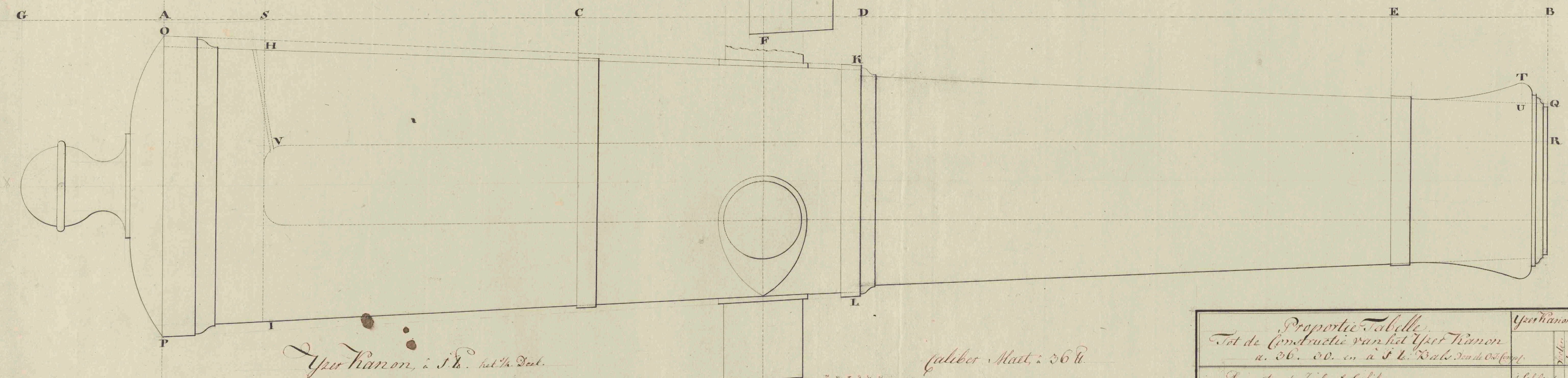
Yzer Kanon, à 30 l. het 1/2 Deel van zijn Effectieve Groute
