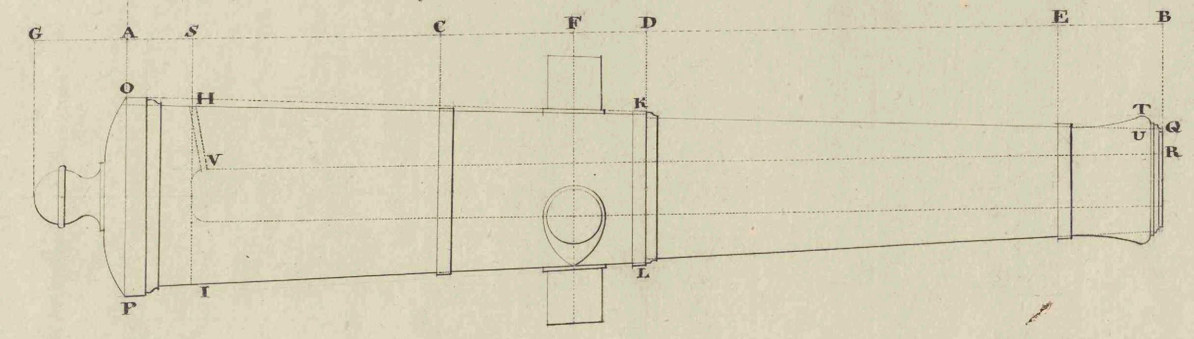
Yzer Kanon, à 18 l. het 1/2 Deel.
