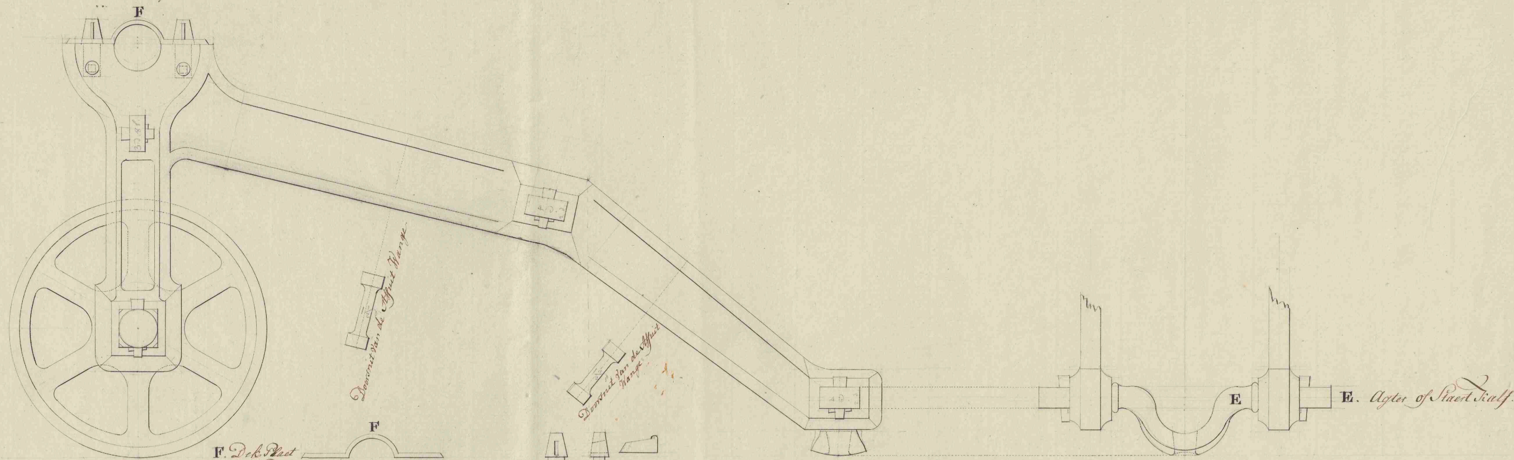
F. Deel van de Affuit Wange van ter zijden.
