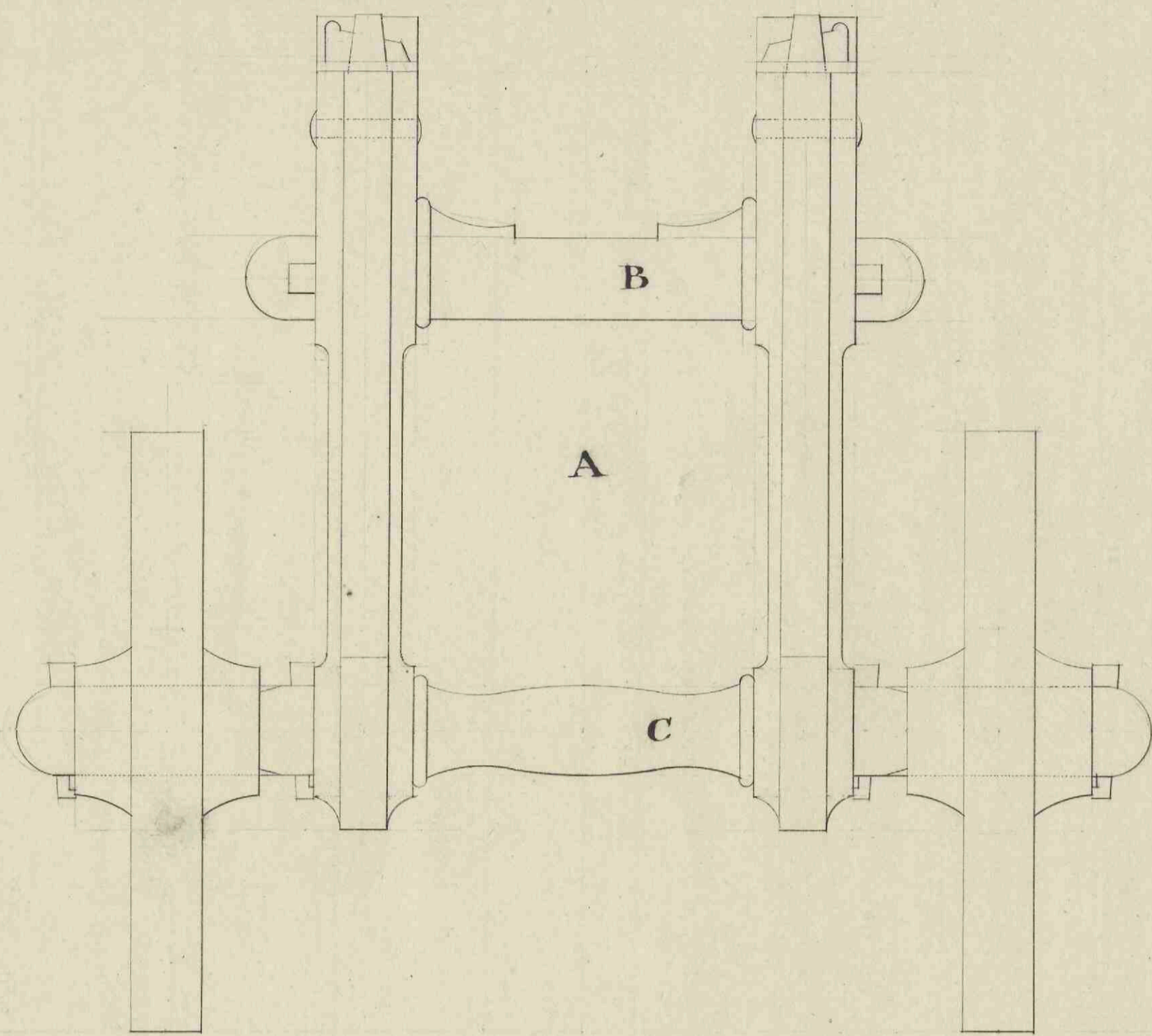
A. Affuit, van Vooren te zien
