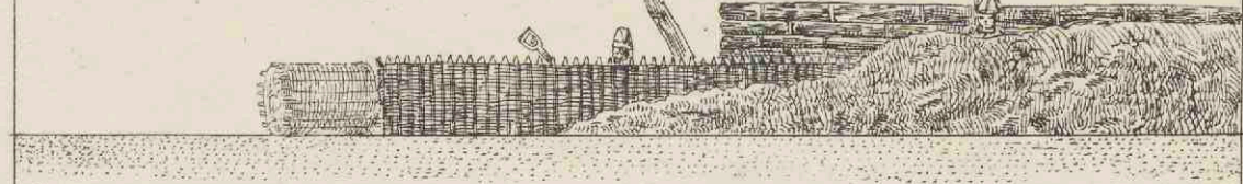
Doorsnede der voltoorde Loopgraaf
