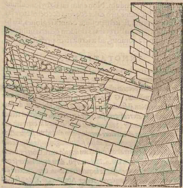
Fundamēti pectinatim facti, ueluti serræ dentes esse solent.
