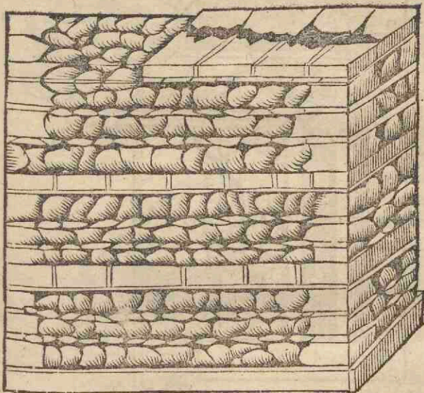
Antiquæ structuræ imbricatæ/ figura, quæ in cer- ti muri di- citur.
