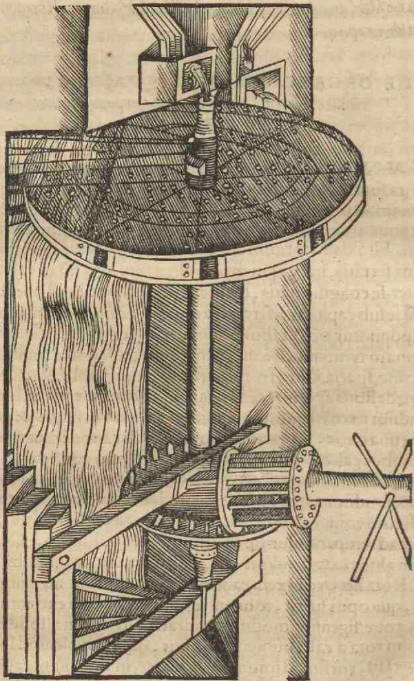
Organum tympani- cum ad a- quam hau- riendam.
