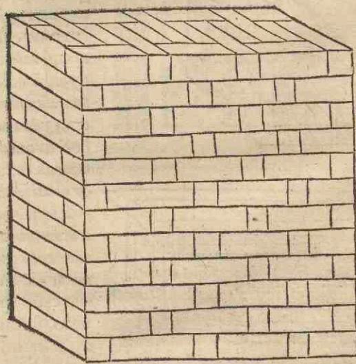
Isodomi structura.
