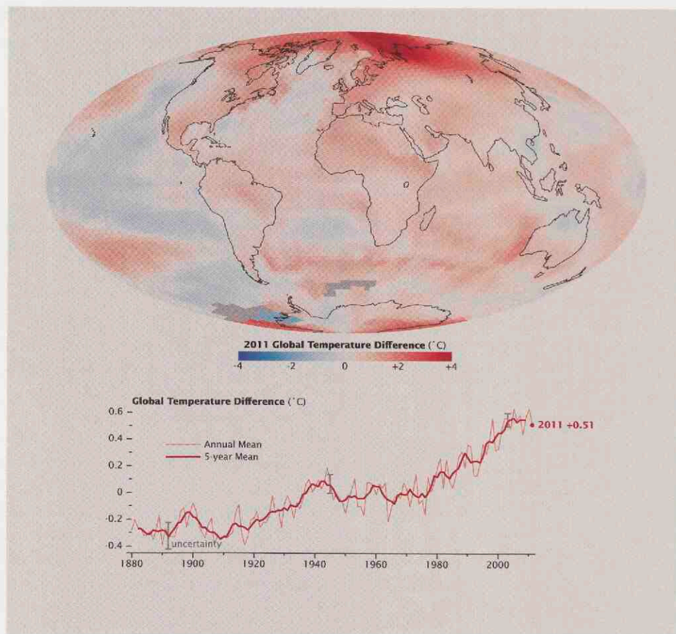
Temperatuurontwikkeling sinds 1880
