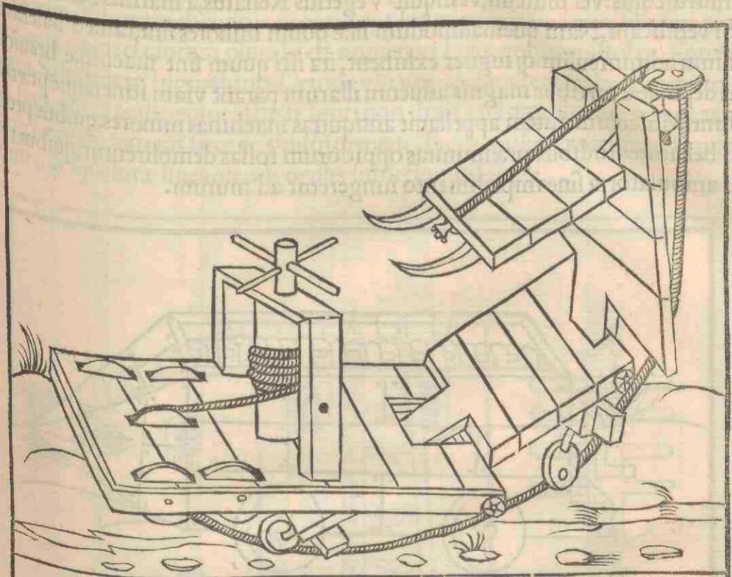
Producendi pontis instrumentum.
