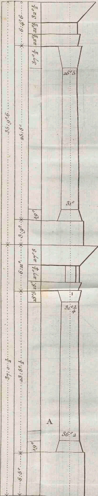
ORDRES Dorique et Corinthien du Portail de St Roch.
