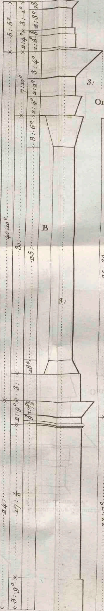
ORDRE Corinthien des Bâtimens de la Place de Louis XV.
