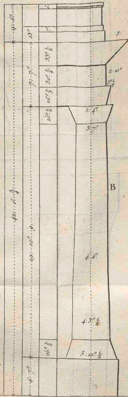
ORDRE Toscan de l'Orangerie de Versailles.
