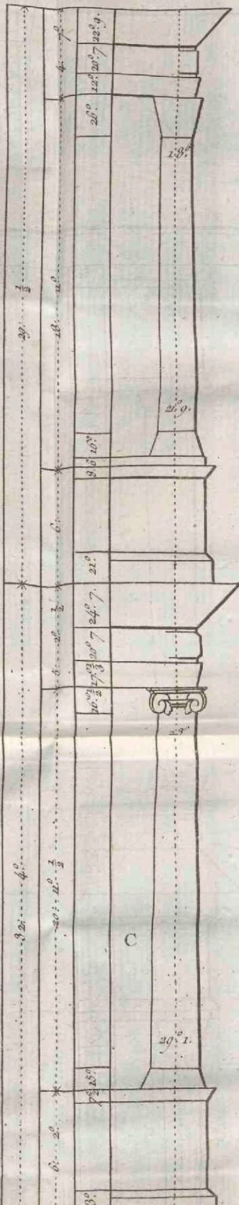
ORDRES Ionique et Corinthien du Portail des Feuillans du Cote de la Cour.
