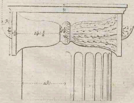
CHAPITEAU VU SUR LE COTE.
