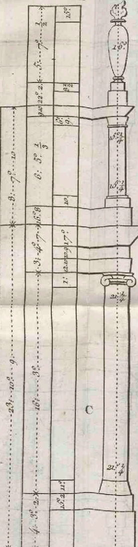
ORDRE Jonique de l'ancien Hotel de Jars avec son Attique.
