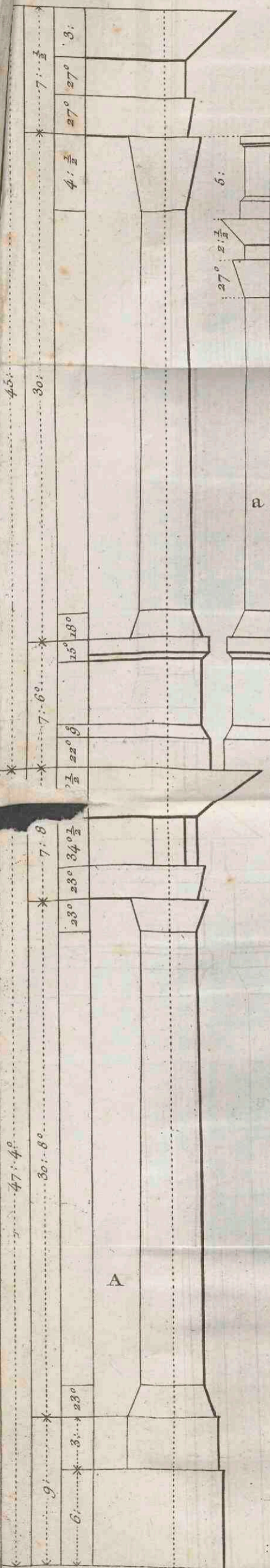
ORDRES Dorique et Corinthien du Portail des Invalides.
