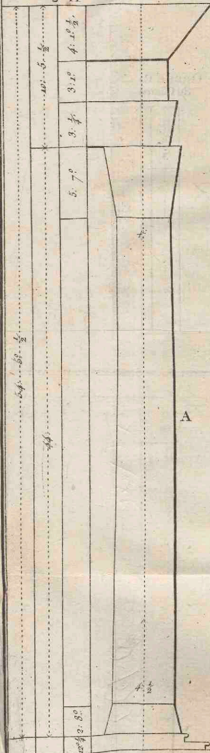
ORDRE Corinthien du Portique d'Agrippa au Pantheon.
