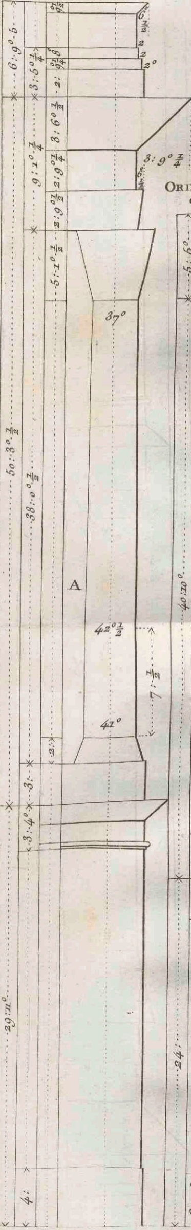
ORDRE Corinthien du Peristyle du Louvre.
