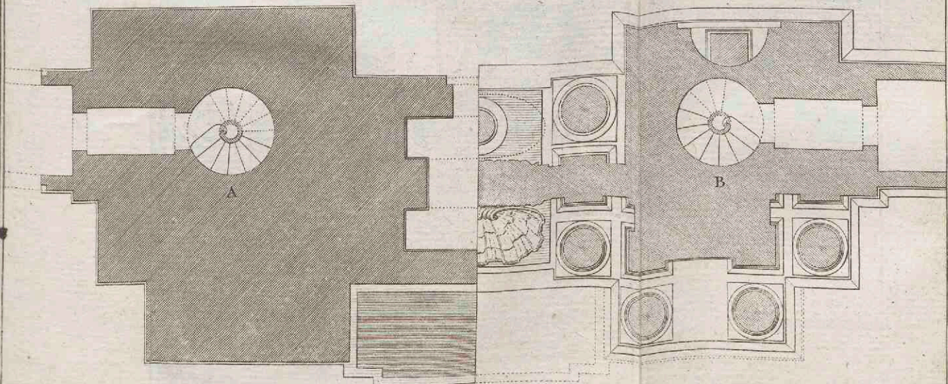
PLANS DÉVELOPÉS D'UNE FONTAINE PUBLIQUE.
