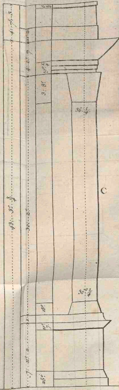
ORDRE Corinthien de l'Exterieur du Chateau de Montmorancy.
