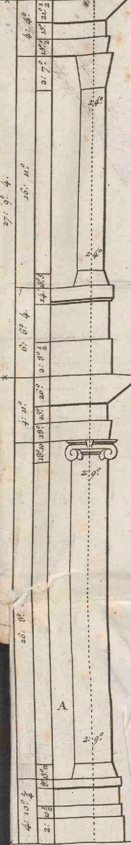
ORDRE Ionique du Portail de St. Nicolas du Chardonnet avec son Attique.
