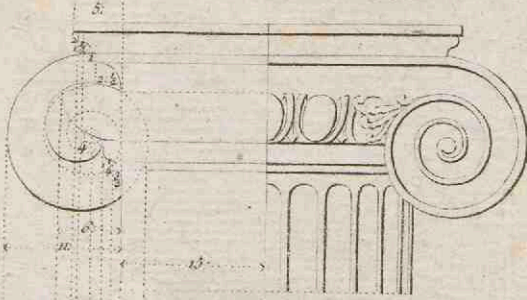
CHAPITEAU VU DE FACE.
