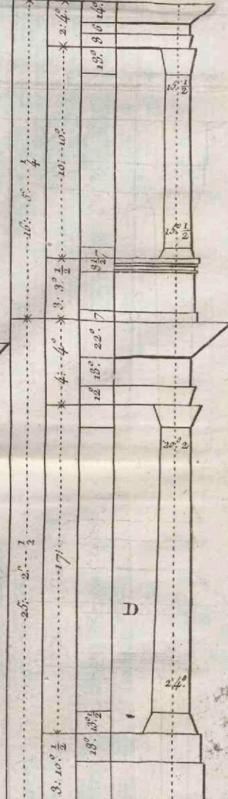
ORDRE Dorique de la Porte de l'Hotel du grand Prieur de France du Cote de la rue du Temple avec son Attique.
