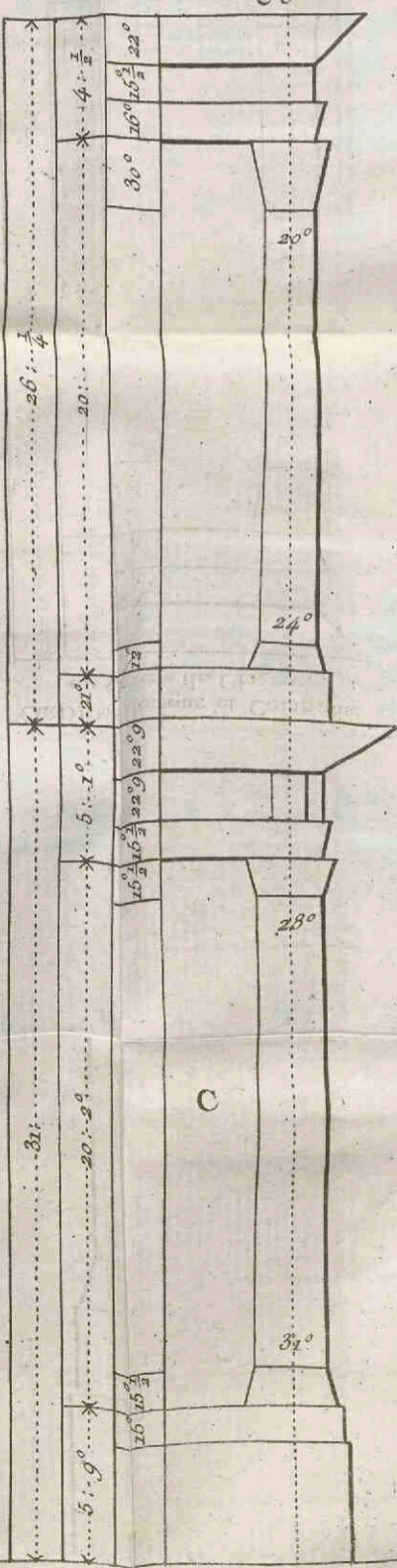
ORDRES Dorique et Composite du Château de Clagny.
