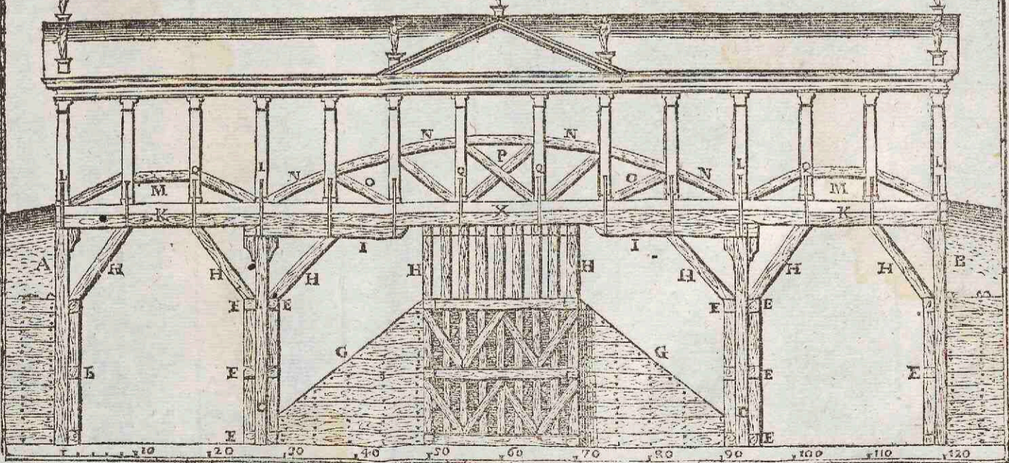
PONTE ARTIFICIOSIS. DE LEGAMI ARMATI COPERTO, Vint. Scam. Arch.
