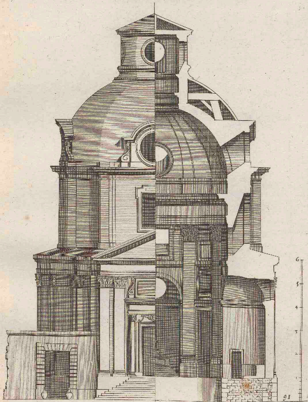
Elevation et Coupe d'une Eglise Composée par Jean Marot Architecte.
