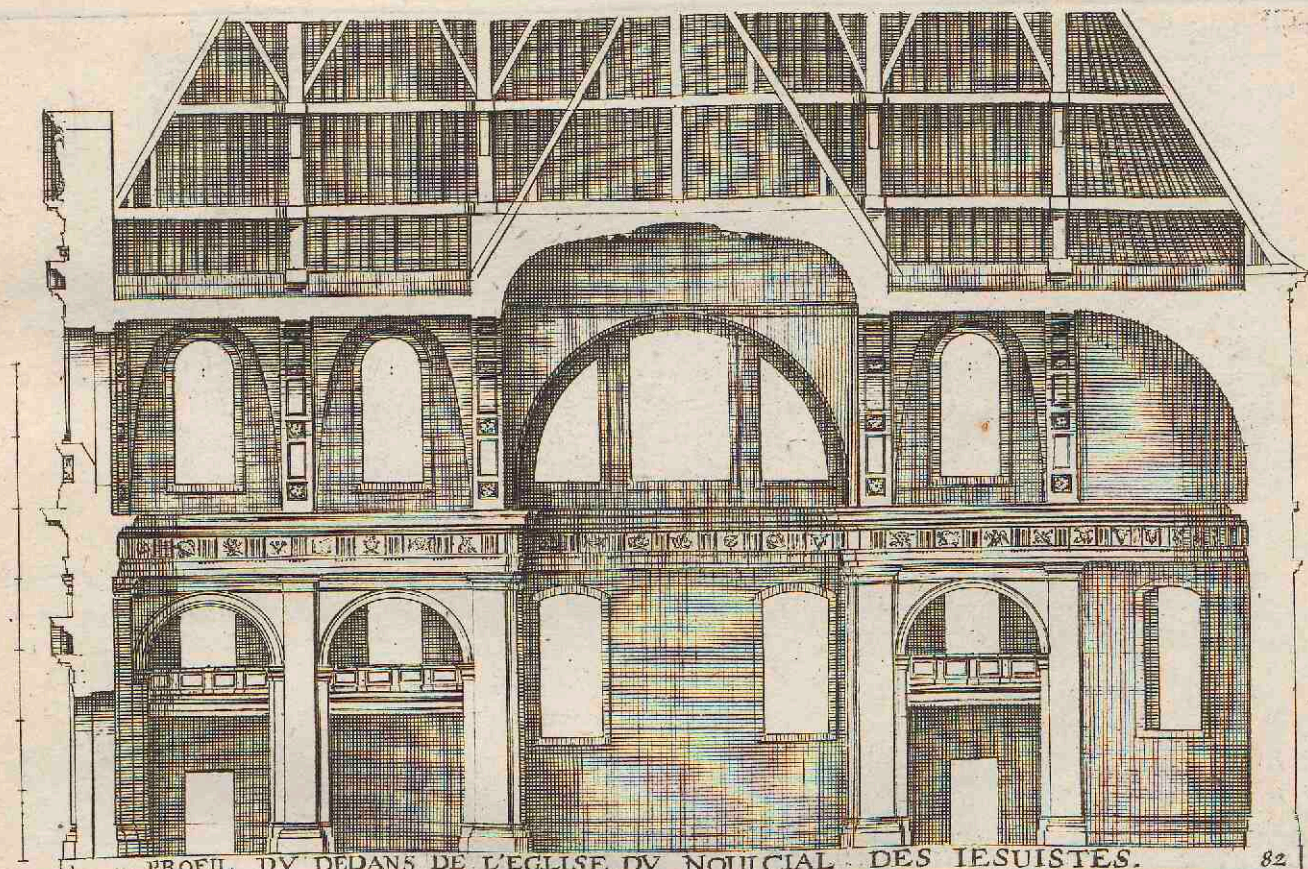
PROFIL DV DEDANS DE L'EGLISE DV NOUCIAL DES IESUISTES.
