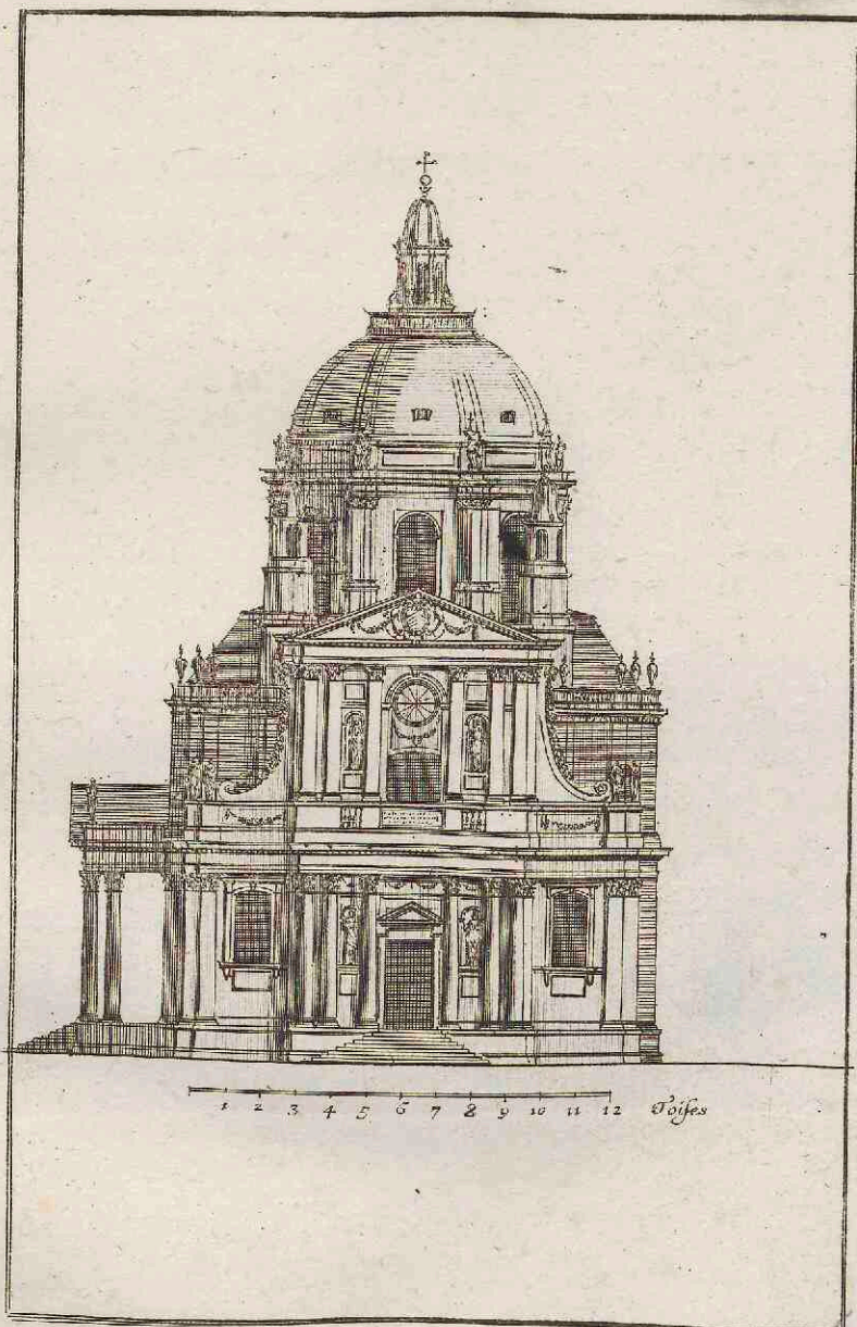
Le grand portail de l'Eglise de la Sorbonne du costé de la rue.
