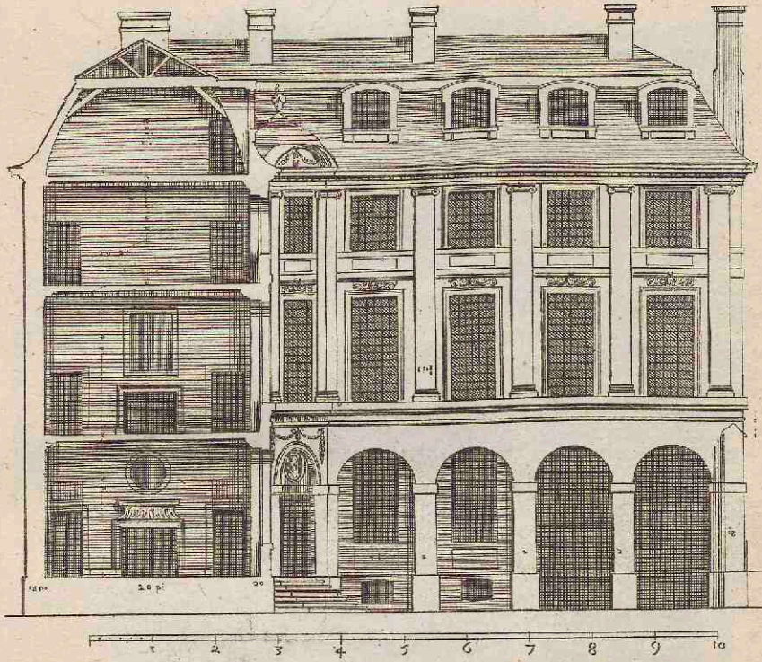
Profil du dedans de la Cour de la Maison de Monsieur Roland A Paris: Jean Marot fecit.
