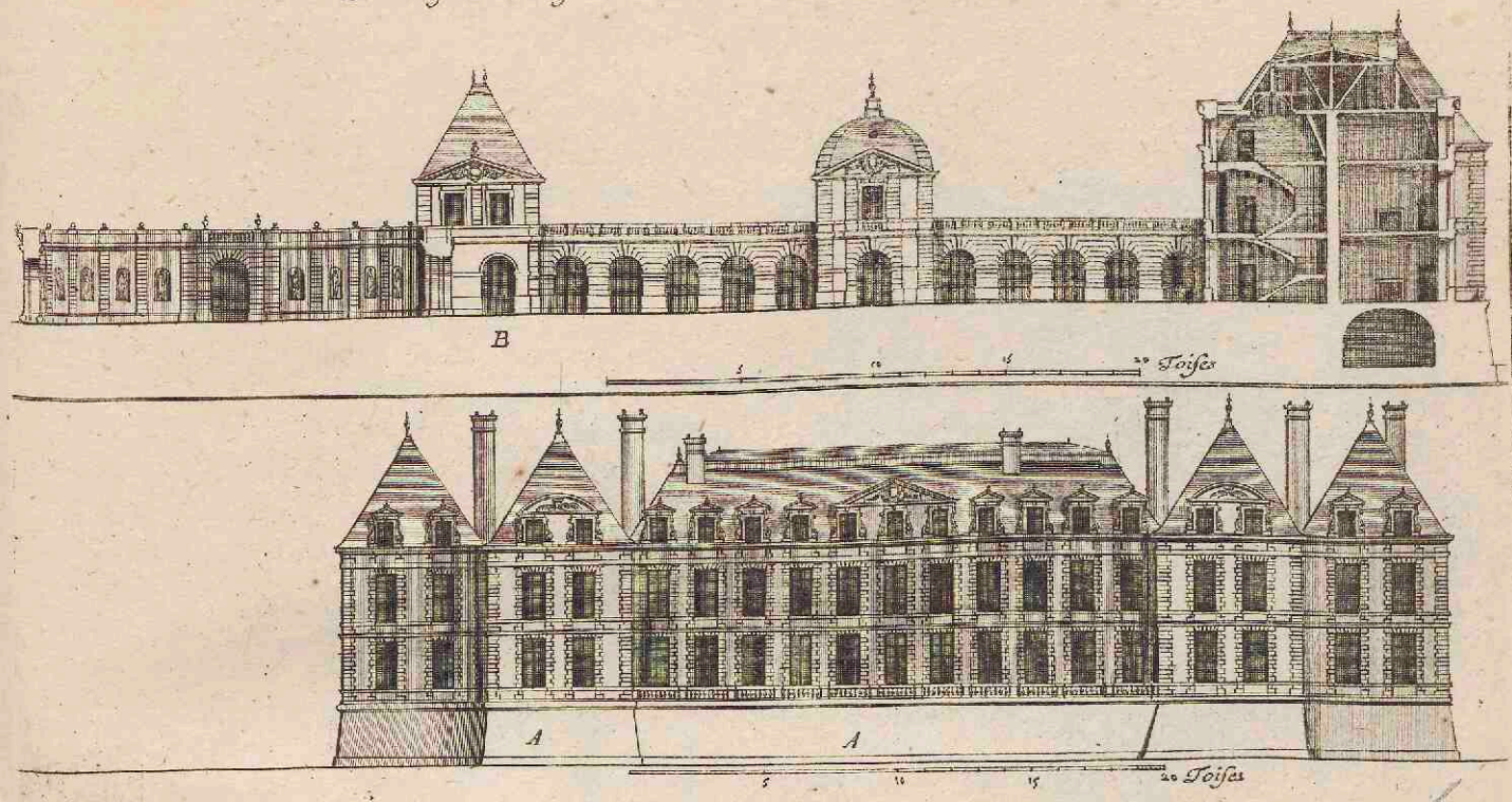
A. Elevation du derriere du Chateau de Tours B. Profil du Chateau de Tours
