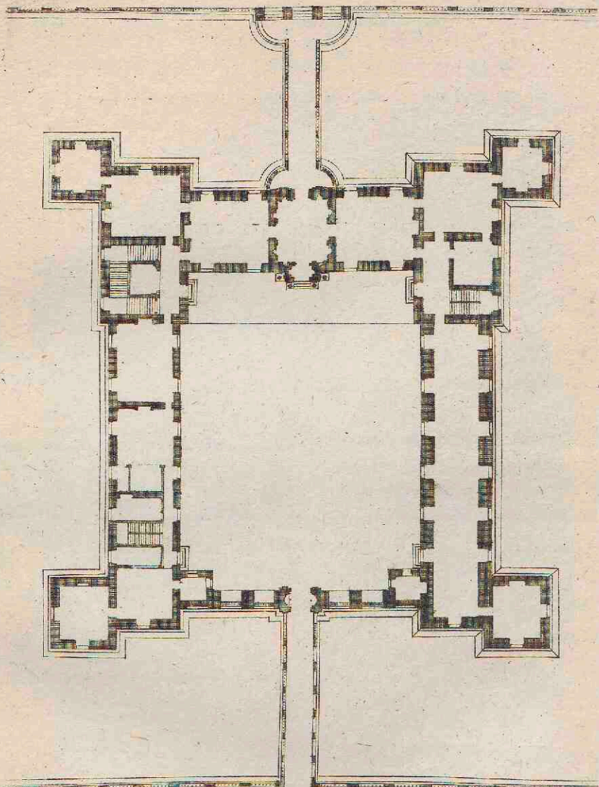
Plan du premier étage du rez de chaussée de la cour du Château de Pontz en Champagne.
