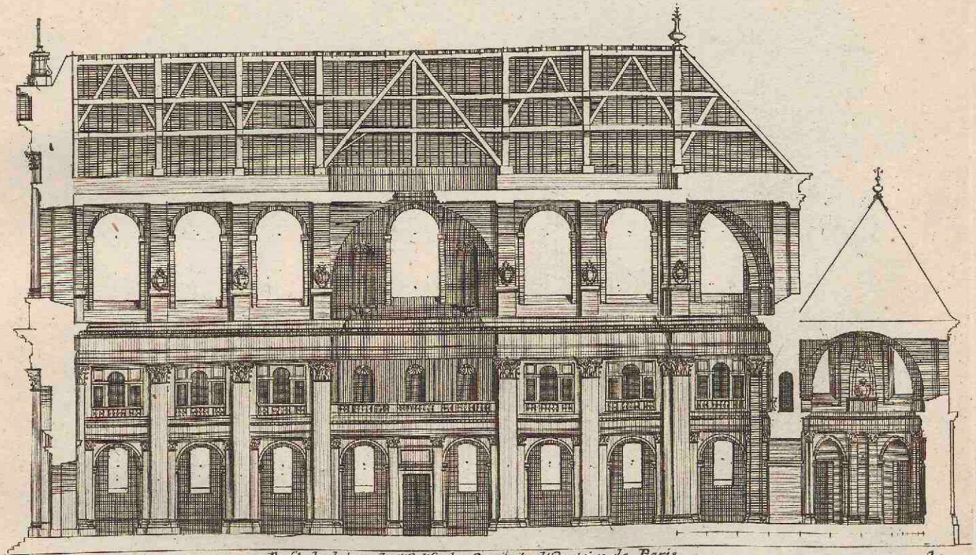
Profil du dedans de l'Eglise des Peres de l'Oratoire de Paris.
