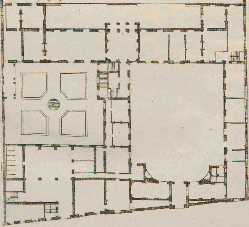
Plan du rez de chaussee de l'Hotel de Liancourt Au fauxbourg S t . Germain à la rue de Seine bâti par Jacques le Mercier .
