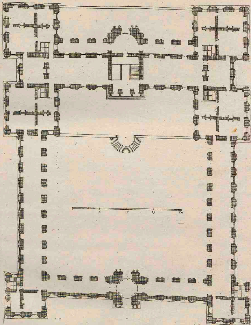
Plan du Palais d'Orléans a Paris. du Dessin de Salomon de Brosse.
