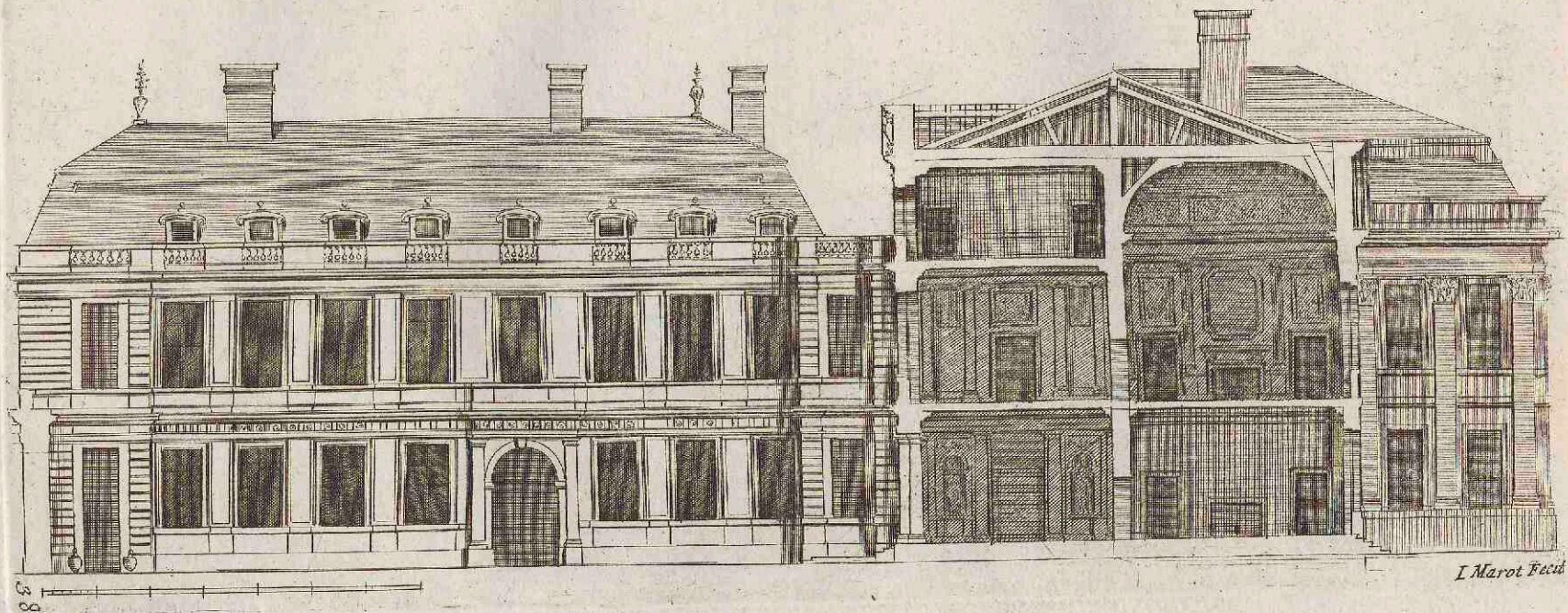
Profil du dedans de la Cour de l'Hostel de Lyonne, bastie A Paris.
