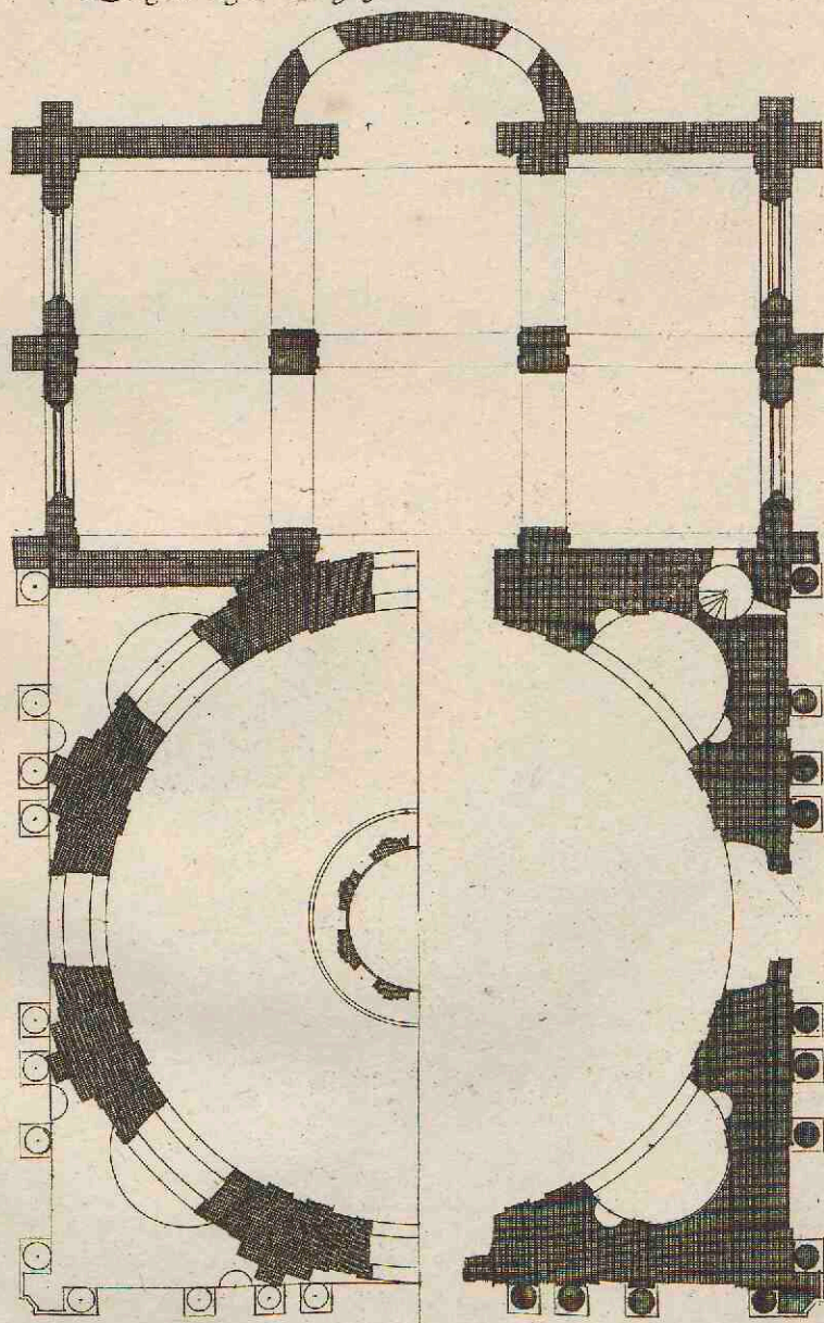
Le Plan de l'Eglise de nostre Dame des Artilieres les Saumur Que fait bastir Monseigneur le Comte de Seruien.
