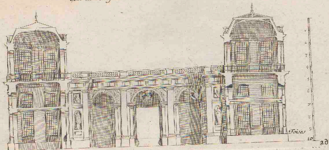
11 Elevation de la demy Lune du dedans de la Cour de l'Edifice de Mons r Jabba. Jean Marot fecit.
