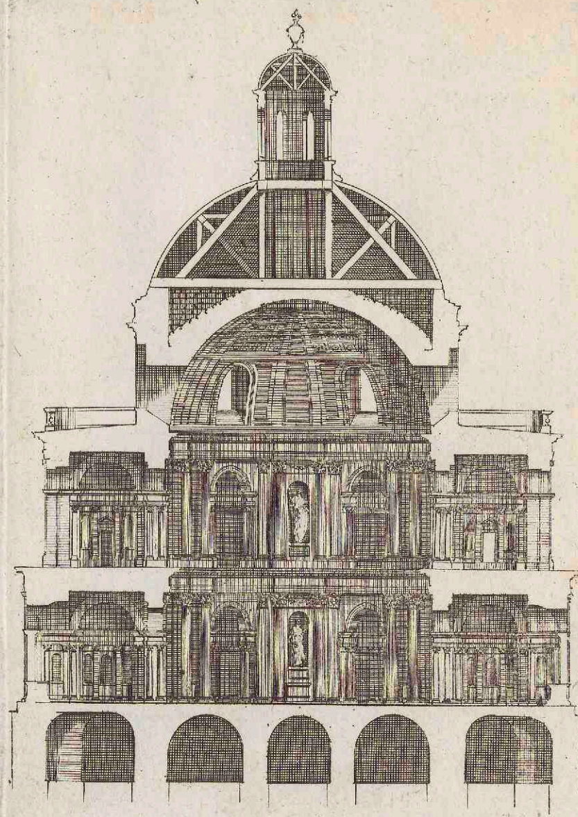
Profil du dedans de la sepulture des Rois des Valois à S t . Denis
