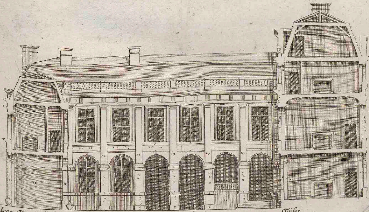
Profil de l'Hostel Tubeuf du costé de la court
