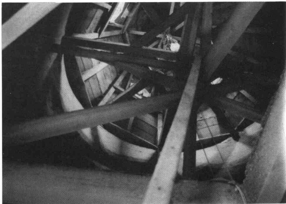
Het interieur naar boven gezien, met de opvallende, ingenieuze balkenconstructie.
