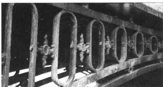
Detail smeedijzeren spanten met gietijzeren ornamenten van de grote brug
