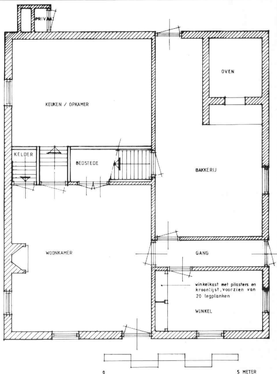
RECONSTRUCTIE WOONHUIS / BAKKERIJ - WINKEL
