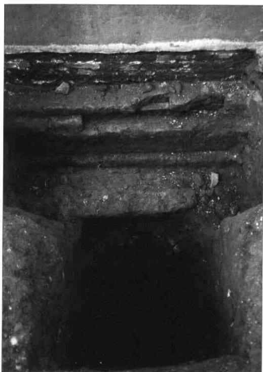
6. Het fundament van de zuidgevel (in 1832 gesloopt en op de bestaande fundering vanaf het maaiveld opnieuw opgetrokken) bestaat uit tufstenen platen, rustend op een laag veldkeien, zowel rond als hoekig. Als bindmiddel tussen de keien is klei gebruikt
