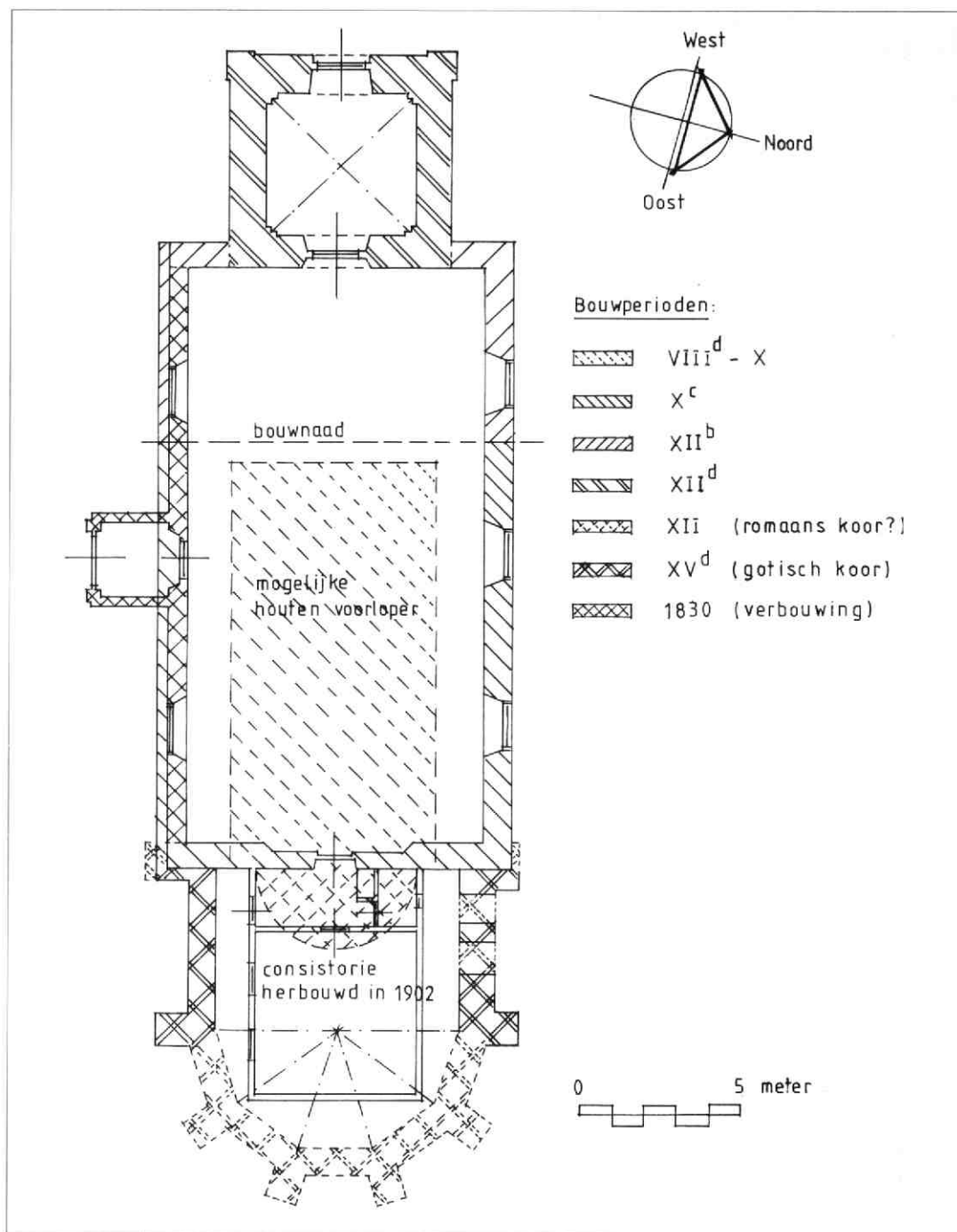
2. Plattegrond van de kerk met de datering van de bouwdeelen. Tevens is op deze plattegrond de mogelijke locatie van een eventuele (houten) voorganger van de huidige kerk en de veronderstelde plattegrond van een mogelijk romaans koor aangegeven.
