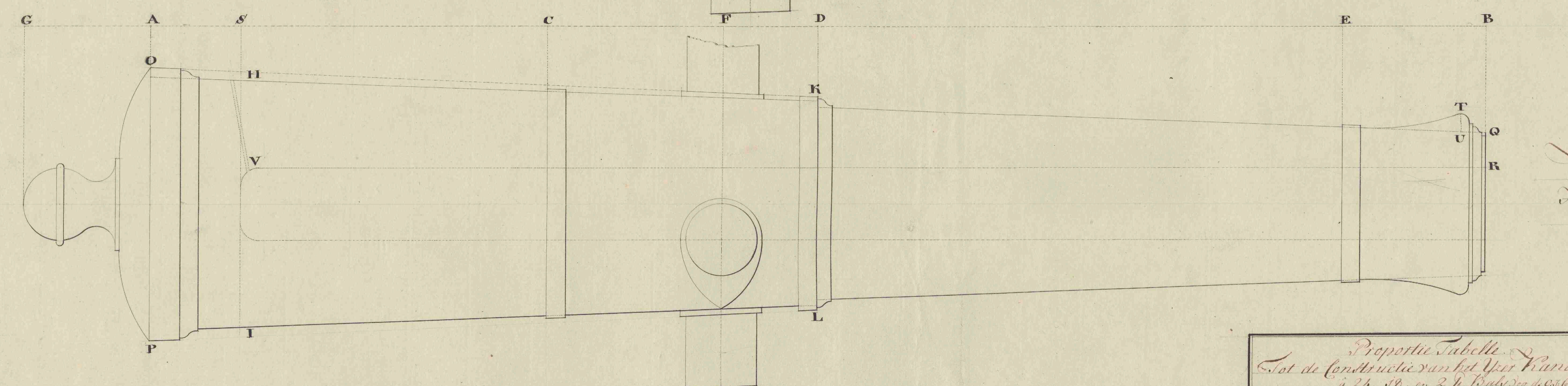
Yzer Kanon, à 36 lb. Het 1/4. Deel van zijn Effectieve Groote.
